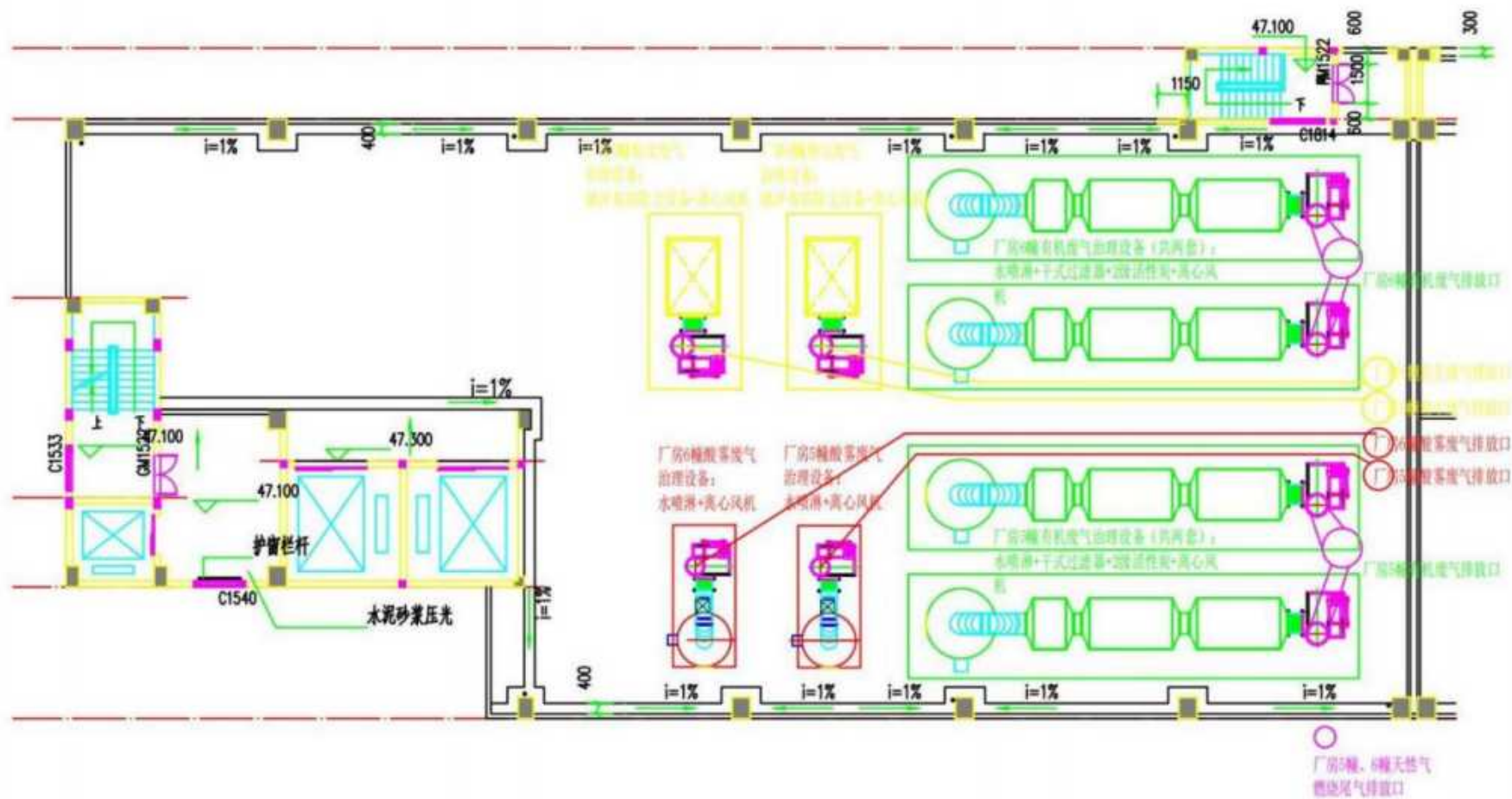
厂房5幢屋面平面图（废气设备示意图）
