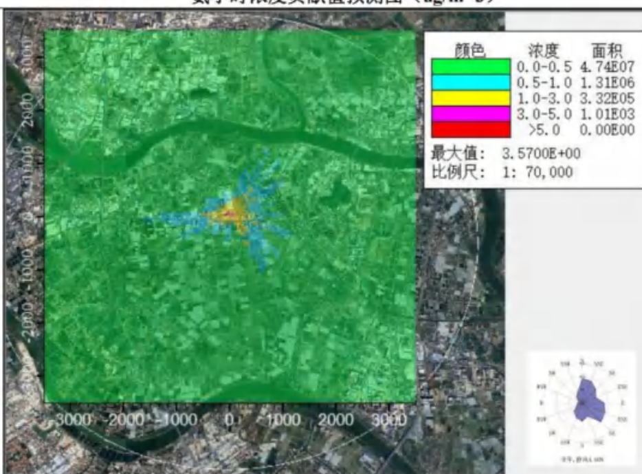
硫化氢小时浓度贡献值预测图 ( \mu\text{g}/\text{m}^3 )
