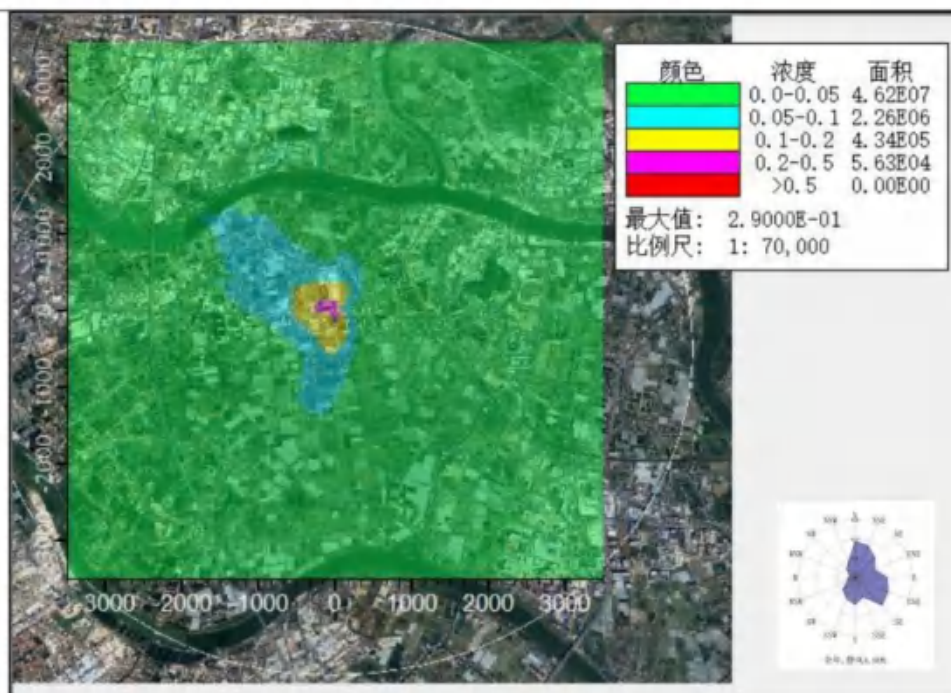
NO2 年均浓度贡献值预测图 ( \mu\text{g}/\text{m}^3 )
