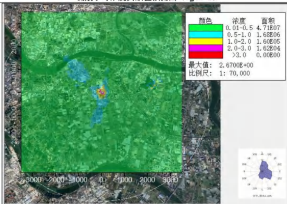
硫酸日均浓度贡献值预测图 (ug/m³)
