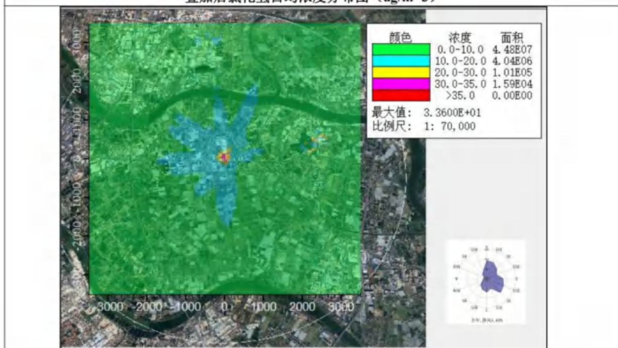
叠加后硫酸小时浓度分布图 ( \mu\text{g}/\text{m}^3 )
