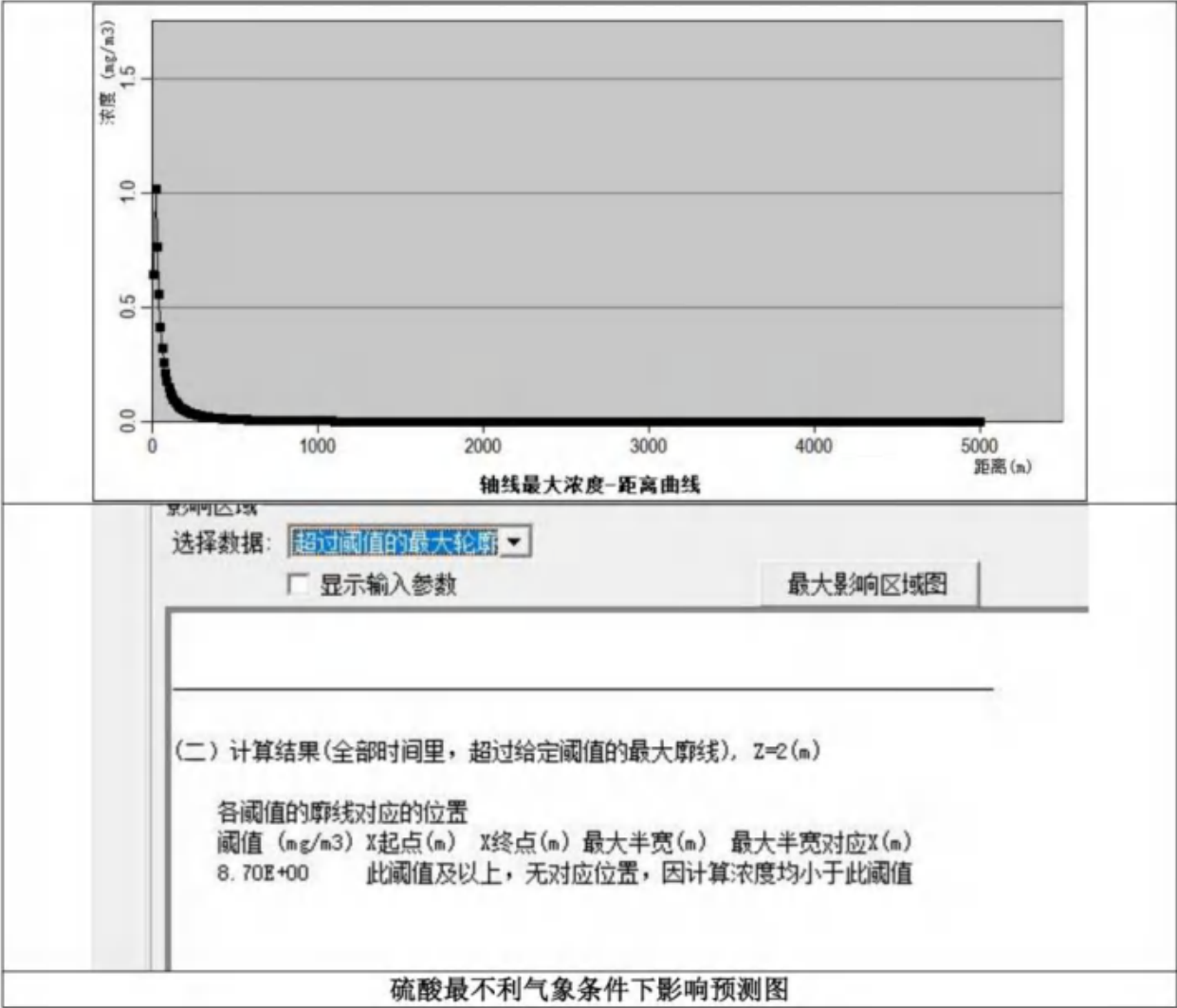
图 7.6-1 硫酸泄漏影响预测结果图
