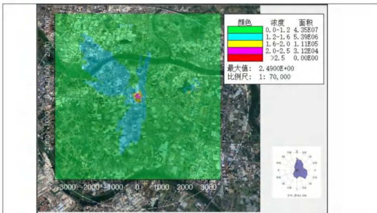
叠加后氯化氢日均浓度分布图 ( \mu\text{g}/\text{m}^3 )
