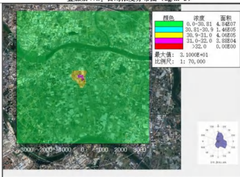
叠加后 NO 2 年均浓度分布图 (ug/m 3 )
