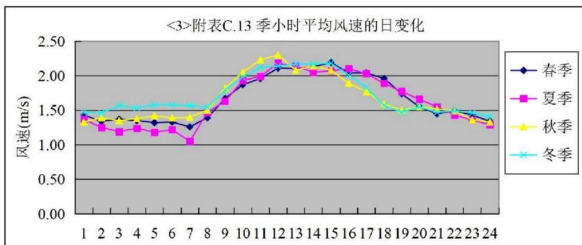
图 6.1-6 中山市 2023 年季小时平均风速日变化图
