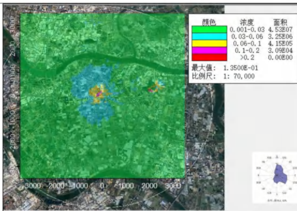
氨小时浓度贡献值预测图 ( \mu\text{g}/\text{m}^3 )
