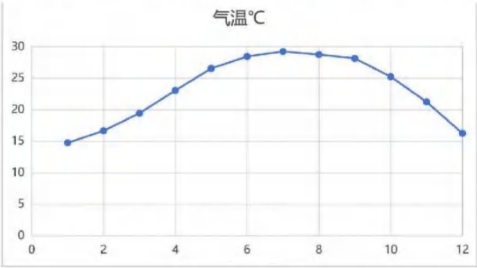
图 6.1-1 2004～2023 年中山市平均气温年变化
