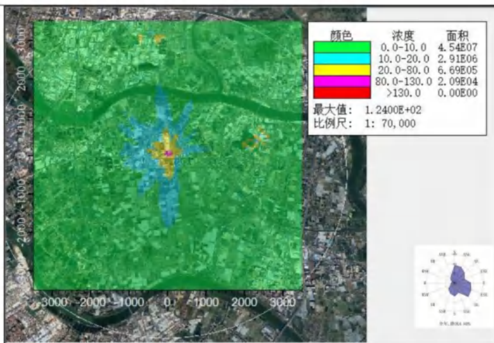
甲苯小时浓度贡献值预测图 ( \mu\text{g}/\text{m}^3 )
