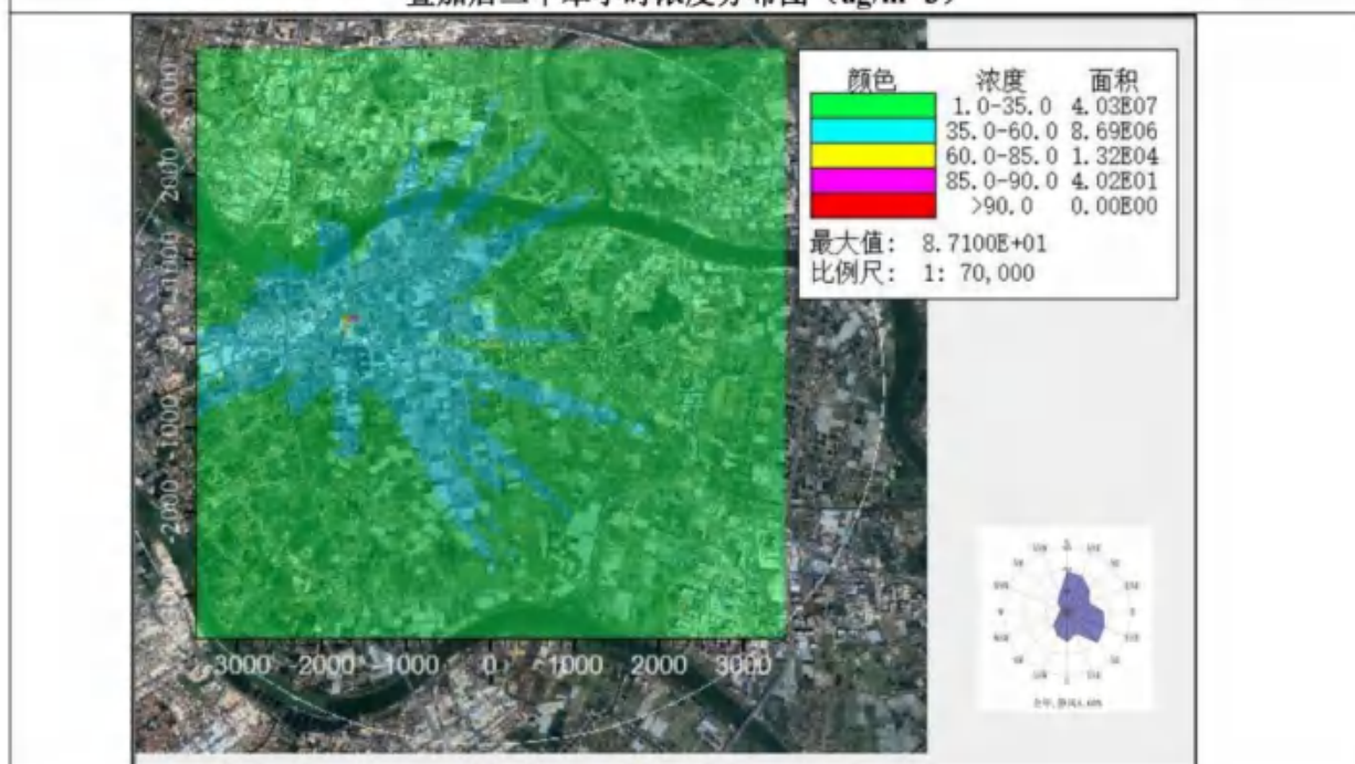
叠加后氨小时浓度分布图 ( \mu\text{g}/\text{m}^3 )
