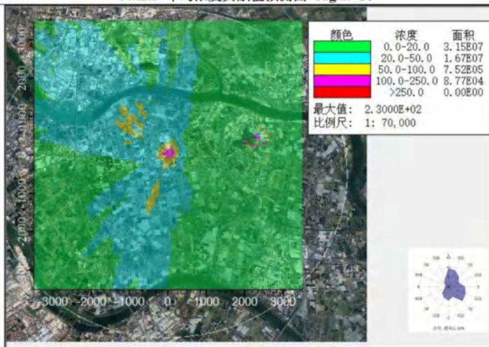
TVOC8 小时浓度贡献值预测图 (ug/m 3 )
