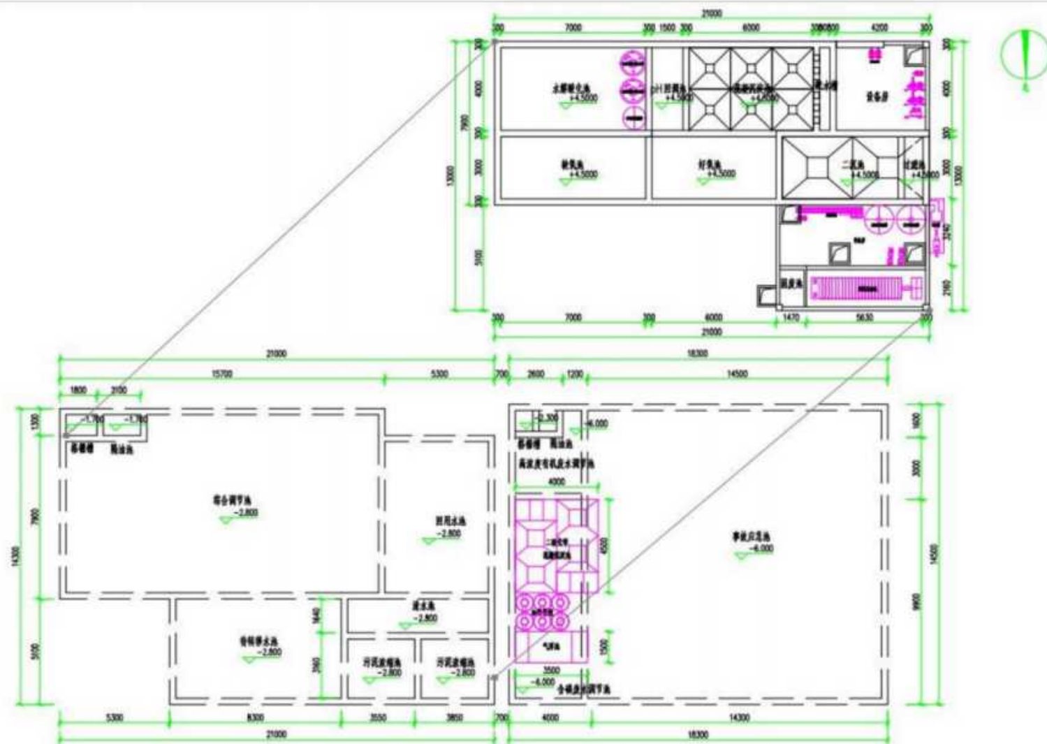
图 3.1-7 废水处理站布置图
