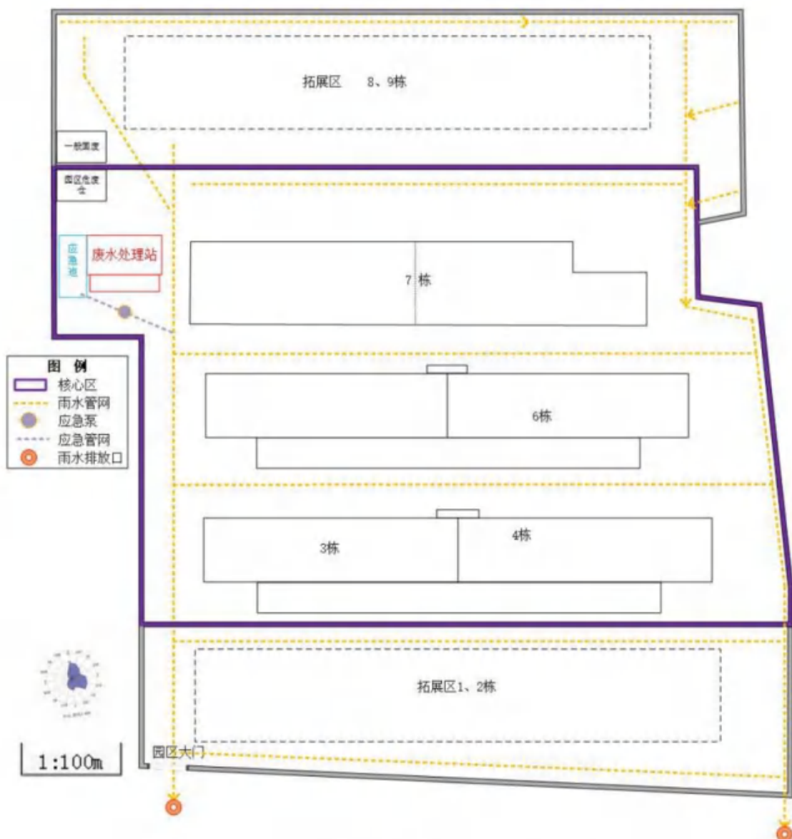
图 3.1-3 产业园雨水管网走向图
