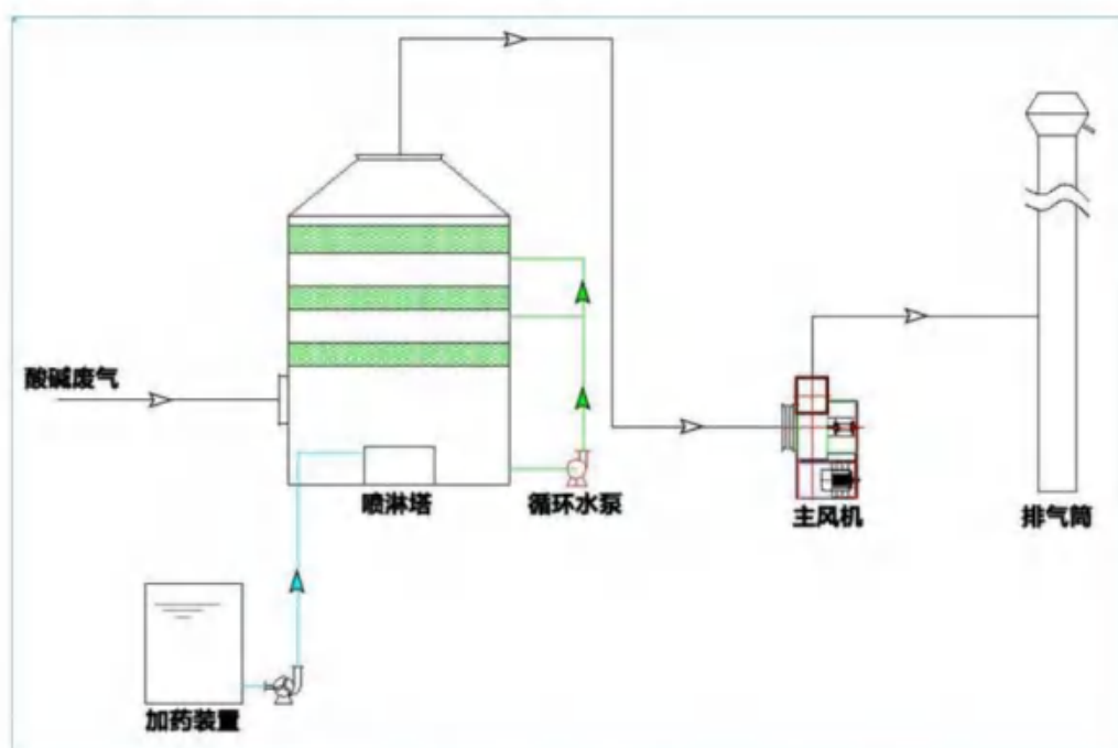
图 8.2-6 酸雾废气治理工艺流程图
