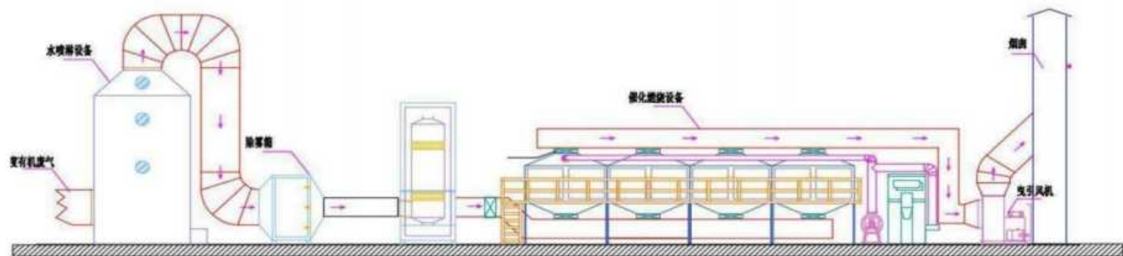
(高浓度) 有机废气废气治理系统示意图
