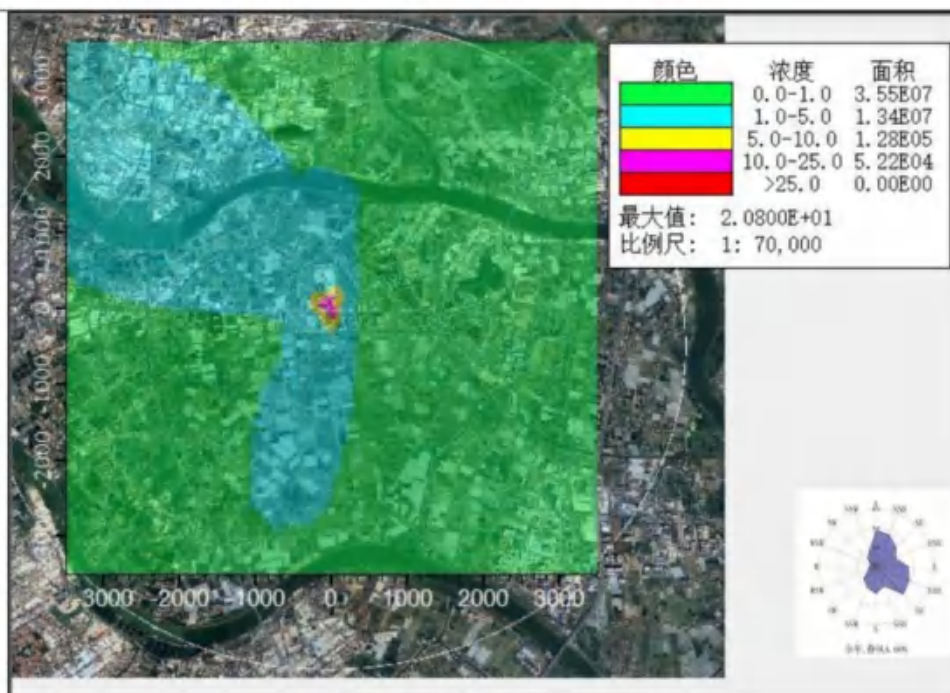
PM10 年均浓度贡献值预测图 ( \mu\text{g}/\text{m}^3 )
