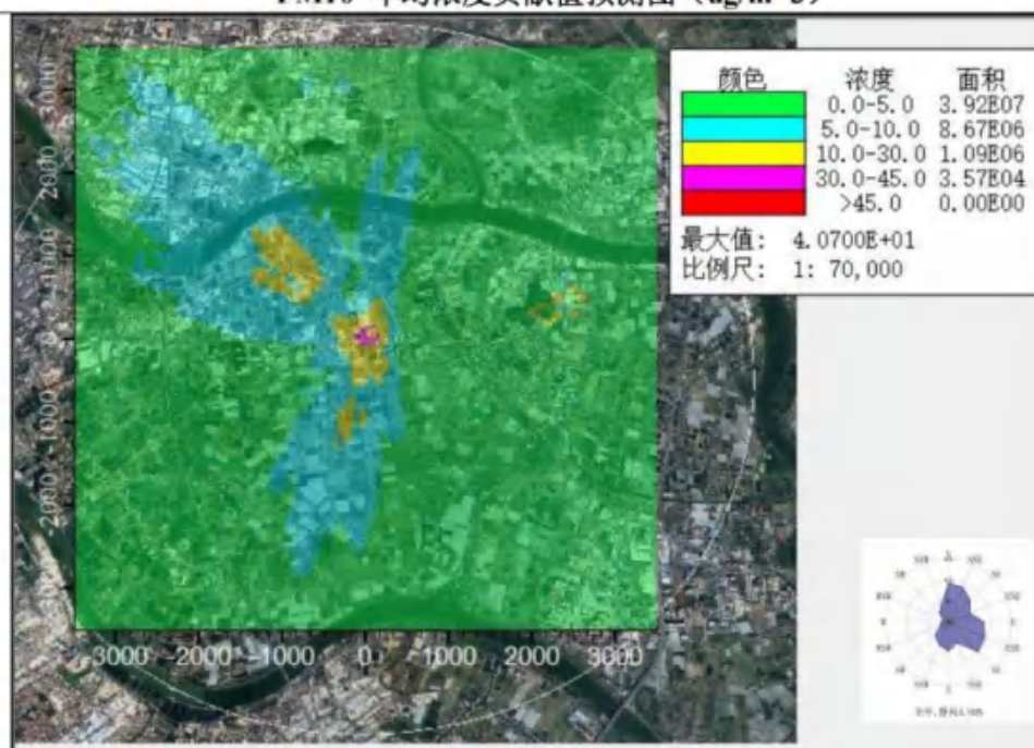
PM2.5 日均浓度贡献值预测图 ( \mu\text{g}/\text{m}^3 )
