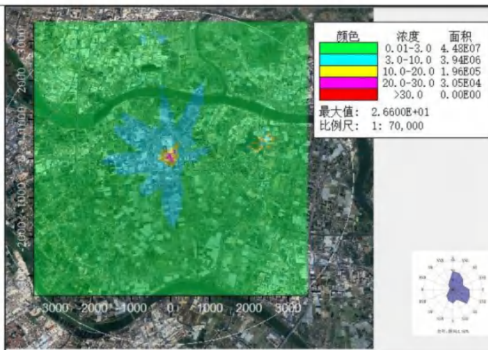
硫酸小时浓度贡献值预测图 (ug/m³)
