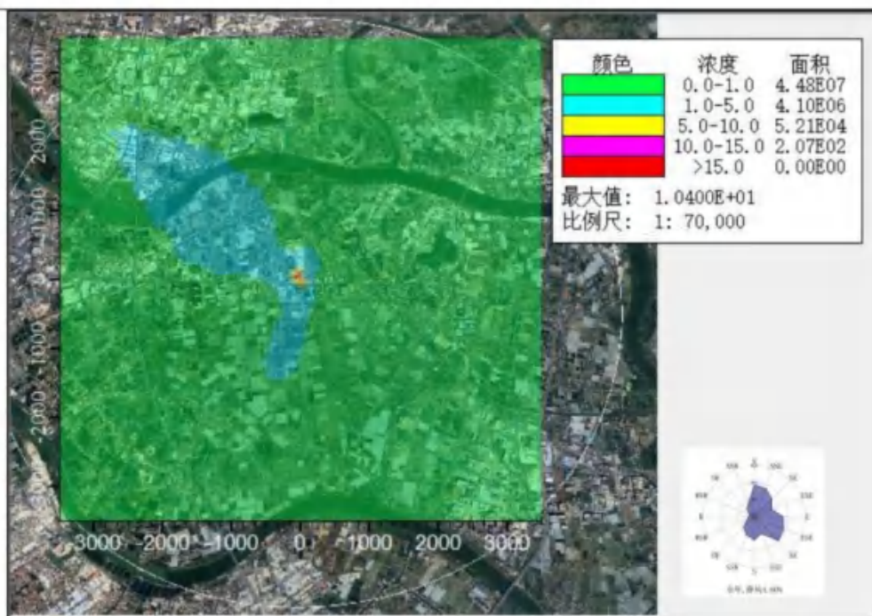
PM2.5 年均浓度贡献值预测图 (ug/m 3 )
