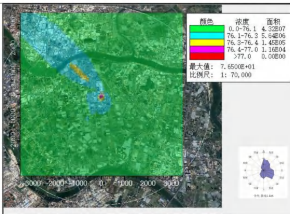
叠加后 NO 2 日均浓度分布图 (ug/m 3 )
