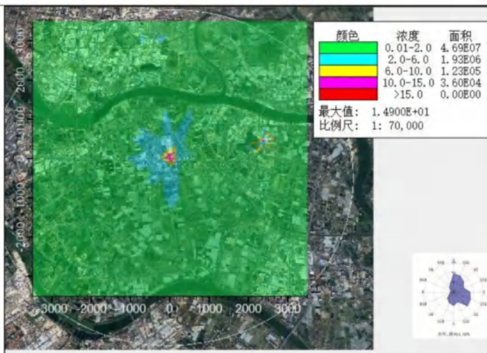
氯化氢小时浓度贡献值预测图 (ug/m 3 )
