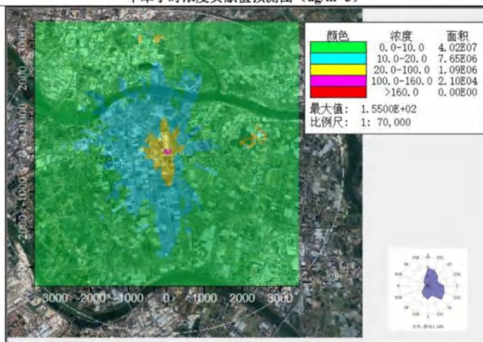
二甲苯小时浓度贡献值预测图 ( \mu\text{g}/\text{m}^3 )
