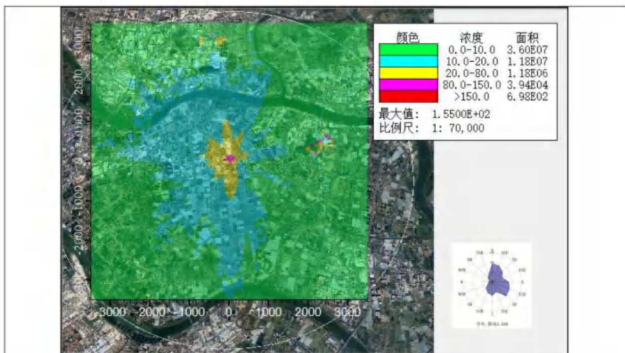
叠加后二甲苯小时浓度分布图 ( \mu\text{g}/\text{m}^3 )
