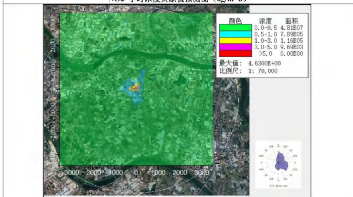
NO2 日均浓度贡献值预测图 (ug/m 3 )
