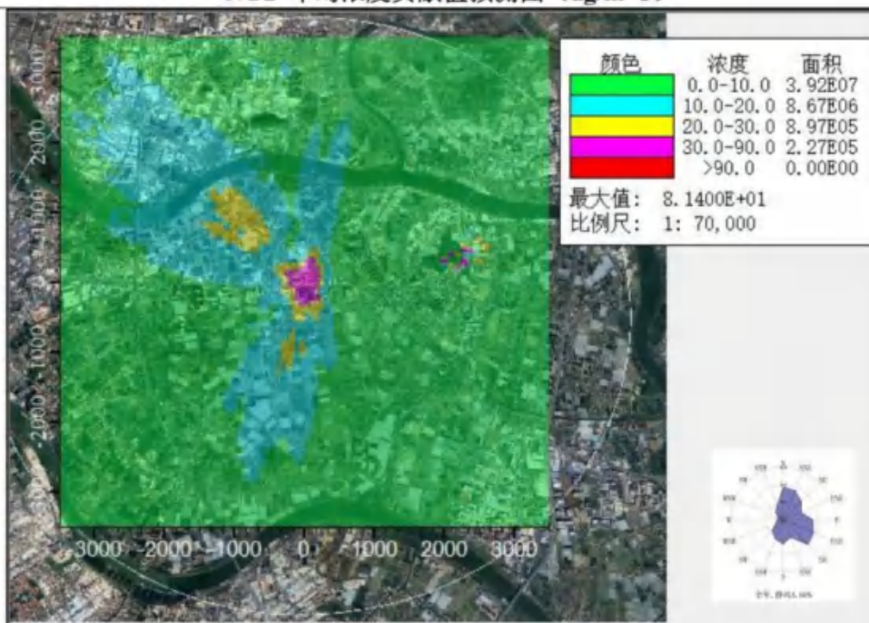
PM10 日均浓度贡献值预测图 ( \mu\text{g}/\text{m}^3 )
