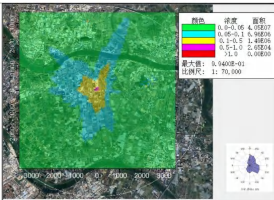
SO2 日均浓度贡献值预测图 ( \mu\text{g}/\text{m}^3 )
