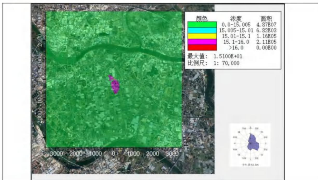
叠加后 SO 2 日均浓度分布图 (ug/m 3 )
