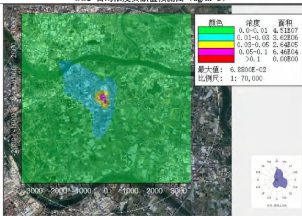
SO2 年均浓度贡献值预测图 ( \mu\text{g}/\text{m}^3 )
