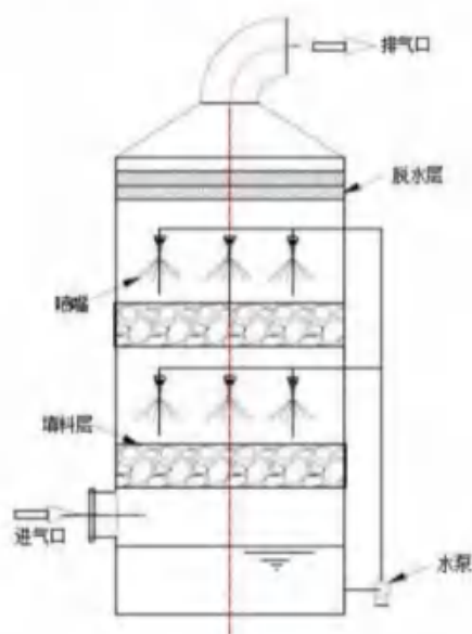
图 8.2-7 酸雾废气喷淋塔示意图
