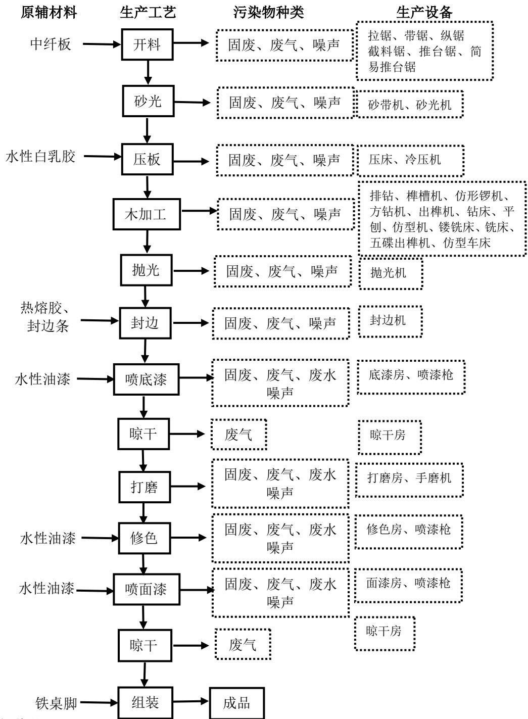
扩建部分餐桌生产工艺流程简述（流程图）
