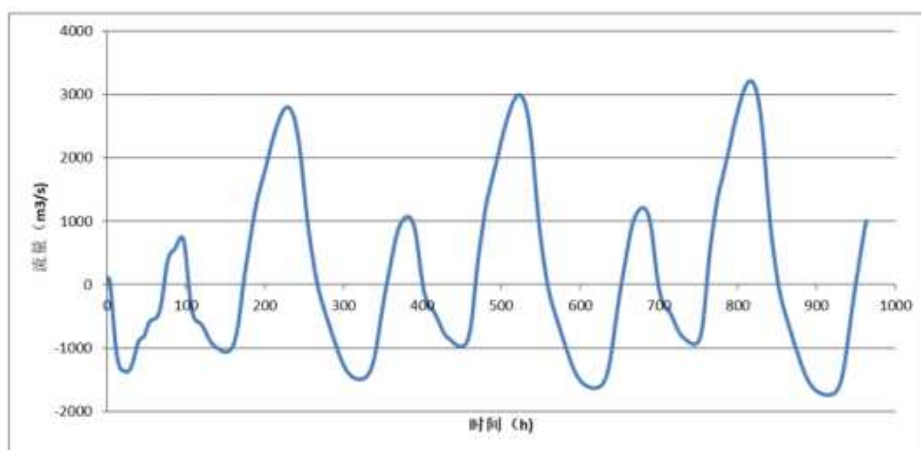
图7.2-13 排污口附近断面流量过程示意图（丰水期）
