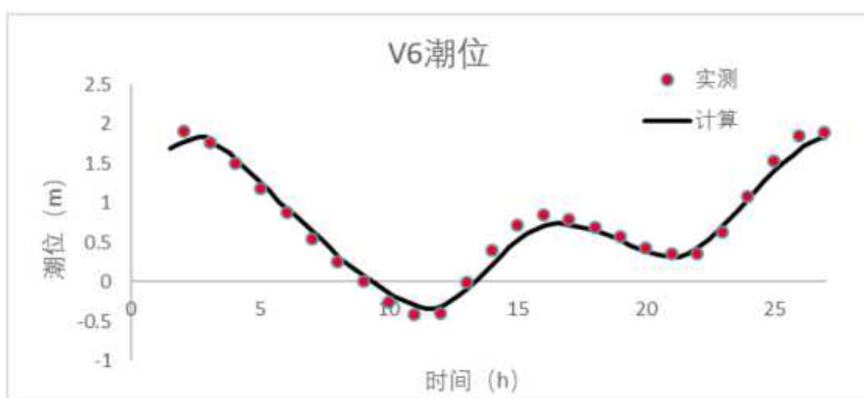
图7.2-9 潮位验证情况（2021年7月11日9:00-12日12:00）
