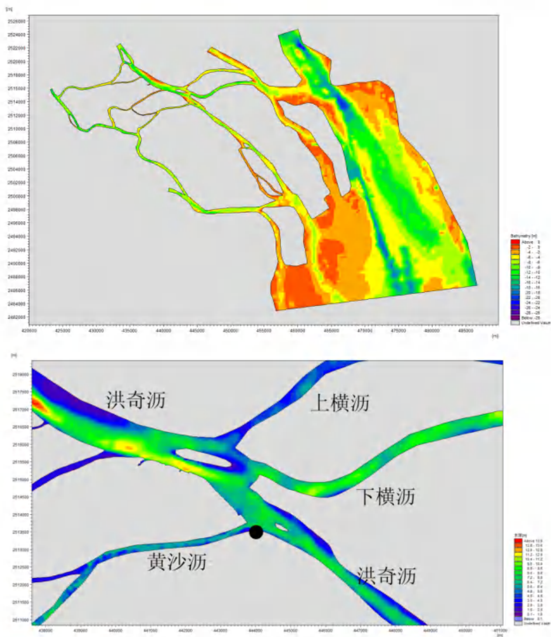
图7.2-4 项目地附近水下地形
