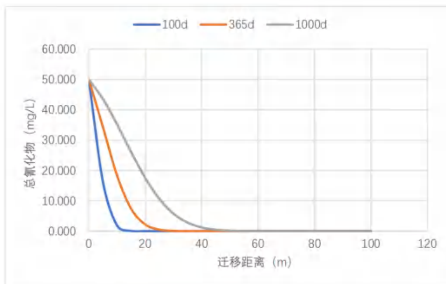
图7.4-10 总氰化物不同泄漏时间（100d、365d 及 1000d）运移范围预测图
