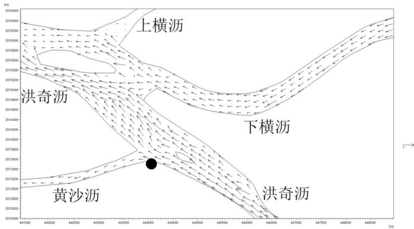
图7.2-16 模拟区域丰水期涨急流场流速图
