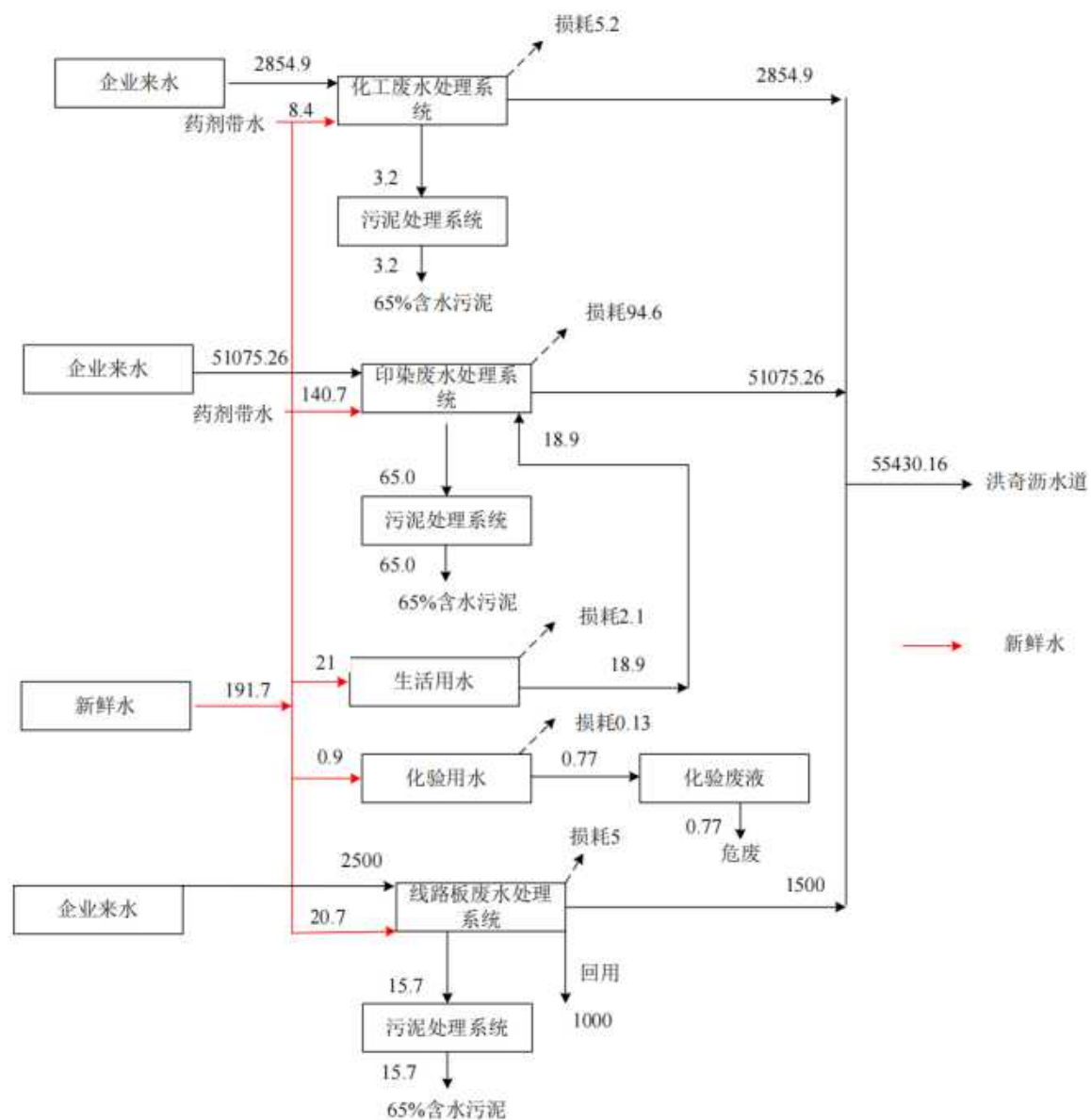
图4.1-6 改扩建后全厂水平衡图 单位: \text{m}^3/\text{d}
