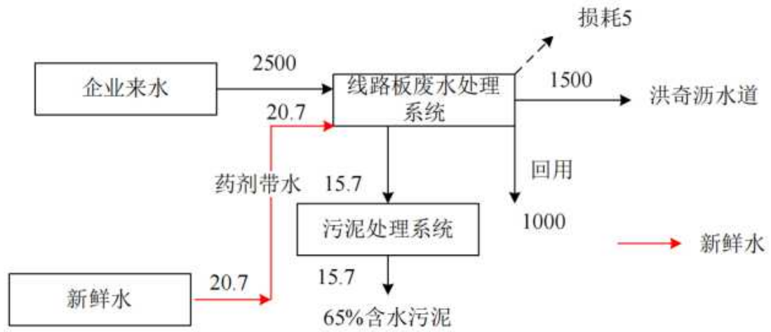
图4.1-5 改扩建项目水平衡图 单位: \text{m}^3/\text{d}
