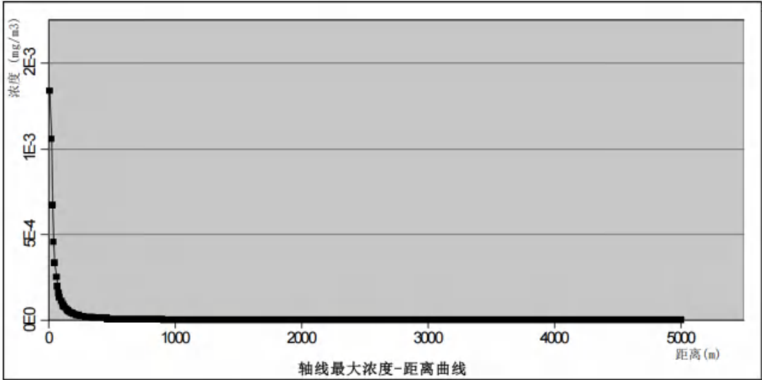
图8.7-3 次氯酸钠轴线最大浓度-距离轴线图
