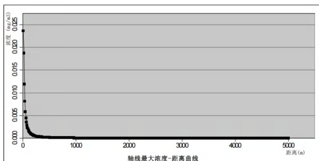
图8.7-4 盐酸轴线最大浓度-距离轴线图
