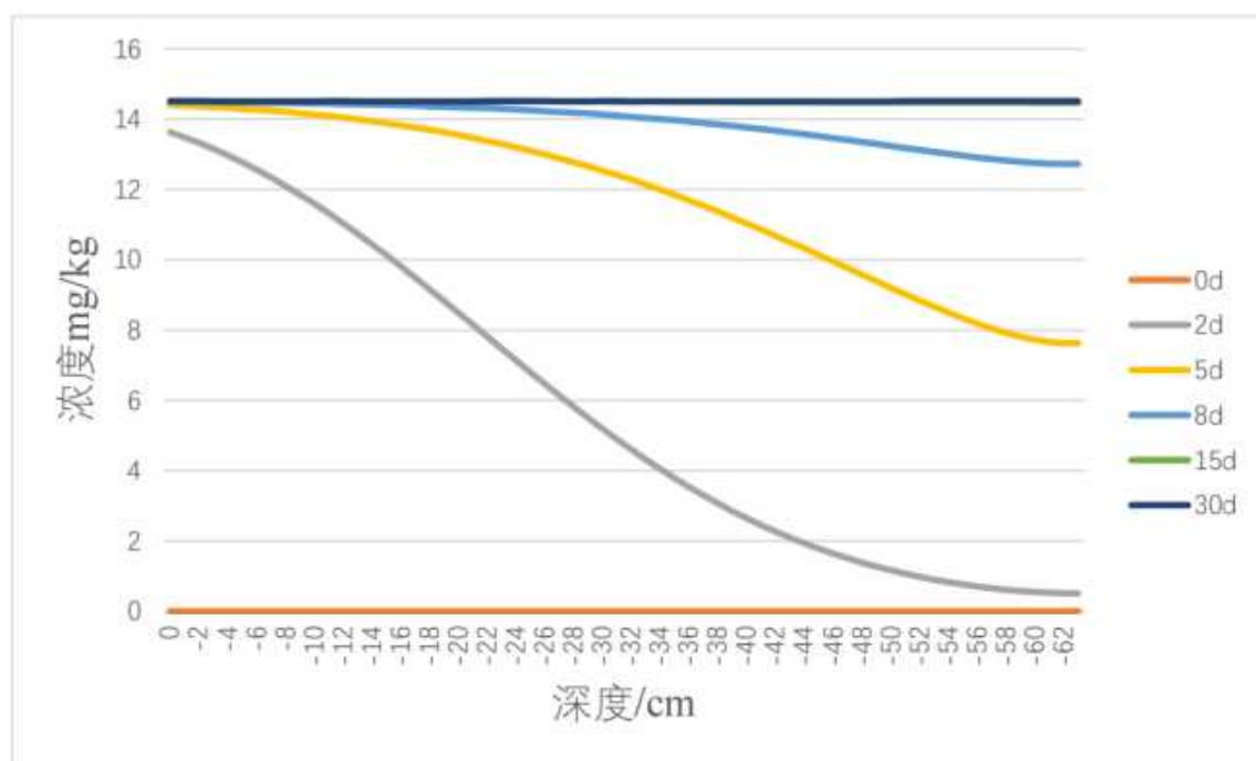
图7.5-6 总镍垂直入渗不同时间浓度随深度变化图
