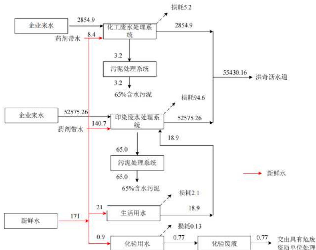
图3.3-1 现有工程水平衡图 单位: \text{m}^3/\text{d}
