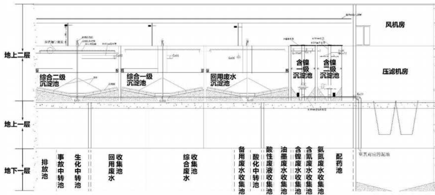
废水处理站立面图
