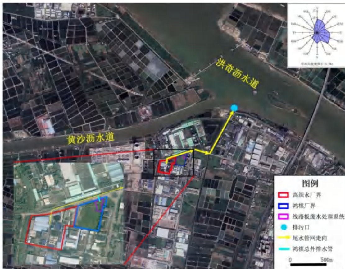
图4.1-4 本项目尾水排放路径及排污口位置图
