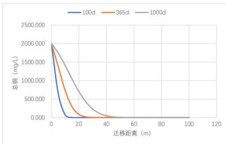
图7.4-6 总铜不同泄漏时间（100d、365d 及 1000d）运移范围预测图
