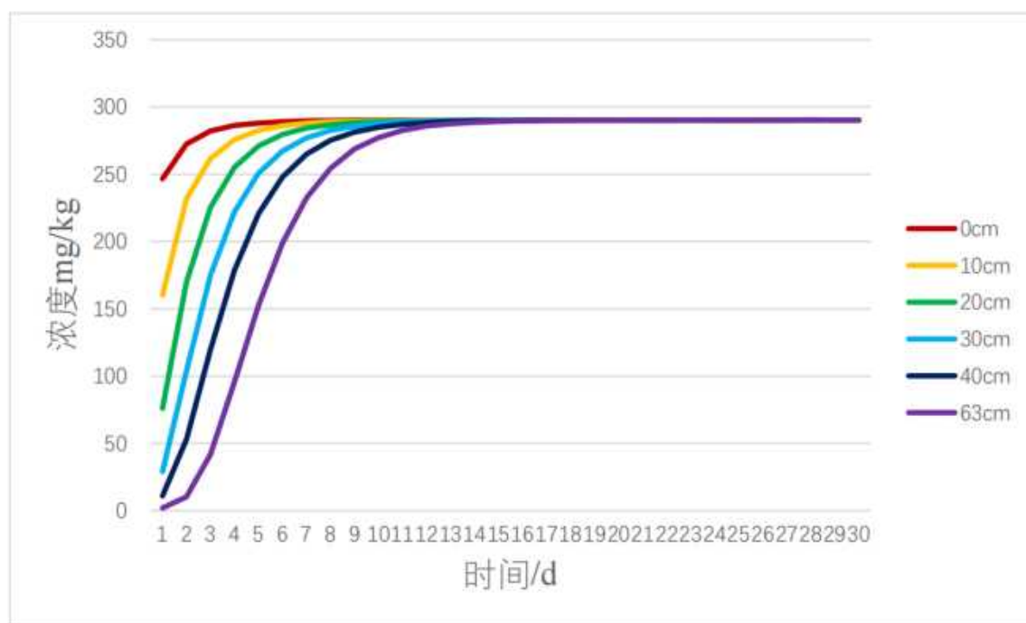
图7.5-3 总铜垂直入渗浓度随时间变化图
