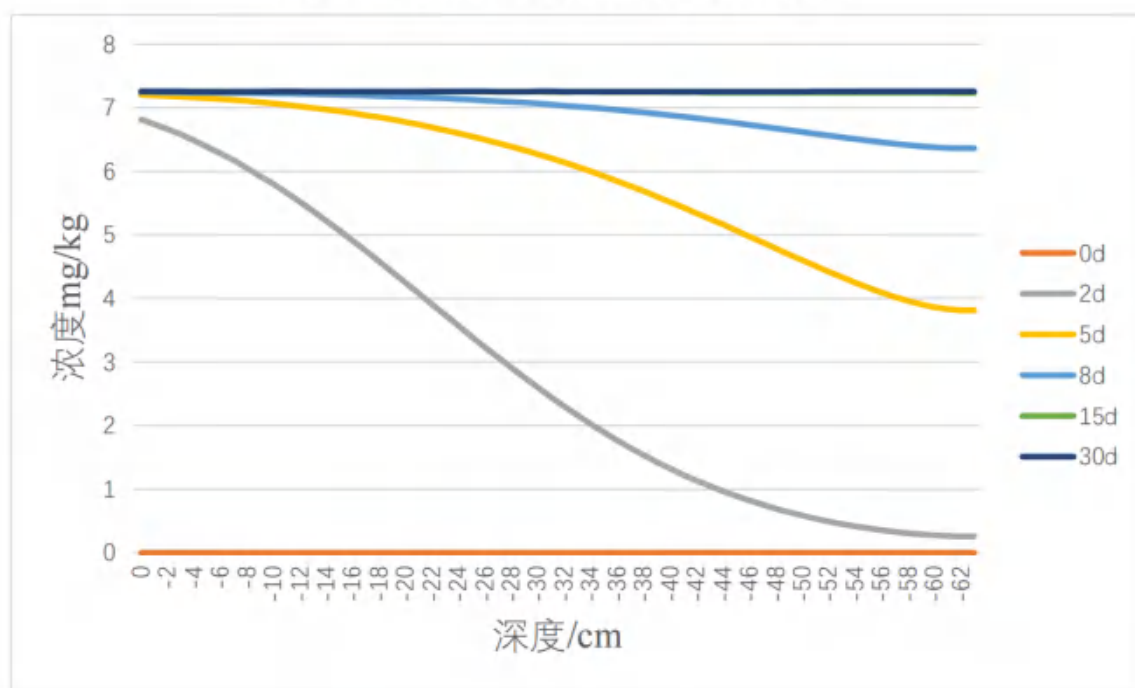
图7.5-8 总氰化物垂直入渗不同时间浓度随深度变化图
