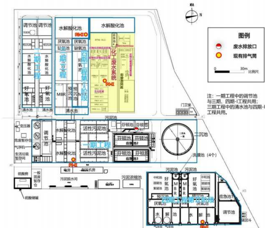
图3.2-2 现有工程总平面布置图
