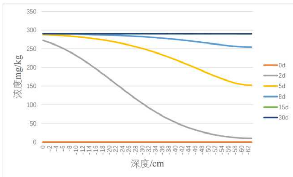
图7.5-2 COD 垂直入渗不同时间浓度随深度变化图
