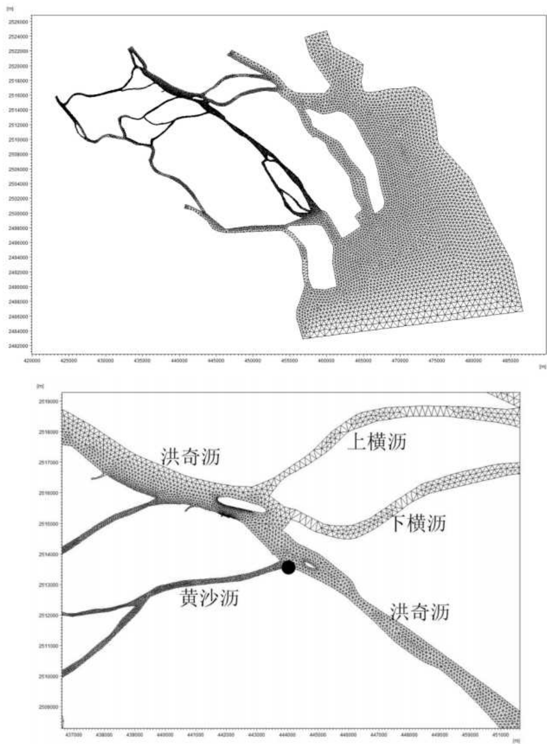
图7.2-3 项目地附近模型水平计算网格布置
