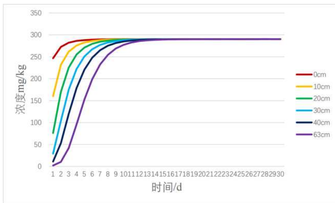
图7.5-1 COD 垂直入渗浓度随时间变化图
