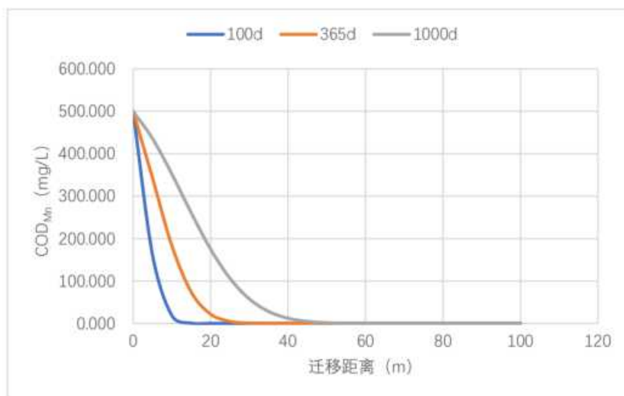
图7.4-8 COD 不同泄漏时间（100d、365d 及 1000d）运移范围预测图
