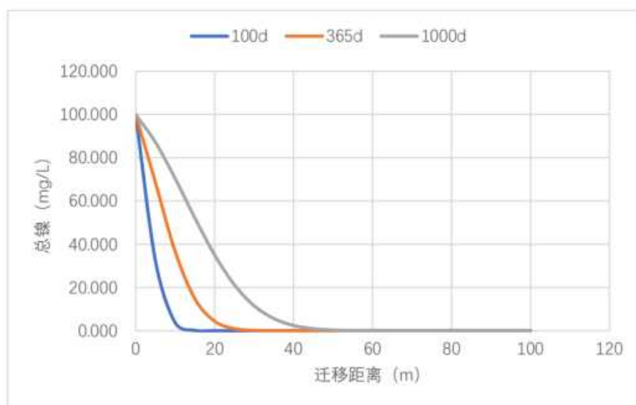
图7.4-7 总镍不同泄漏时间（100d、365d 及 1000d）运移范围预测图
