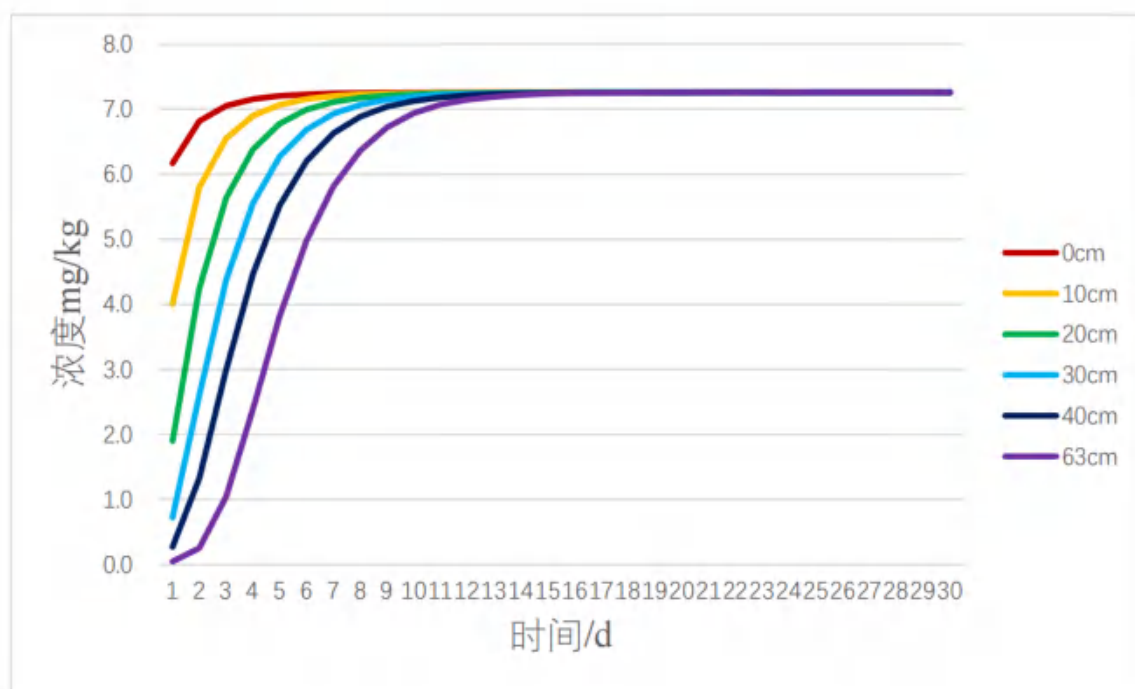
图7.5-7 总氰化物垂直入渗浓度随时间变化图
