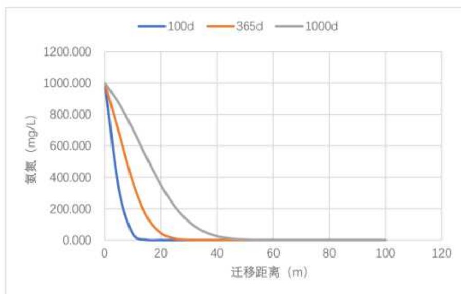
图7.4-9 氨氮不同泄漏时间（100d、365d 及 1000d）运移范围预测图
