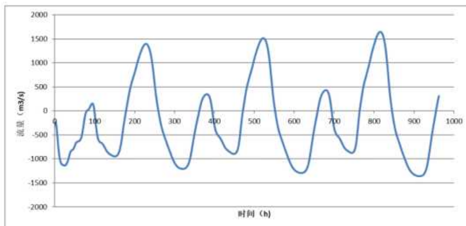
图7.2-12 排污口附近断面流量过程示意图（枯水期）
