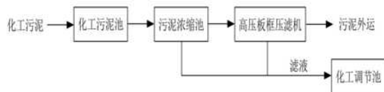
图3.4-1 化工废水处理工艺流程图
