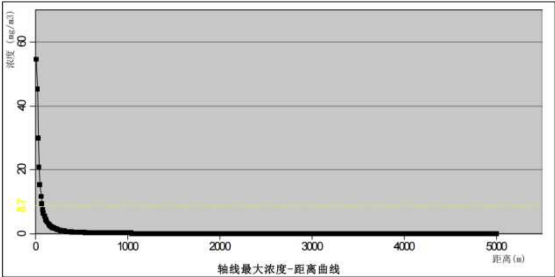
图8.7-1 硫酸轴线最大浓度-距离轴线图
