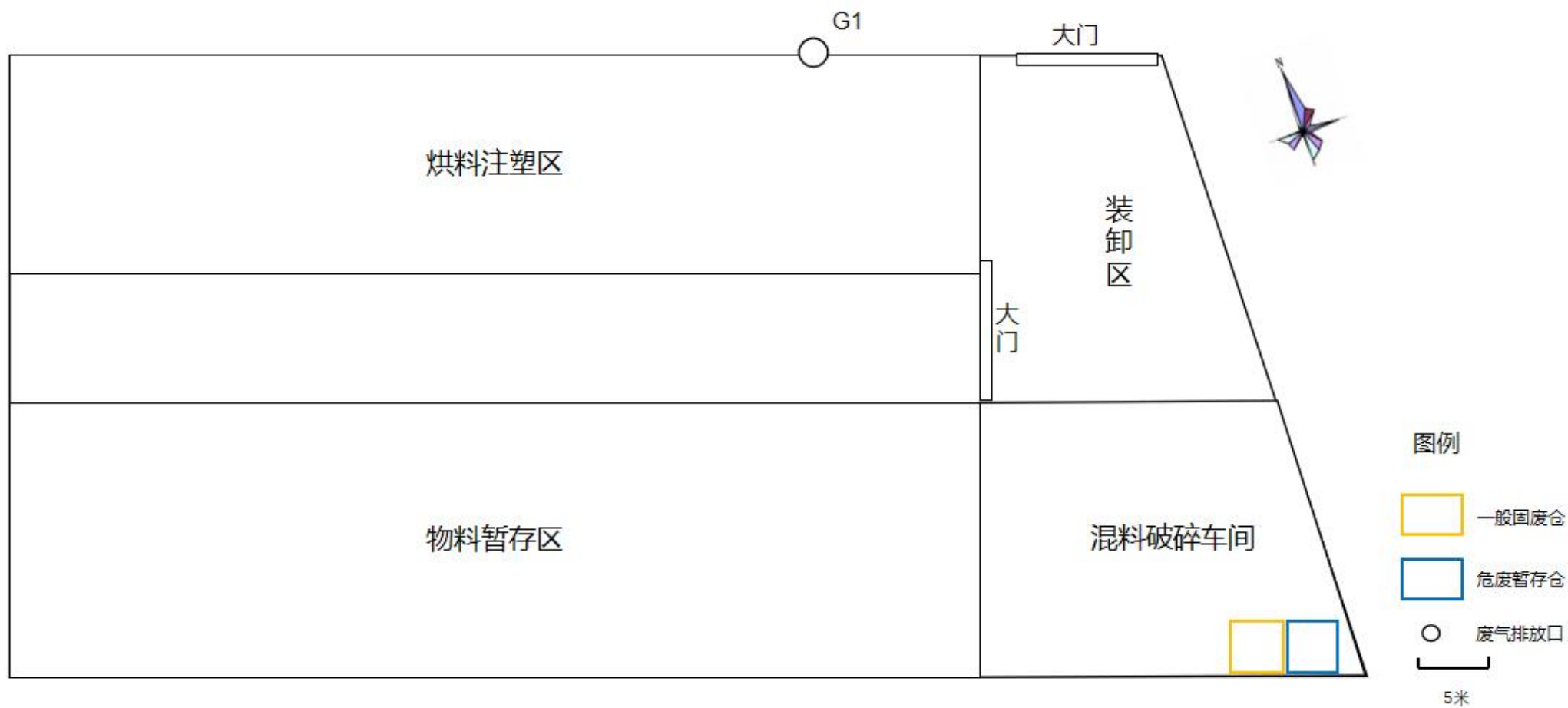
附图3 生产车间平面布置图
