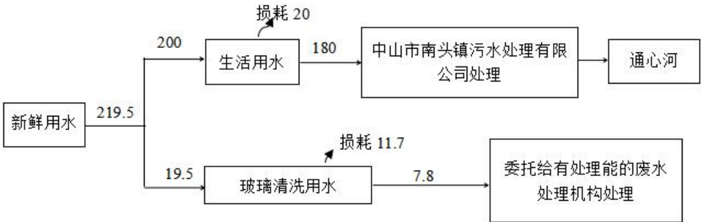
图 1 项目水平衡图（单位：t/a）
