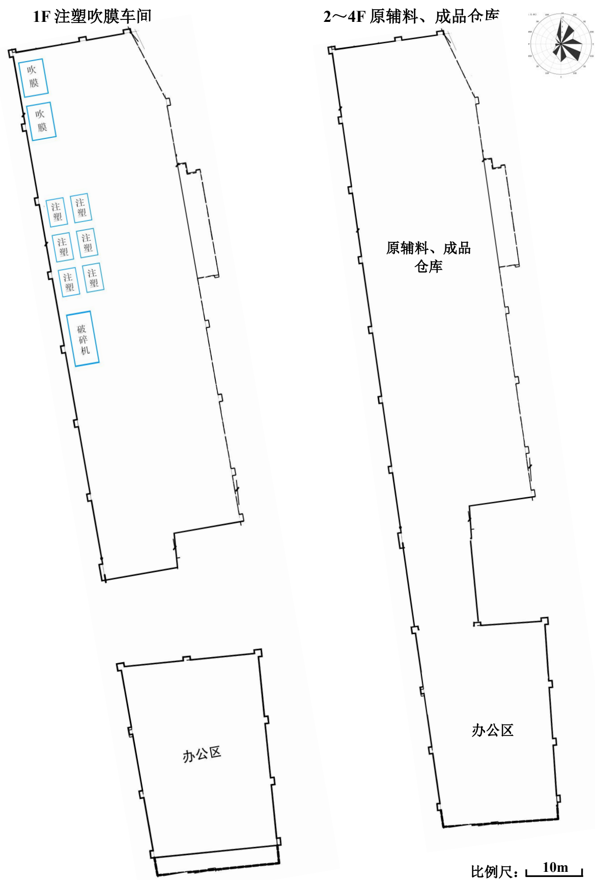
图 4.1-5 项目生产厂房分层平面布置图（1F 和 2-4F）
