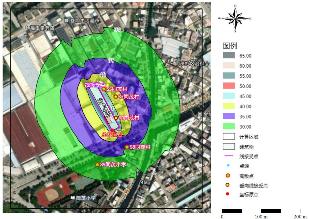
图 6.3-1 项目噪声贡献值等声线图（昼间）
