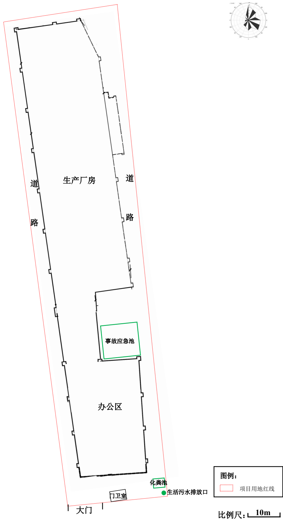
图 4.1-4 项目厂区总平面布置图
