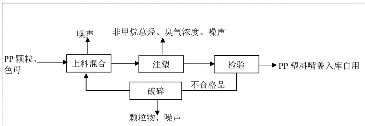
图 4.3-2 项目注塑工艺流程及产污环节图
