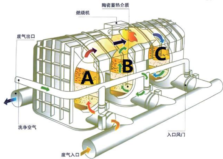
图 8.1-1 RTO 炉运行原理图
