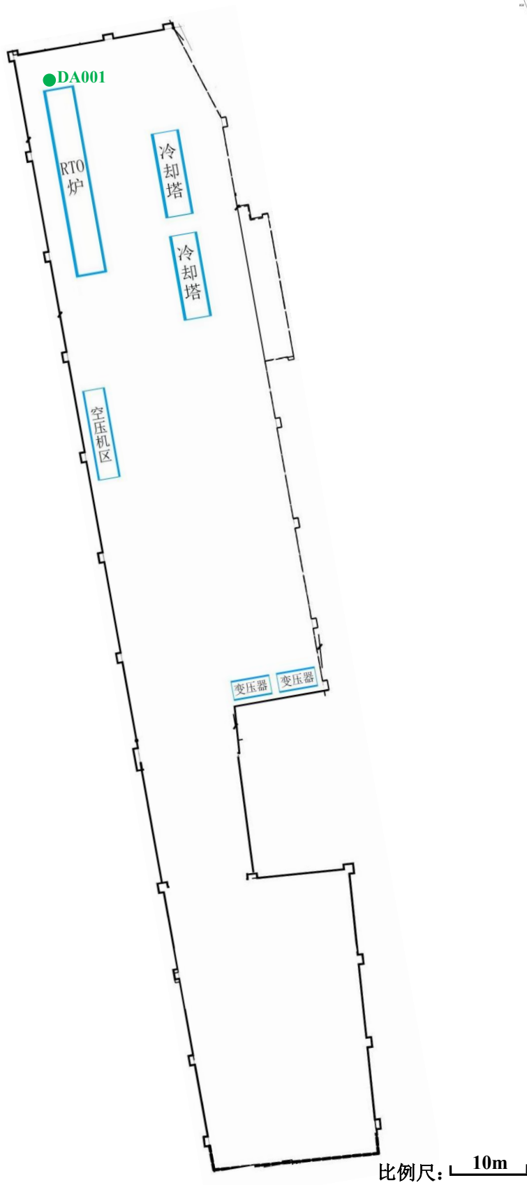
图 4.1-8 项目生产厂房分层平面布置图（8F 楼顶）
