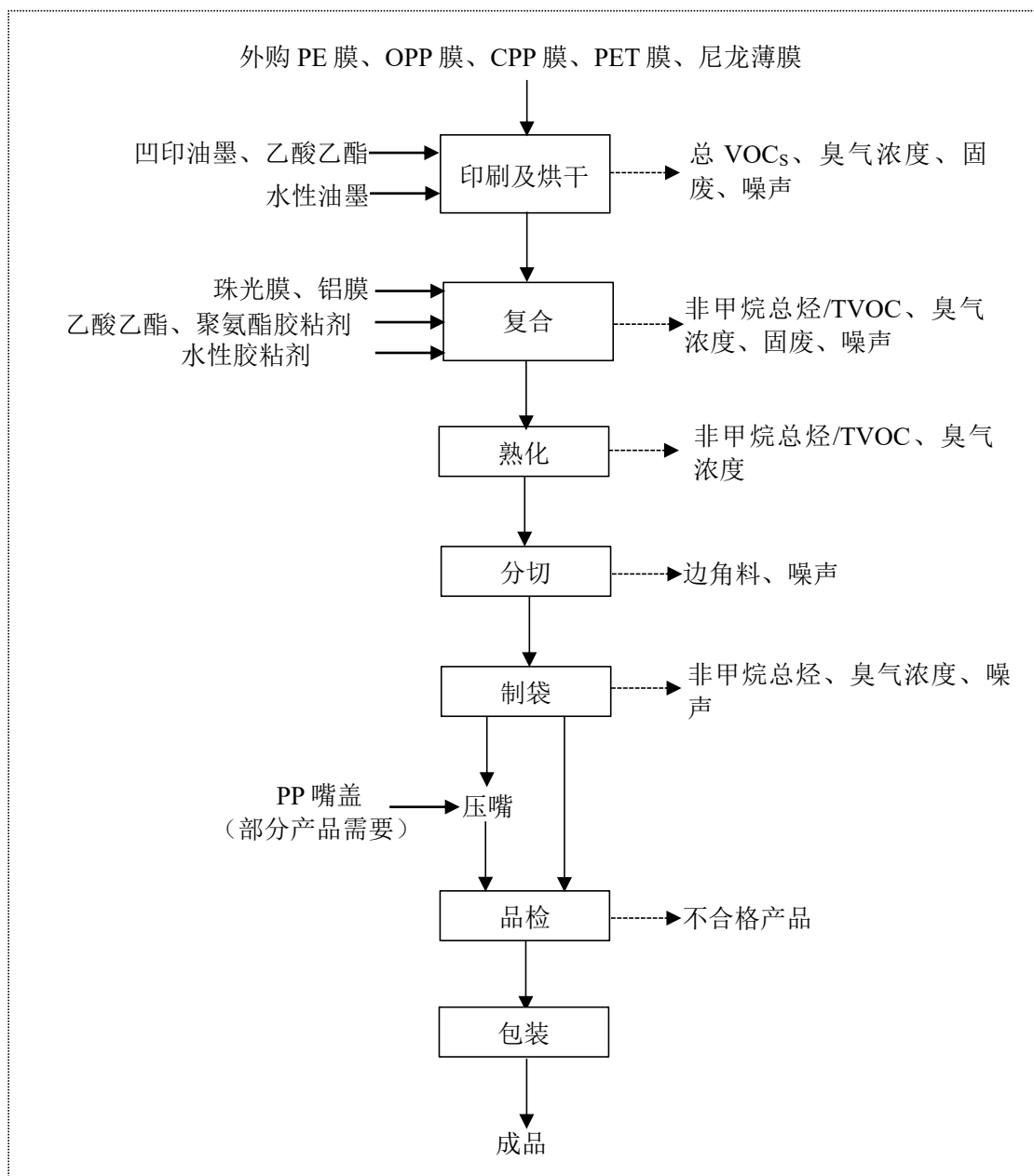
图 4.3-3 项目包装膜袋生产工艺流程和产污环节图
