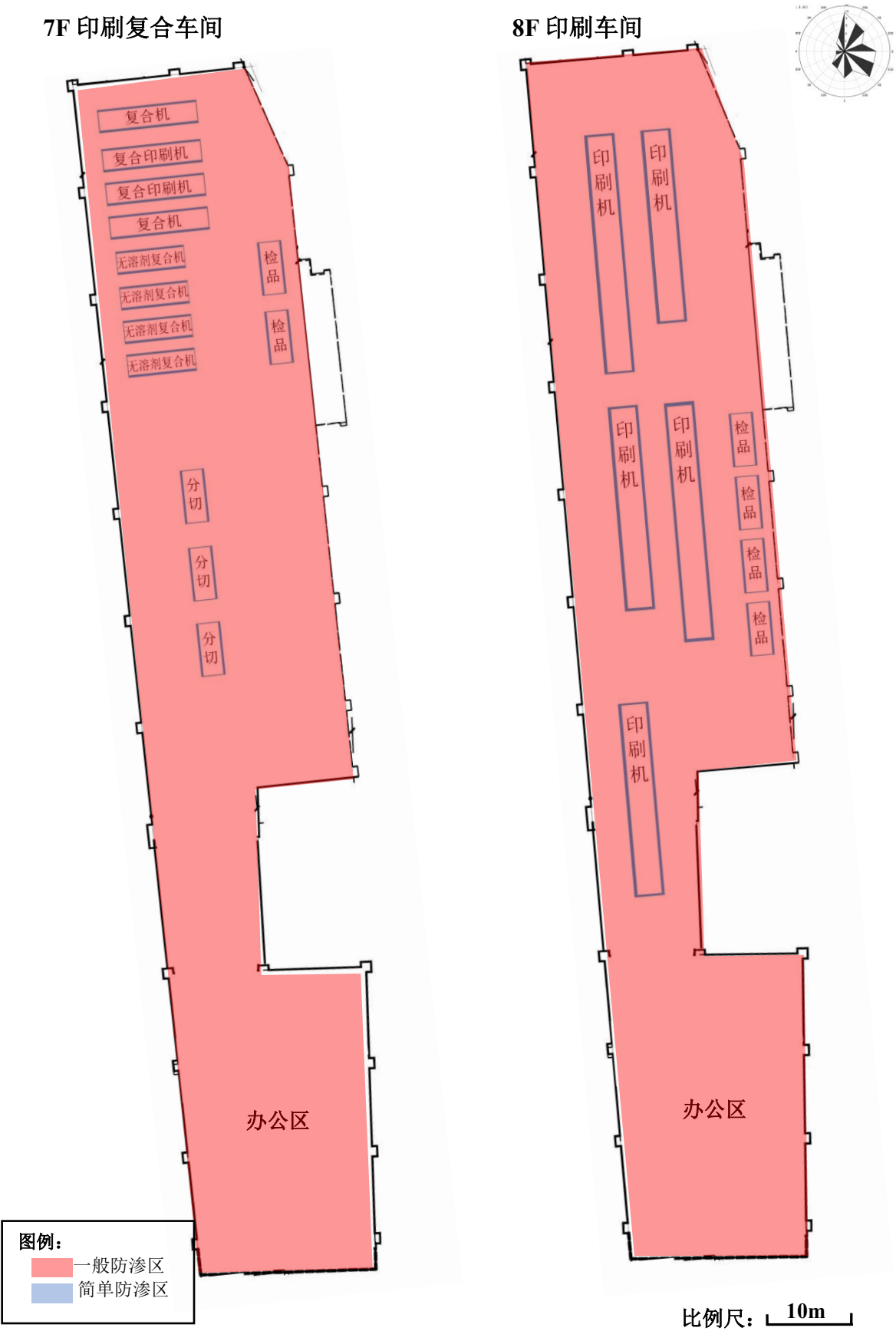
图 8.5-3 项目地下水污染防渗分区图（7F 和 8F）
