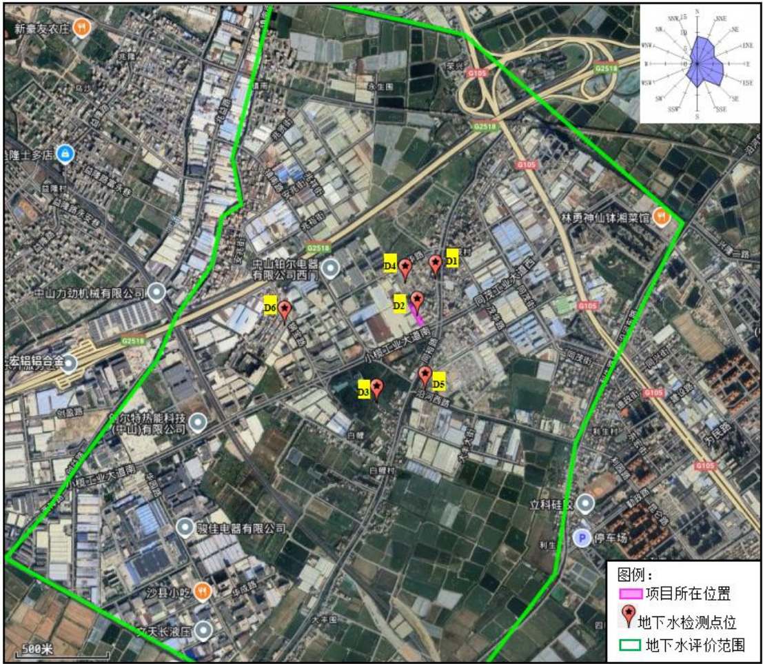
图 5.2-3 项目地下水监测点位图
