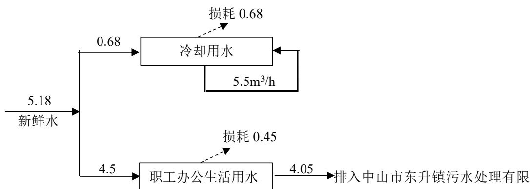
图 4.4-1 全厂水平衡图（ \text{m}^3/\text{d} ）
