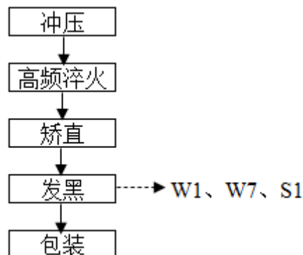
图 3.3-18 木工尺铁条生产工艺流程
