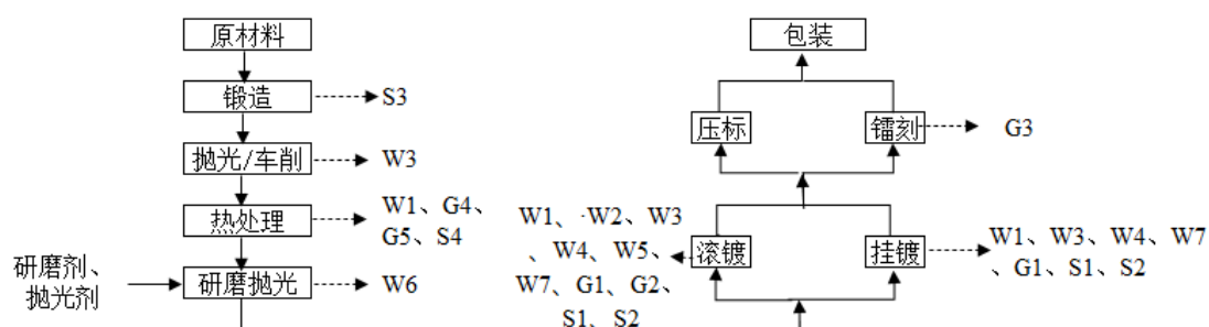
图 3.3-7 套筒（B 类）生产工艺流程
