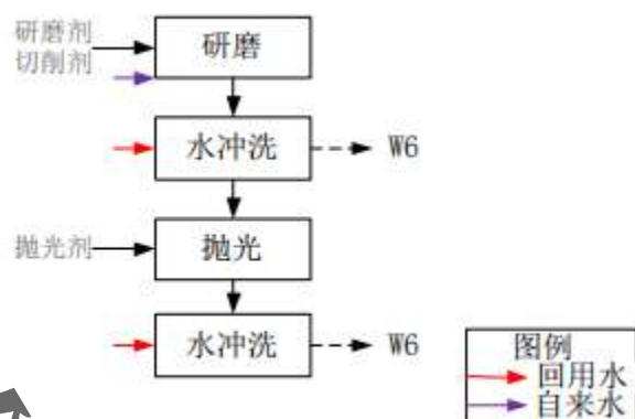
图 3.3-24 研磨抛光工艺流程图
