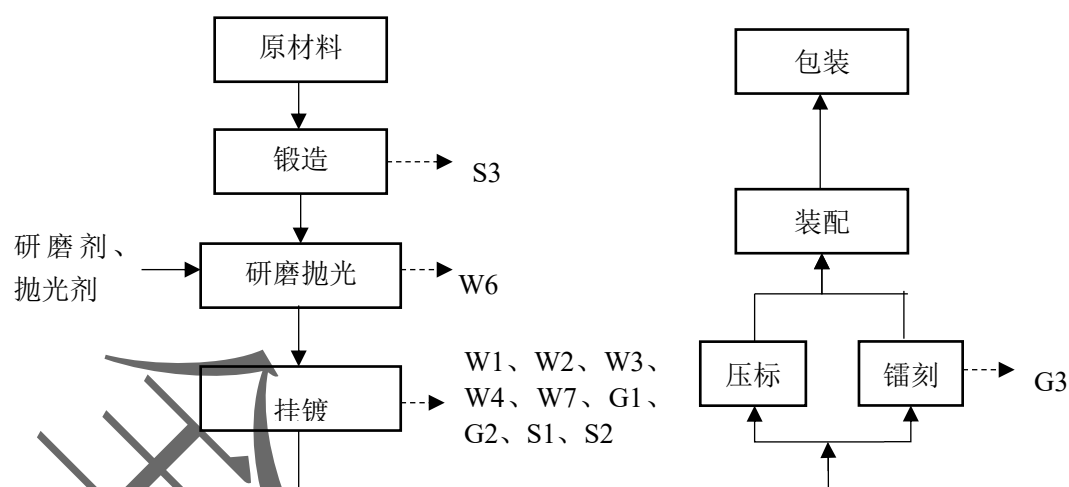
图 3.3-12 H 柄（C 类）生产工艺流程图
