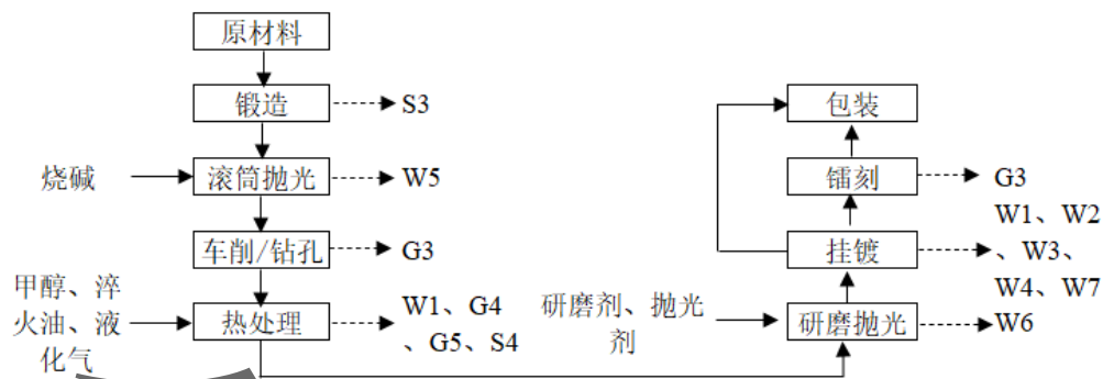
图 3.3-2 扳手生产工艺流程图
