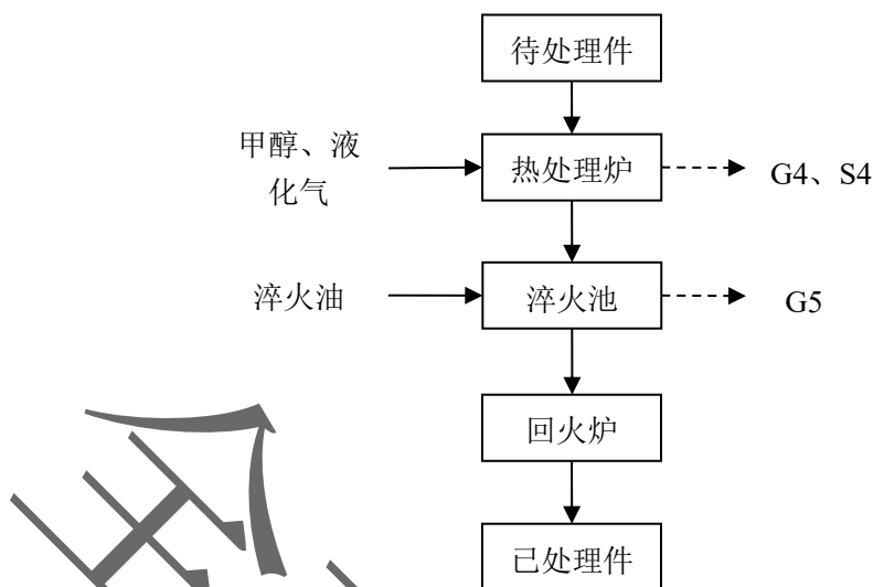
图 3.3-26 热处理工艺流程
