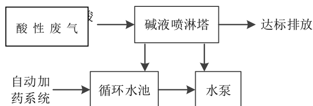
图 7.2-1 氯化氢废气治理工艺流程图
