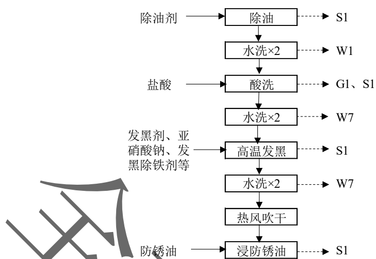
图 3.3-20 发黑（C类）工序工艺流程图
