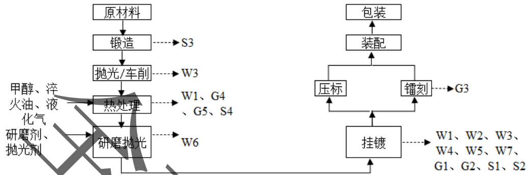
图 3.3-10 H 柄（a 类）生产工艺流程图
