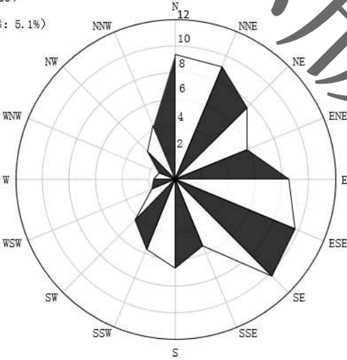
图 6.3-4 中山市 2004-2023 年风向玫瑰图
