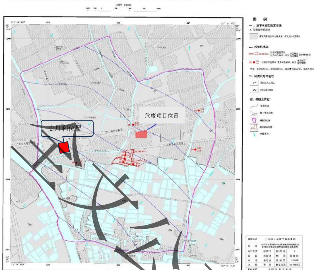
中山市小榄镇龙山电镀基地危险废物综合利用项目水文地质勘查区域水文地质图
