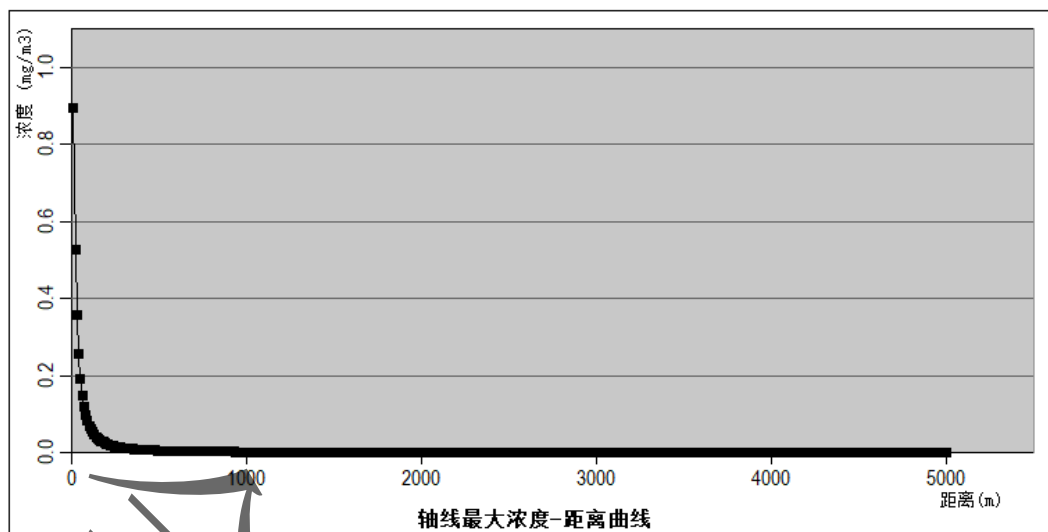
图 6.7-12 CO排放事故最大浓度-距离曲线图
