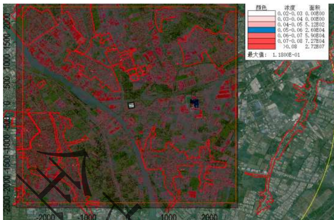
图 6.3-20 项目污染源 PM_{10} 最高贡献浓度预测结果-日均值-叠加值
