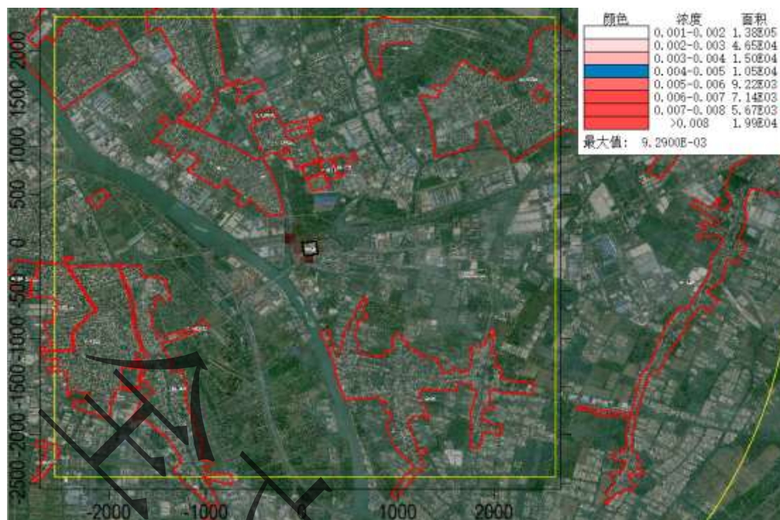
图 6.3-19 项目污染源 TSP 最高贡献浓度预测结果-年均值
