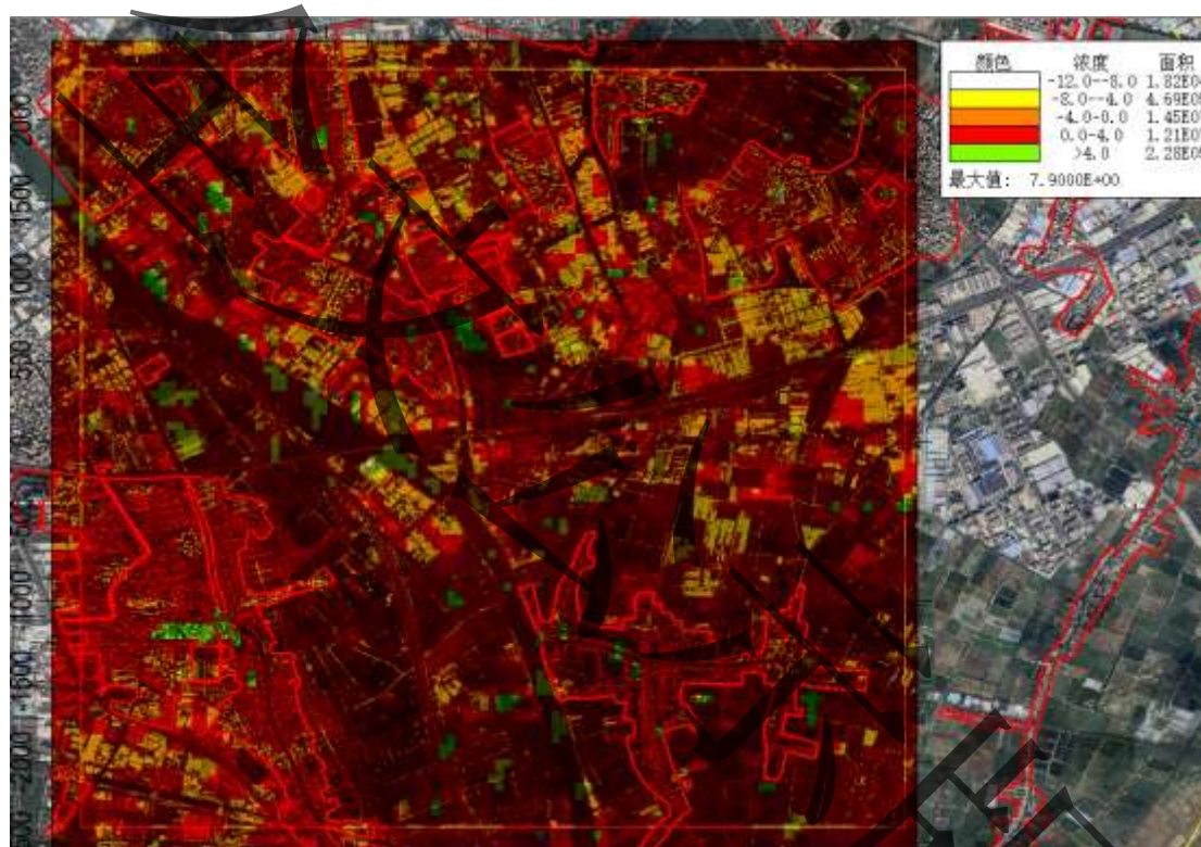
图 6.3-10 预测范围区域地形图
