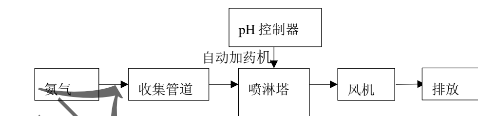
图 7.2-2 氨气废气治理工艺流程图
