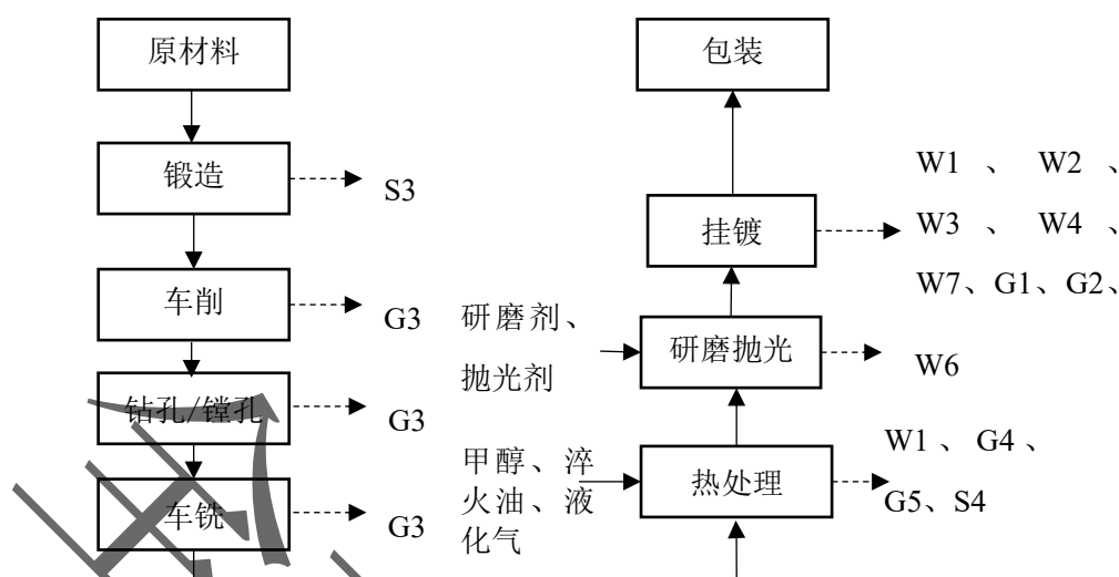
图 3.3-16 D 头（B 类）生产工艺流程图
