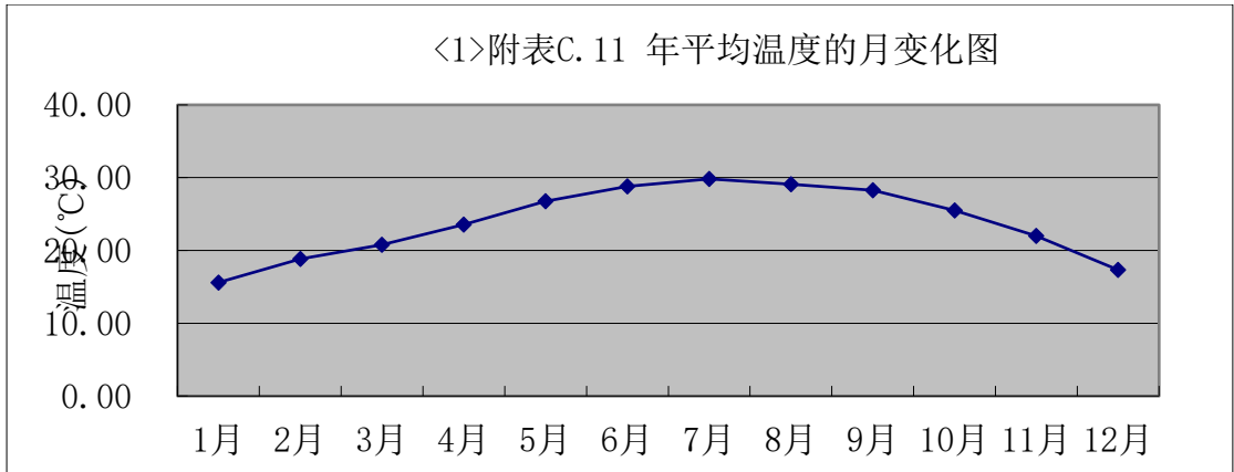
图 6.3-6 中山市 2023 年平均温度月变化图
