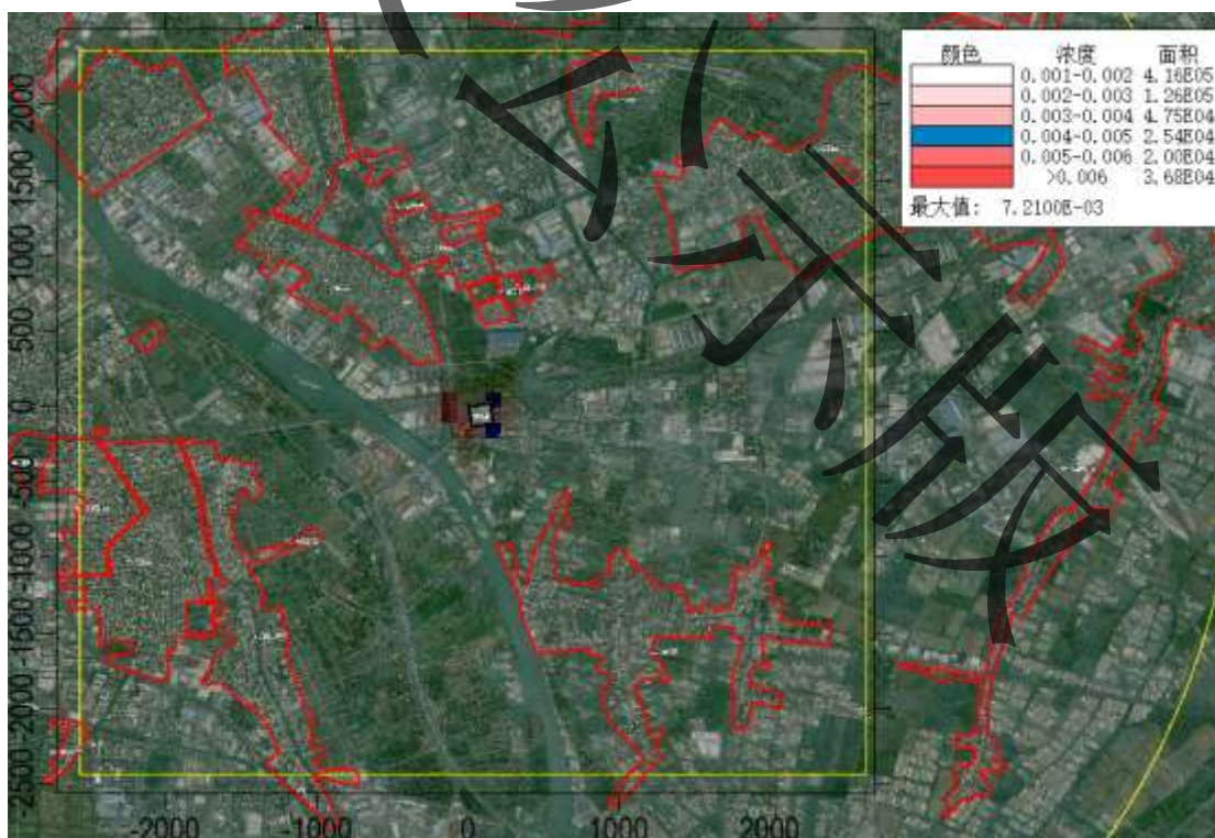
图 6.3-15 项目污染源氯化氢最高贡献浓度预测结果-小时均值
