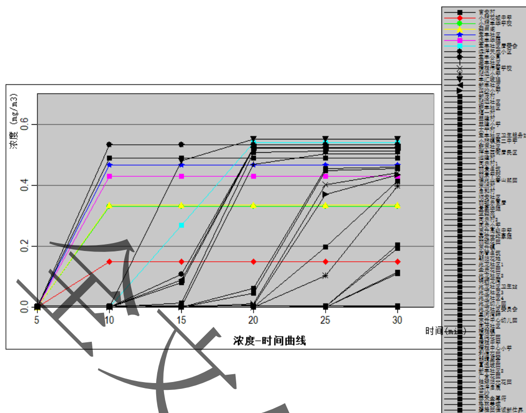
图 6.7-10 甲醇泄漏事故各关心点浓度随时间的变化曲线图
