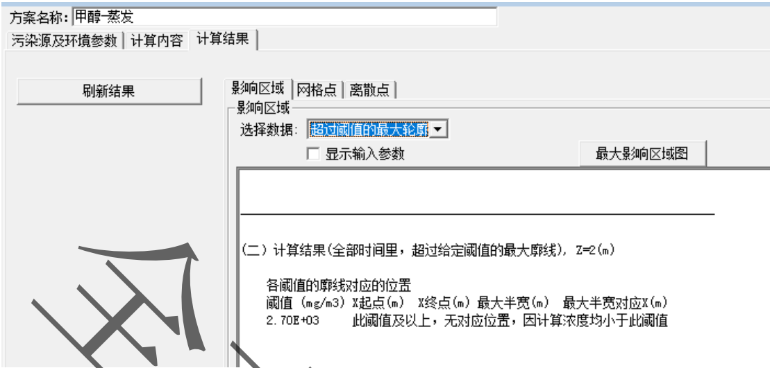
图 6.7-8 甲醇泄漏事故预测结果图
