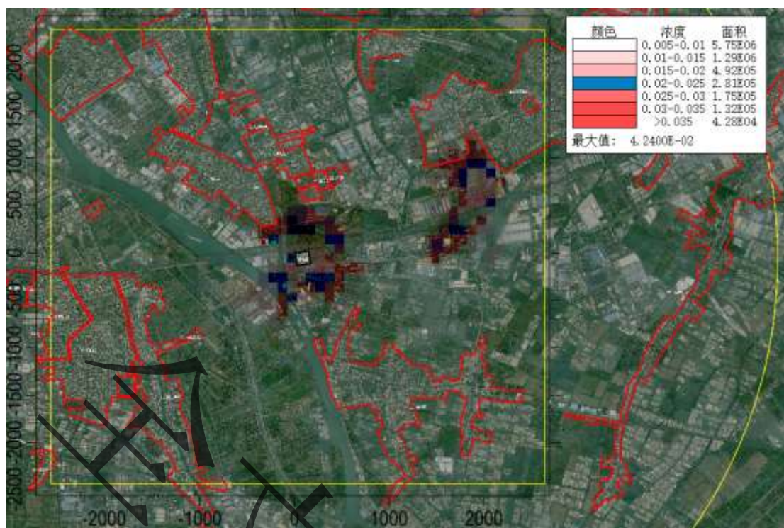
图 6.3-24 项目污染源氯化氢最高贡献浓度预测结果-小时均值-叠加值
