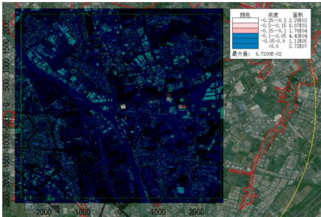
图 6.3-28 项目污染源 TSP 最高贡献浓度预测结果-年均值-叠加值
