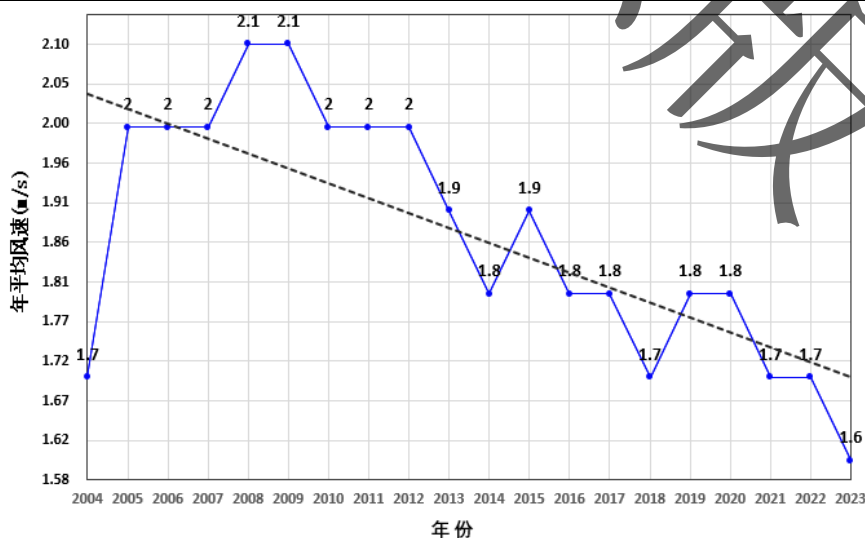
图 6.3-3 中山市 2004-2023 年累年月平均风速统计
