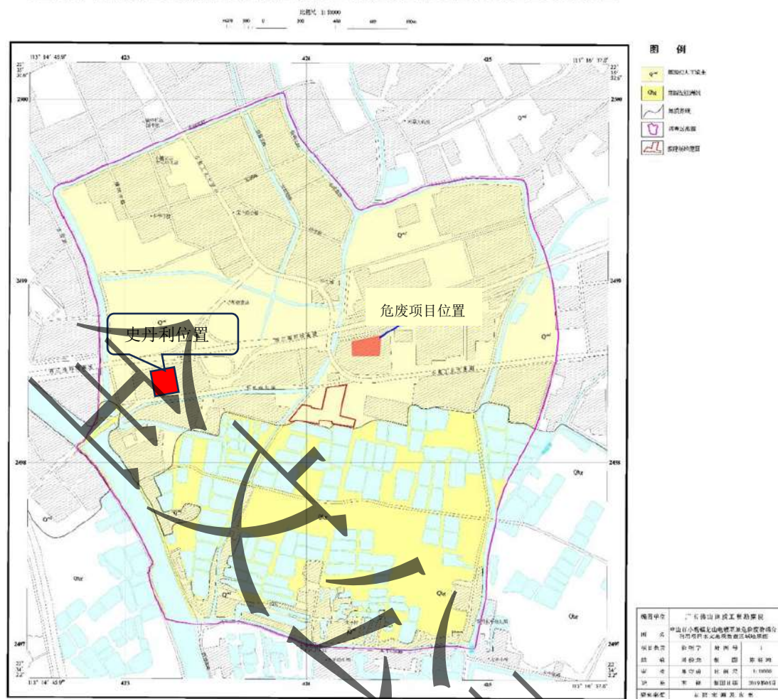
中山市小榄镇龙山电镀基地危险废物综合利用项目水文地质勘查区域地质图
