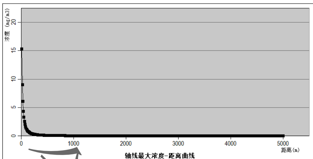
图 6.7-6 氨水泄漏事故最大浓度-距离曲线图
