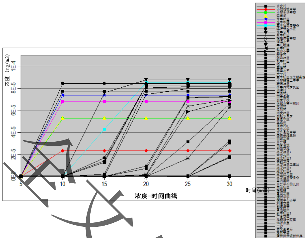
图 6.7-13 CO事故各关心点浓度随时间的变化曲线图
