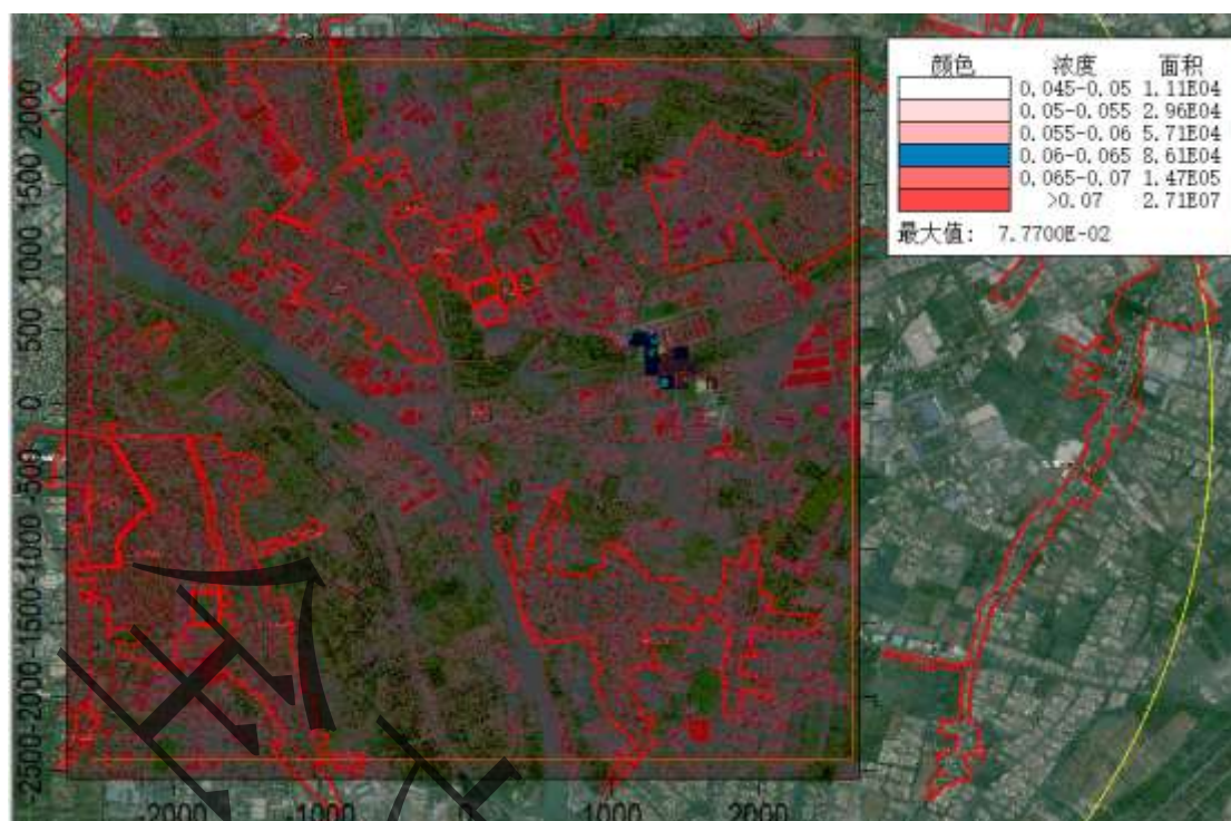
图 6.3-22 项目污染源 PM 2.5 最高贡献浓度预测结果-日均值-叠加值
