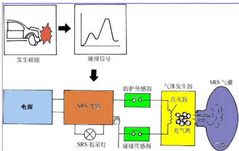
图 2 安全气囊引爆过程图
