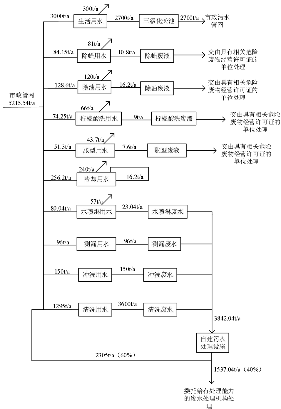
水平衡图:
