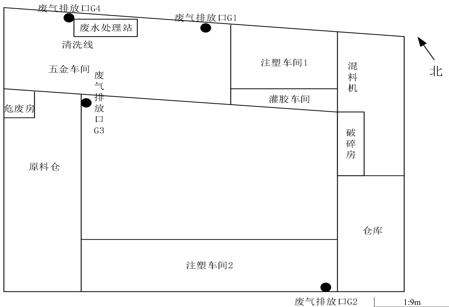
附图一 建设项目 1 楼平面布置图
