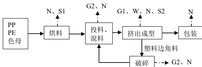
图 2-3 项目卷芯管生产工艺流程及产污环节图
