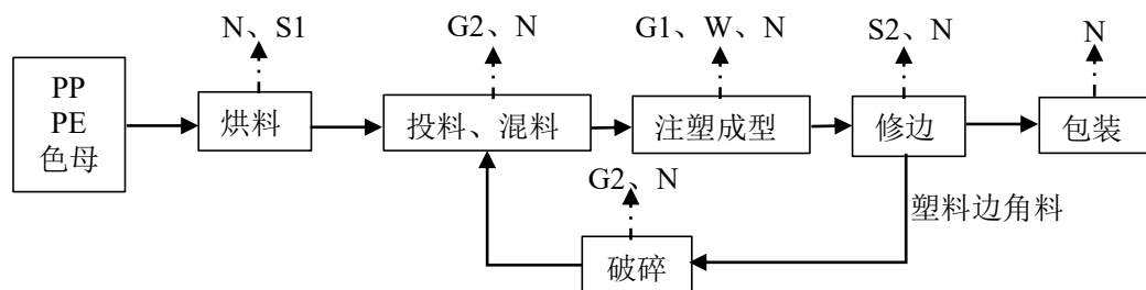
图 2-2 项目灯饰外壳、堵头生产工艺流程及产污环节图
