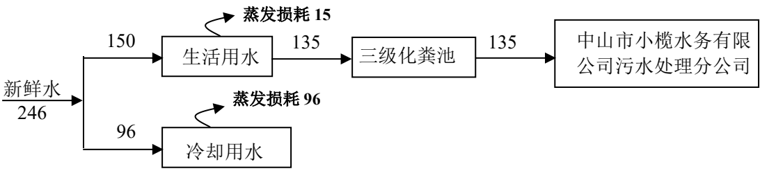
图 2-1 本项目水平衡图 （单位：吨/年）
