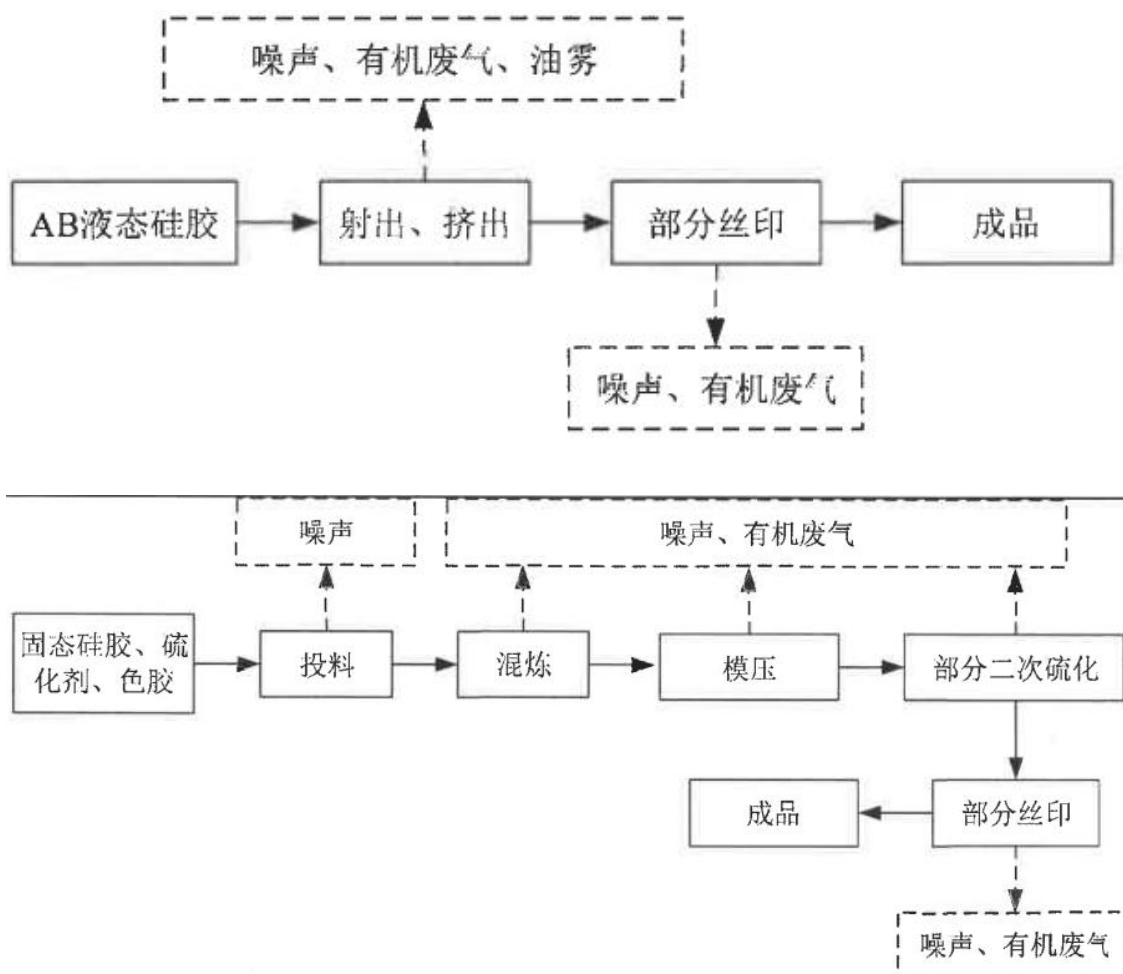
图 1 硅胶制品生产工艺流程图及产污环节图
