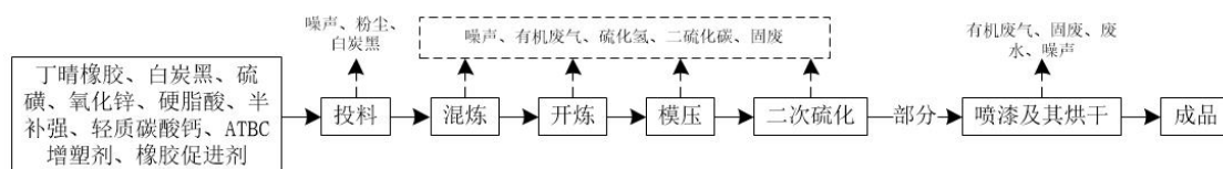
图 2 橡胶制品生产工艺流程图及产污环节图
