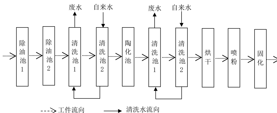
图 2-1 自动表面处理线流程图
