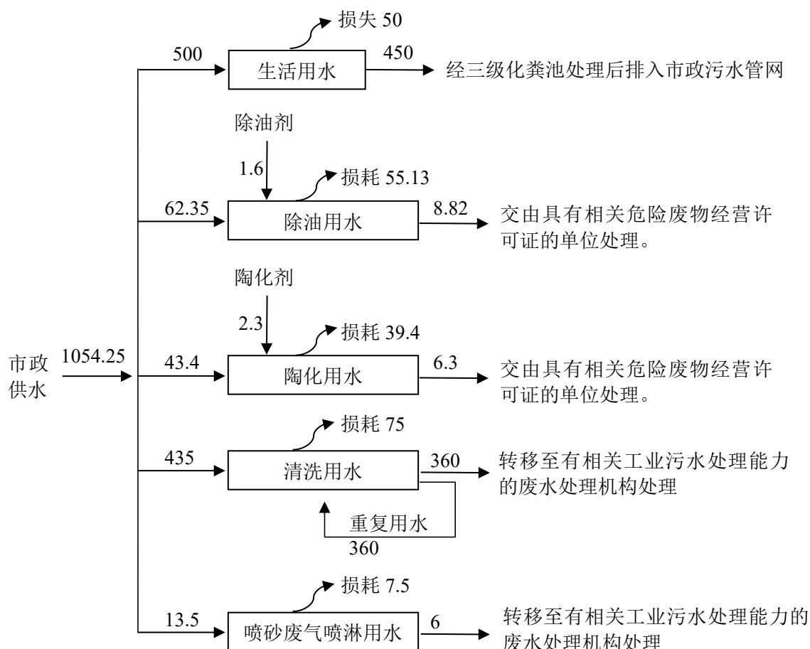
图 2-2 搬迁项目水平衡图 (m³/a)
