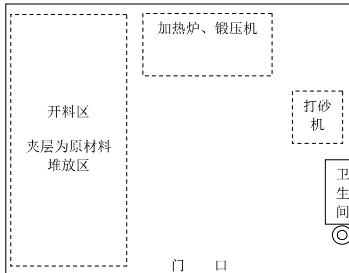
项目 1F 平面布置图
