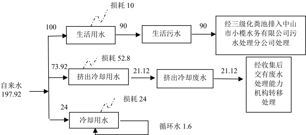
图 1 全厂水平衡图（单位：t/a）
