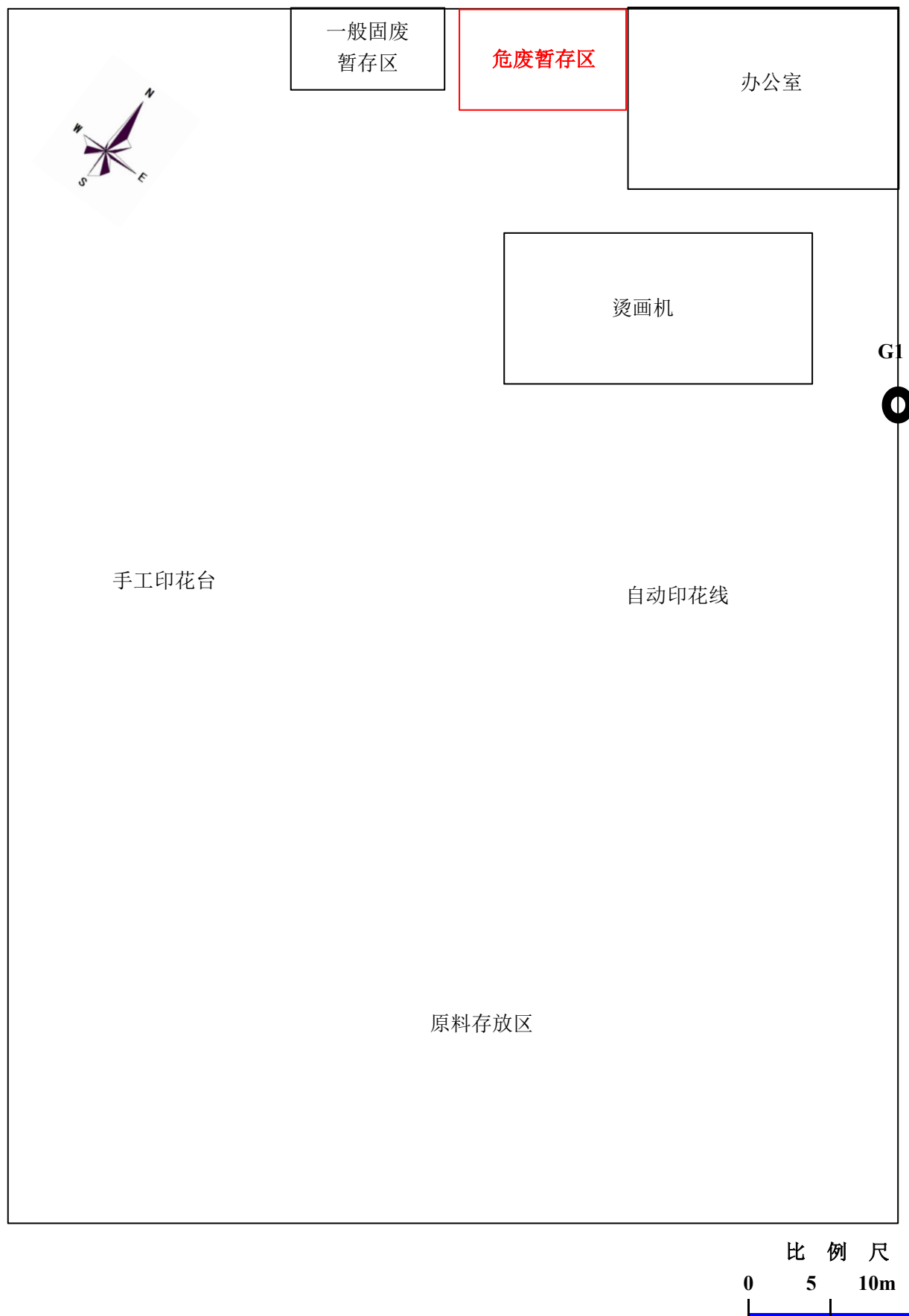
图 3-2 项目平面布置图 (B 车间一层)
