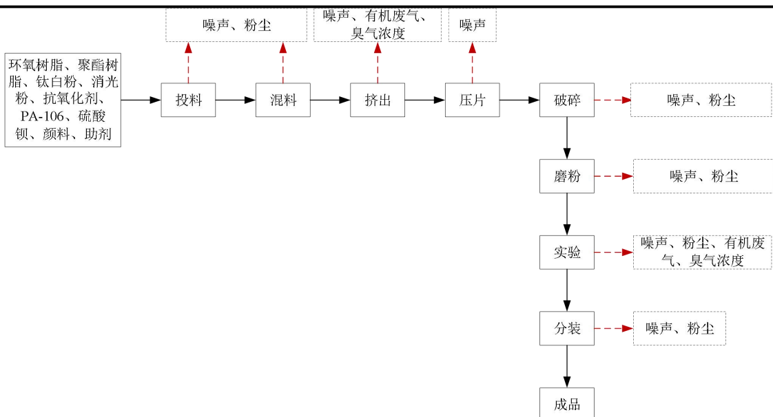
图3 生产工艺流程图及产污环节
