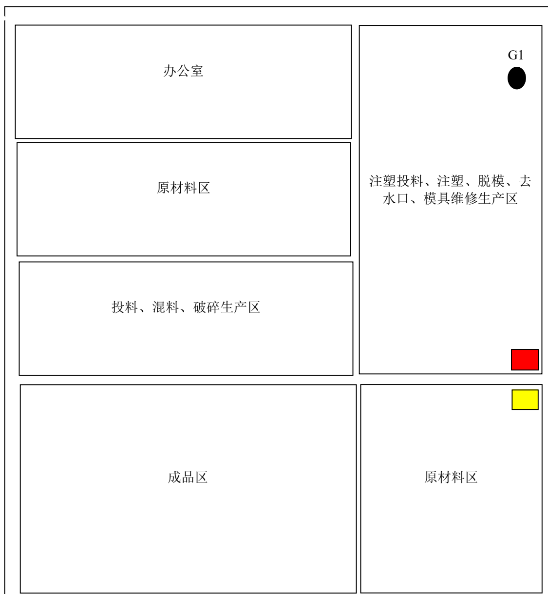
图 3 厂房平面布局图
