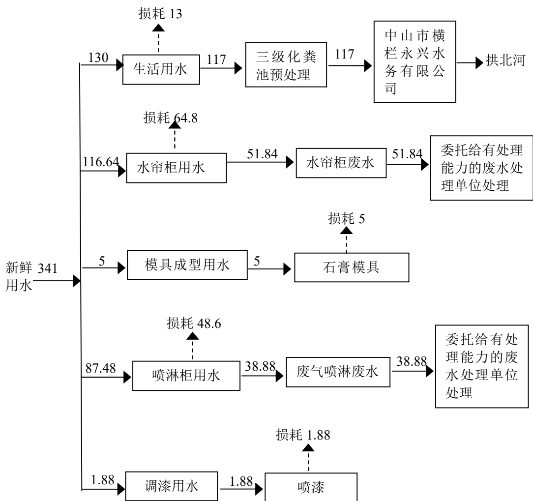
图 1 项目水平衡图 (t/a)
