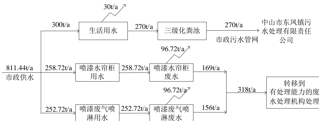
附图 1 水平衡图
