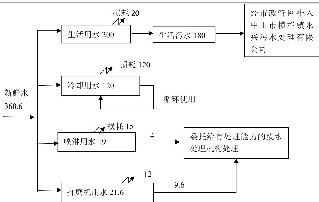
图 1 全厂水平衡图（单位：t/a）
