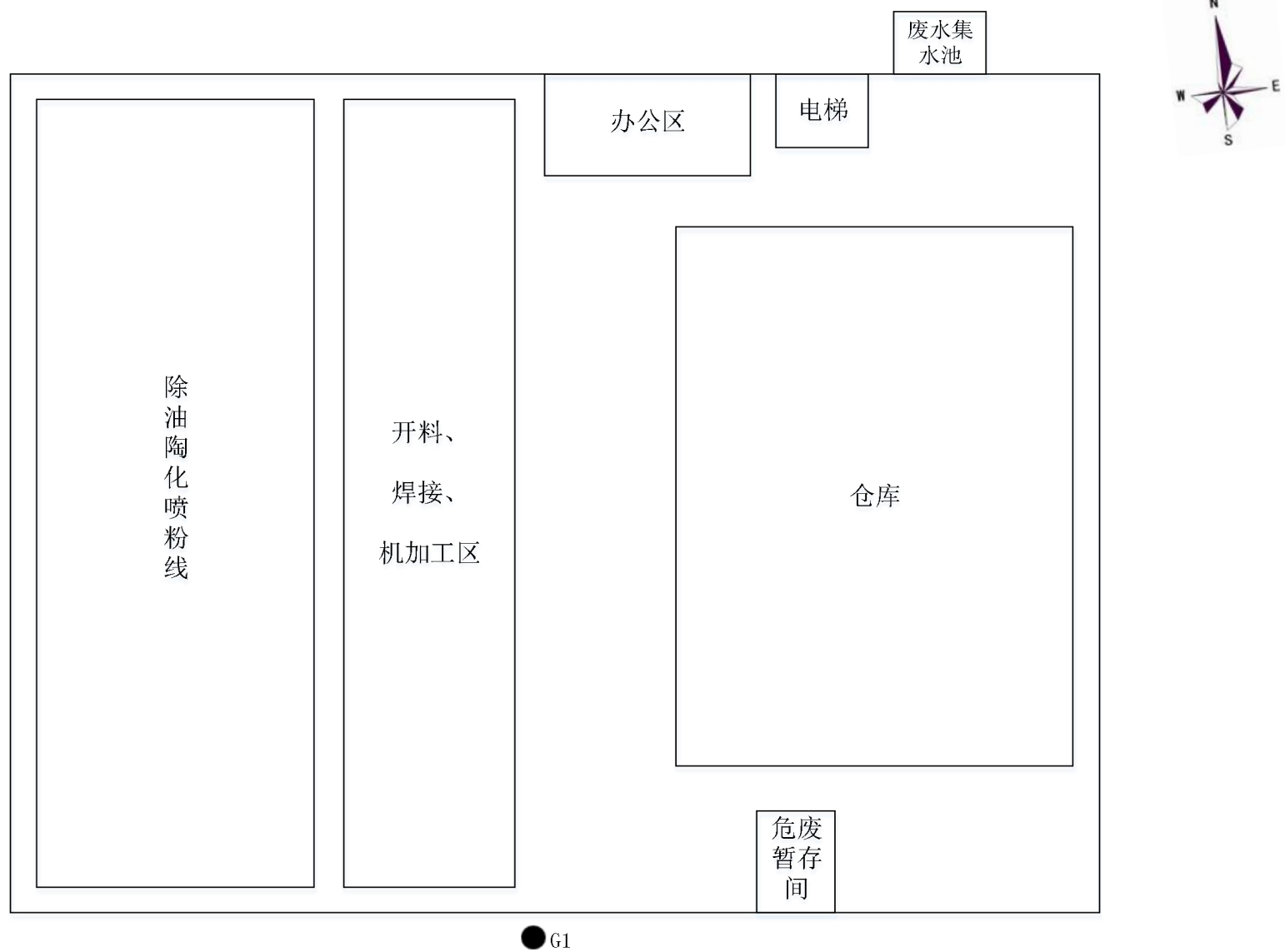
附图 3 建设项目平面图
