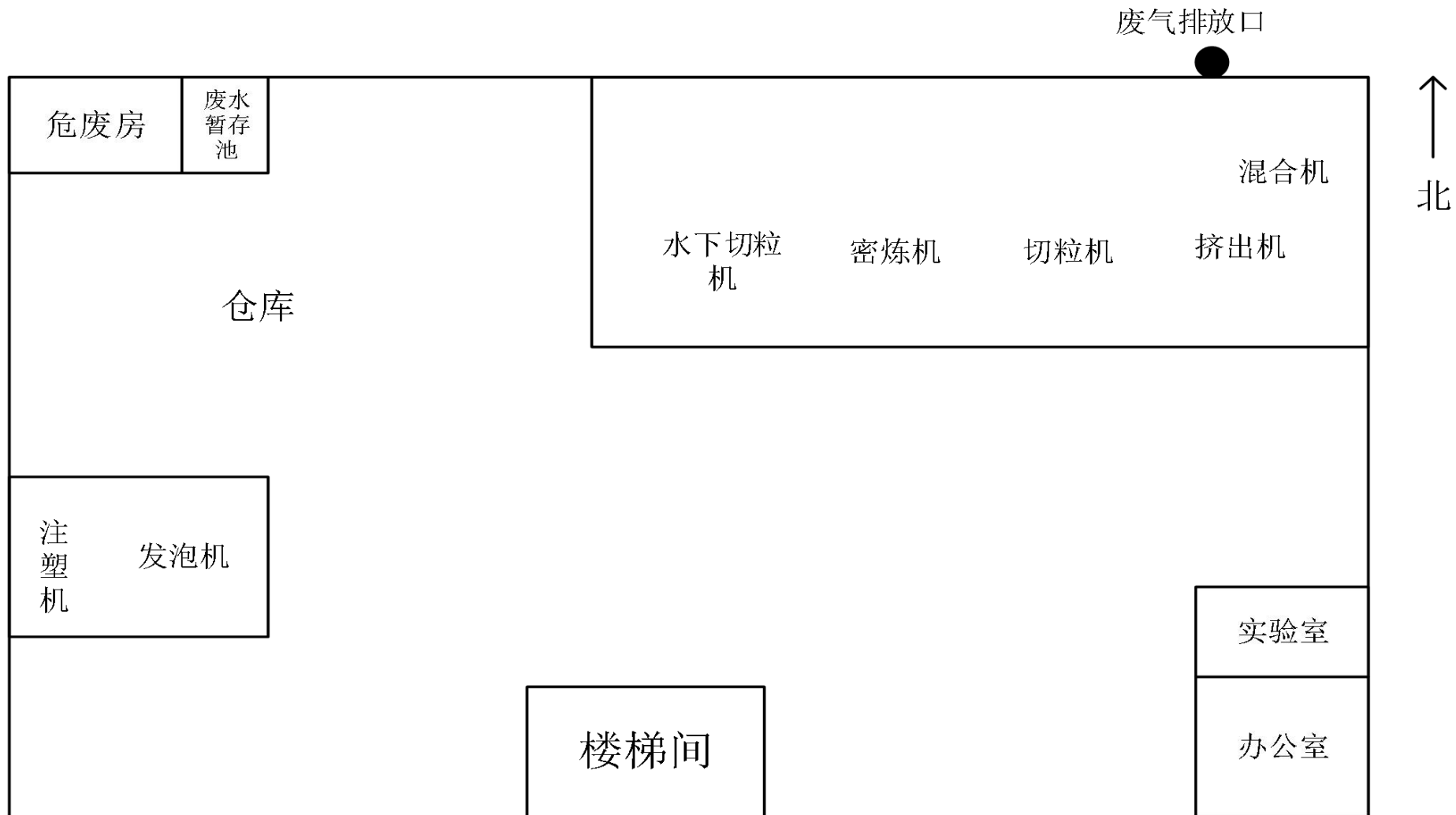
图三 建设项目 1 楼平面布置图
