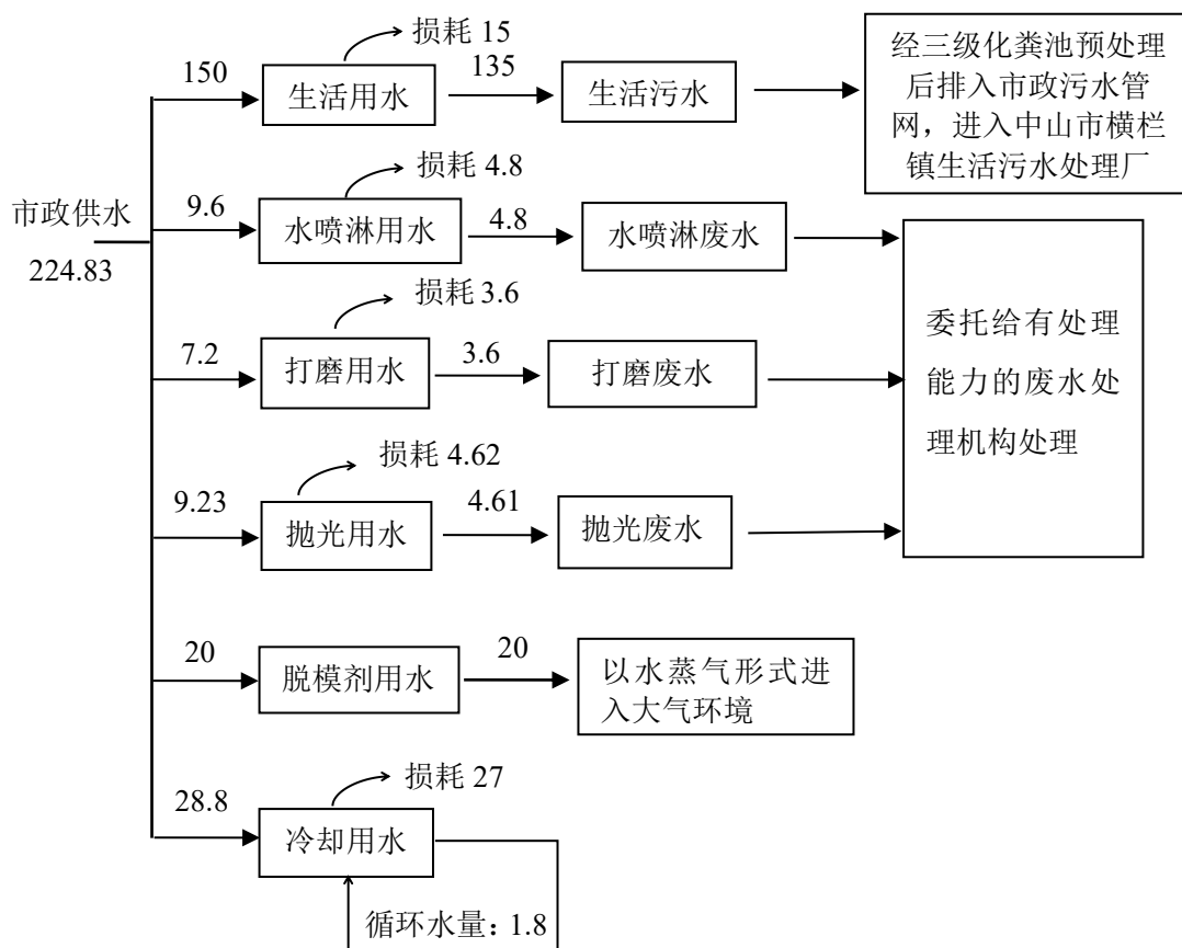
图 1 水平衡图 (单位: t/a)
