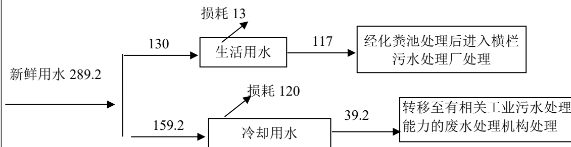
图 2-1 项目水平衡图 (m³/a)
