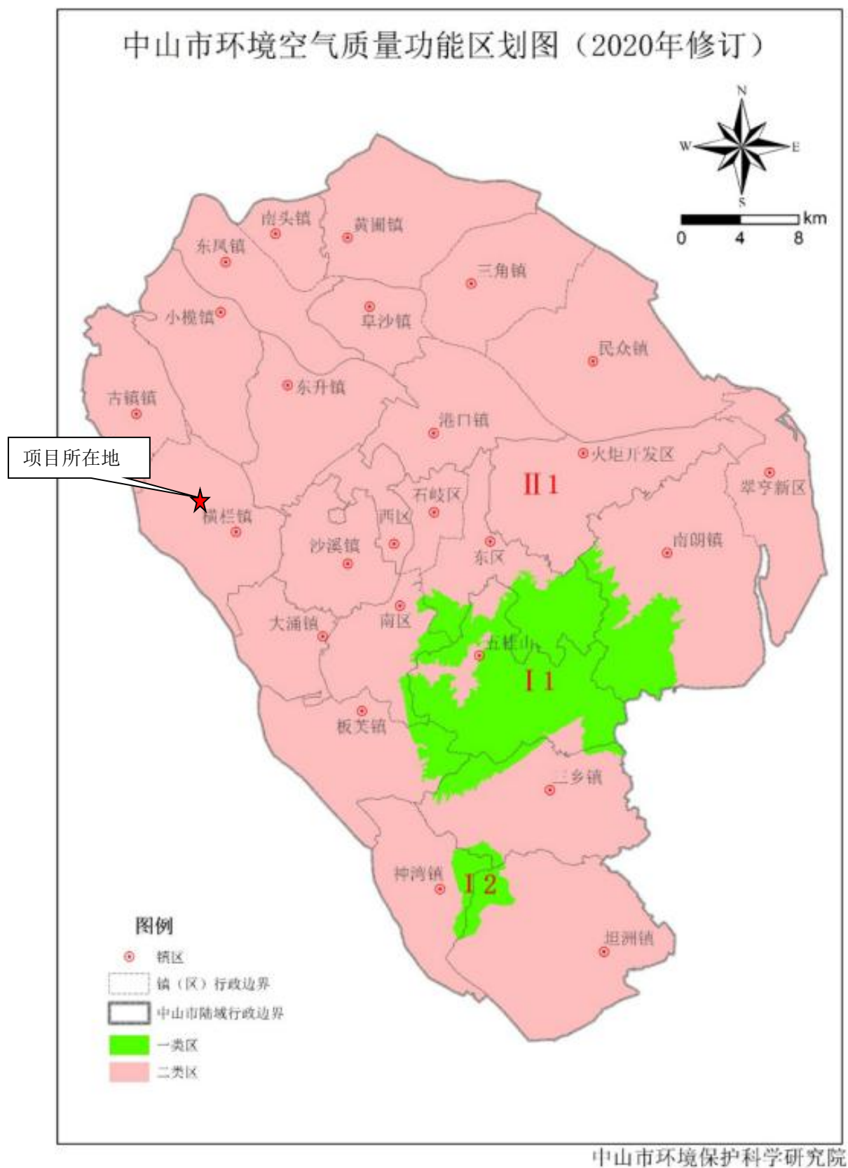
附图六：环境空气质量功能区划图
