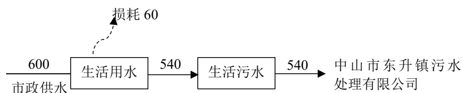
图 2-1 扩建前项目水平衡图（单位：t/a）
