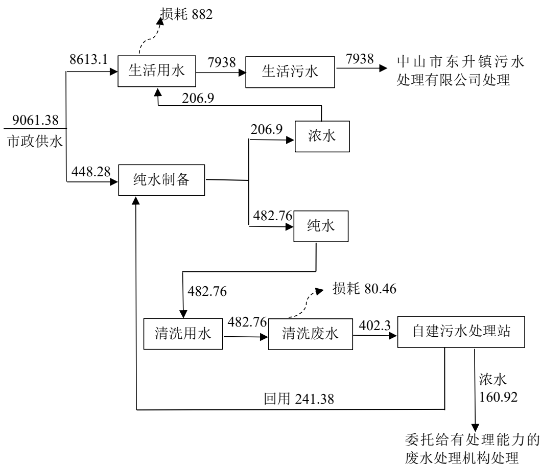
图 1-2 扩建后全厂水平衡图（单位：t/a）
