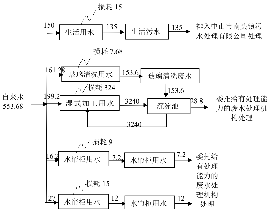
图 2 全厂水平衡图 (单位: t/a)
