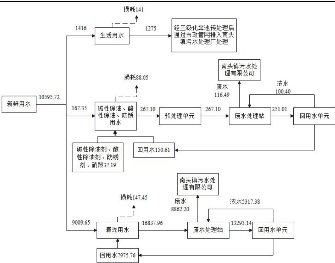
图二 项目改扩建后水平衡图 单位 t/a
