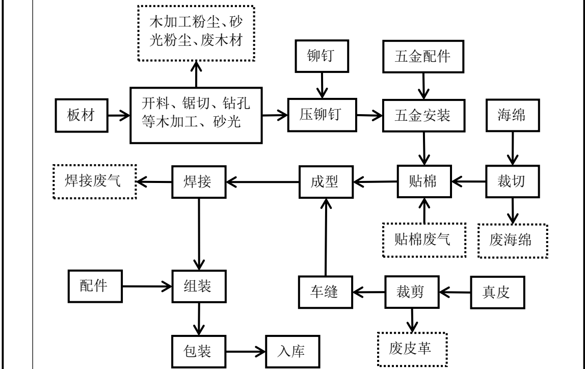
图七 座椅生产工艺流程图
