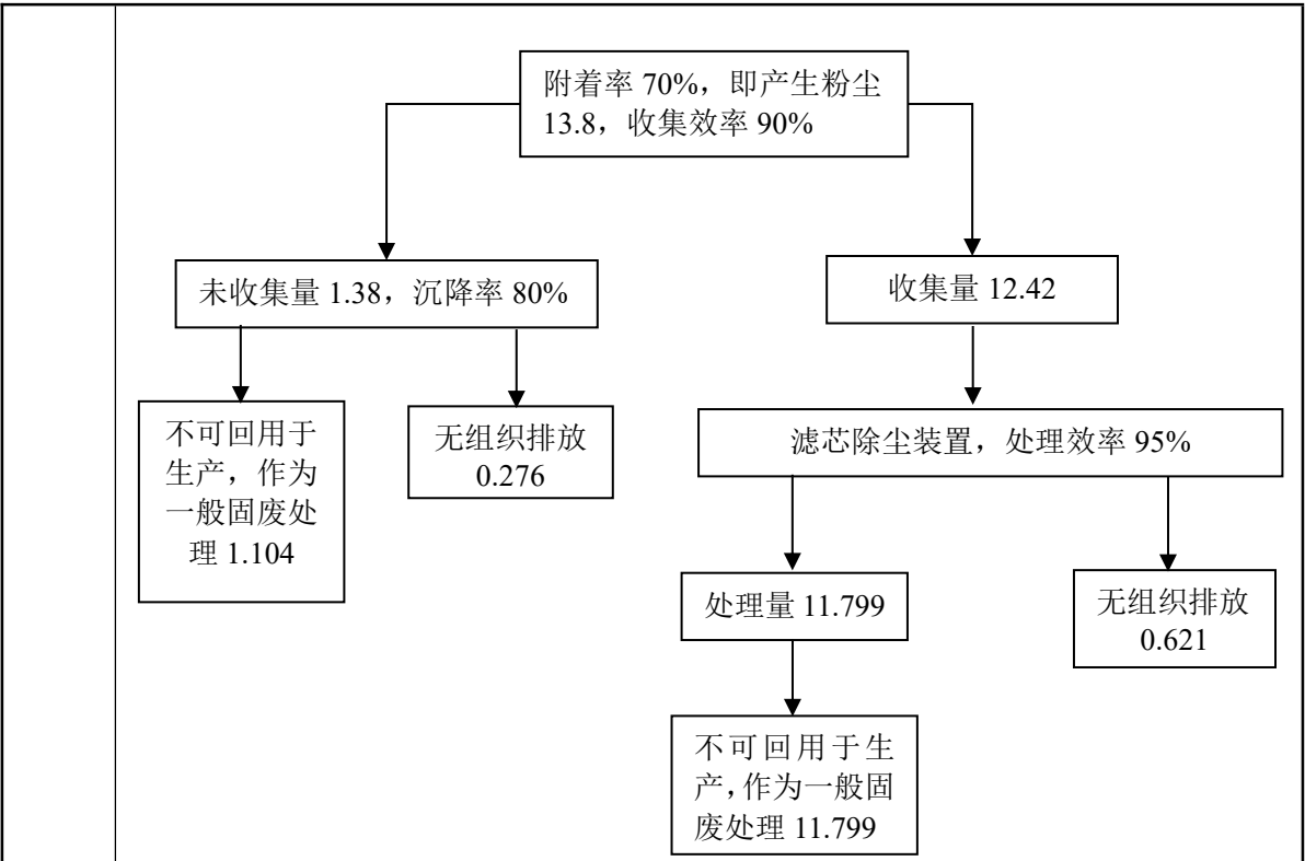
图 喷粉产生颗粒物物料平衡图（t/a）
