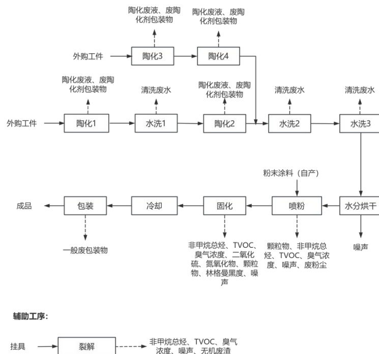
图4 喷涂工件生产工艺流程图
