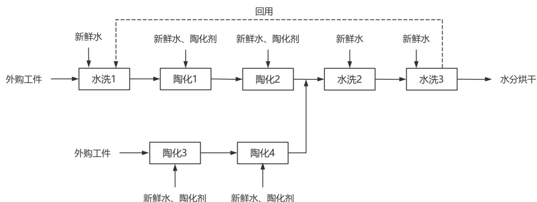
图 1 工件前处理槽体示意图
