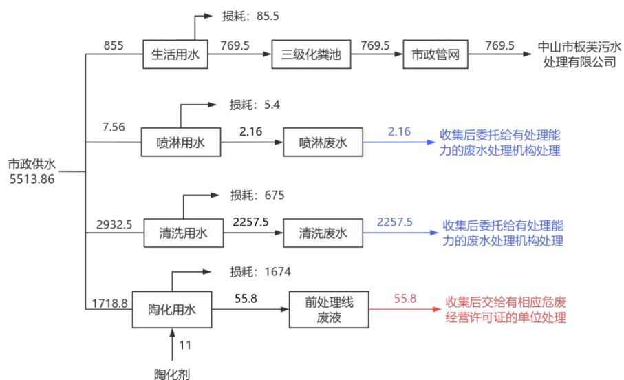
图2 水平衡图 (t/a)
