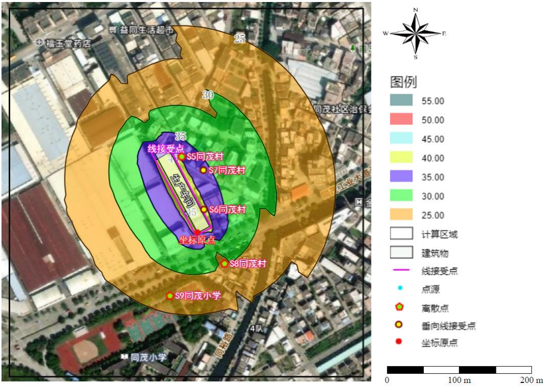
图 6.3-2 改扩建完成后项目噪声贡献值等声线图（夜间）
