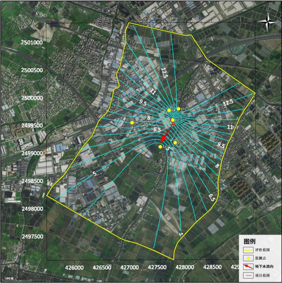
图 6.5-3 地下水流向图
