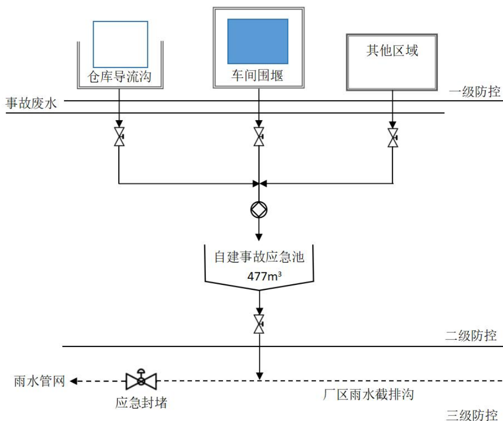
图 7.4-2 企业环境风险三级防控体系示意图
