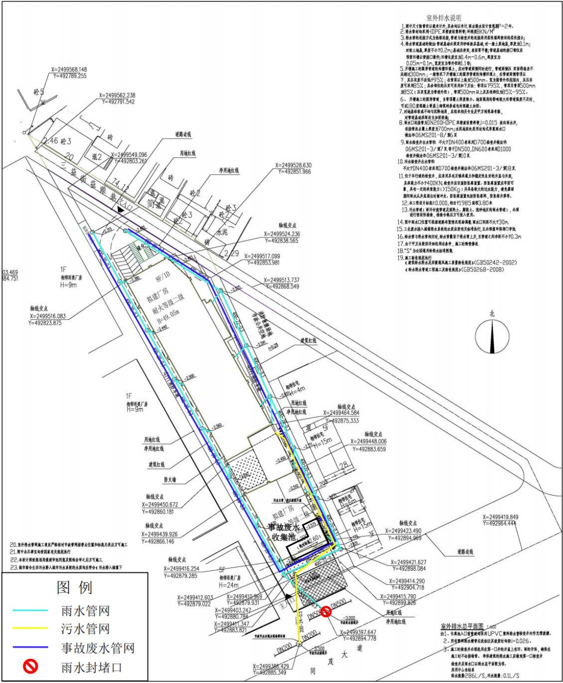
图 7.4-3 项目雨污管网和事故废水管网图
