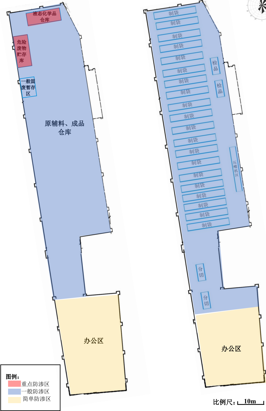
图 8.5-2 改扩建完成后项目地下水污染防渗分区图（5F 和 6F）
