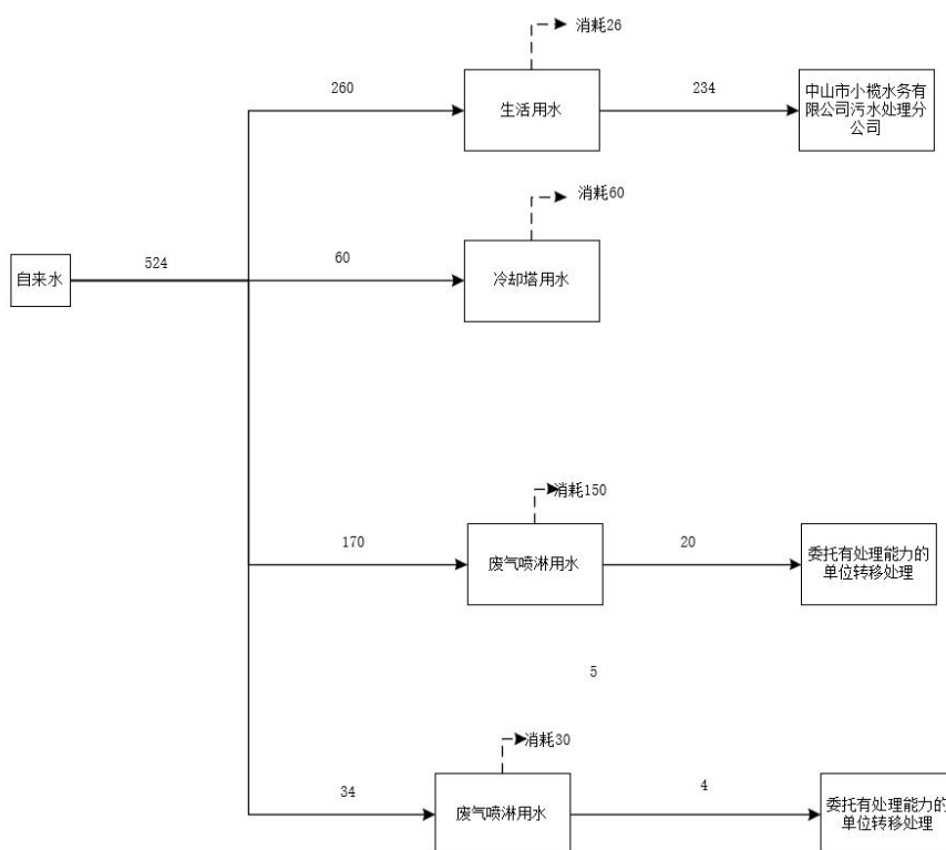
图 2-1 项目水平衡情况图 (m³/a)
