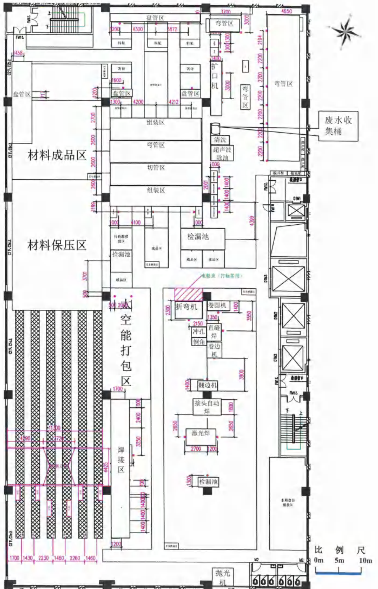
附图 2-2 项目 2F 平面布置示意图
