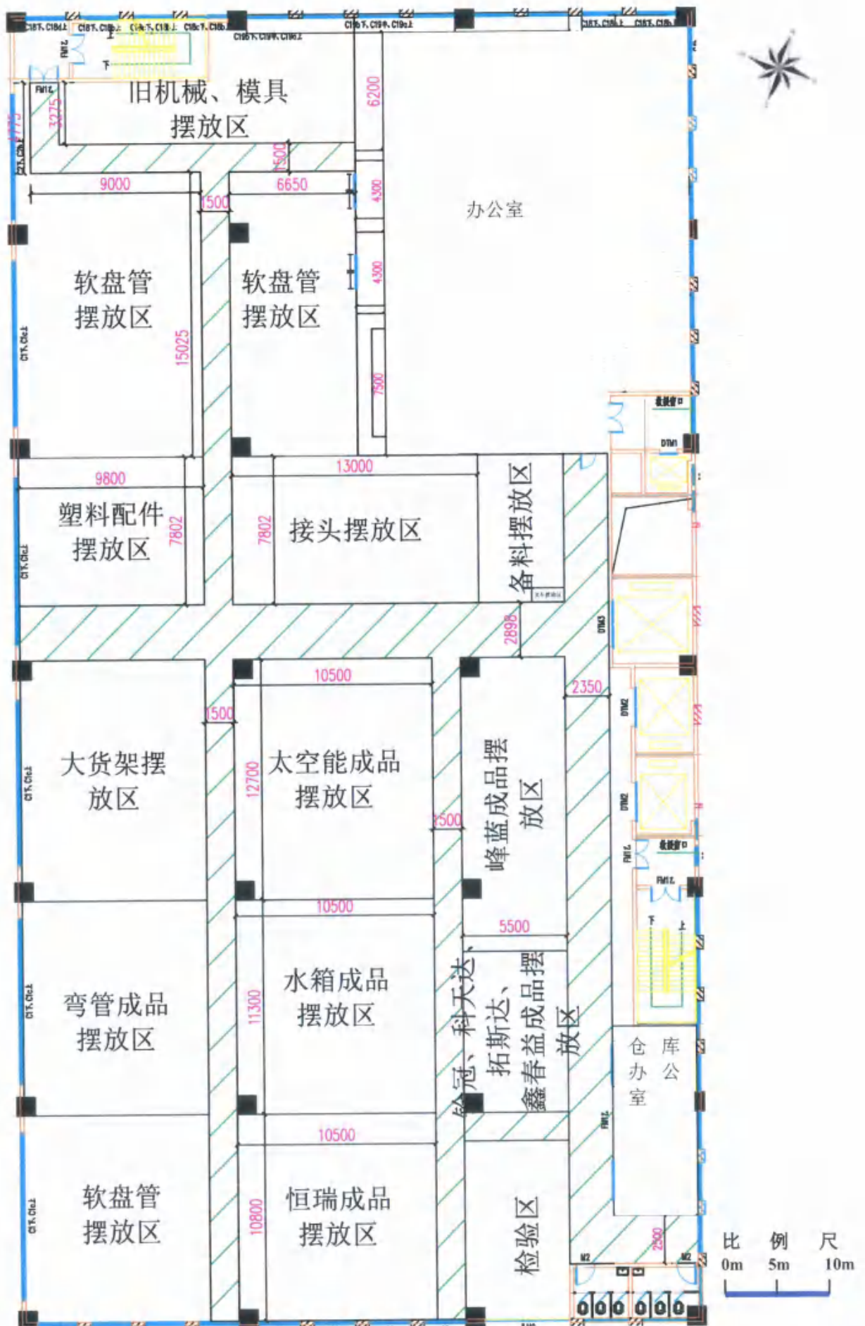
附图 2-3 项目 3F 平面布置示意图
