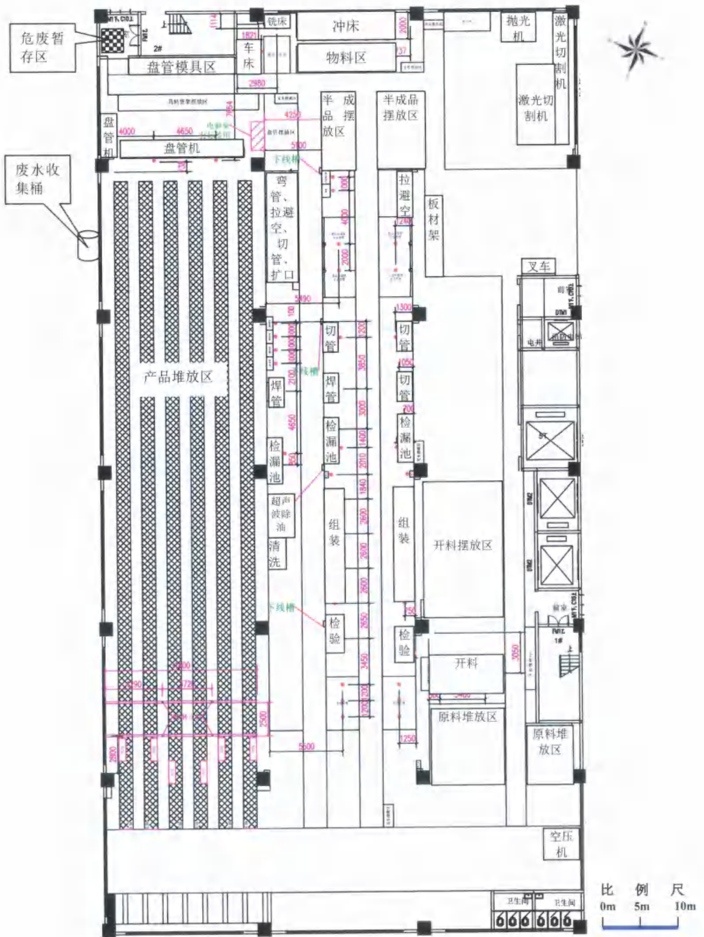
附图 2-1 项目 1F 平面布置示意图
