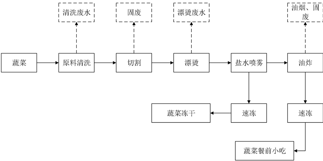
图 4 蔬菜制品工艺流程及产污环节图
