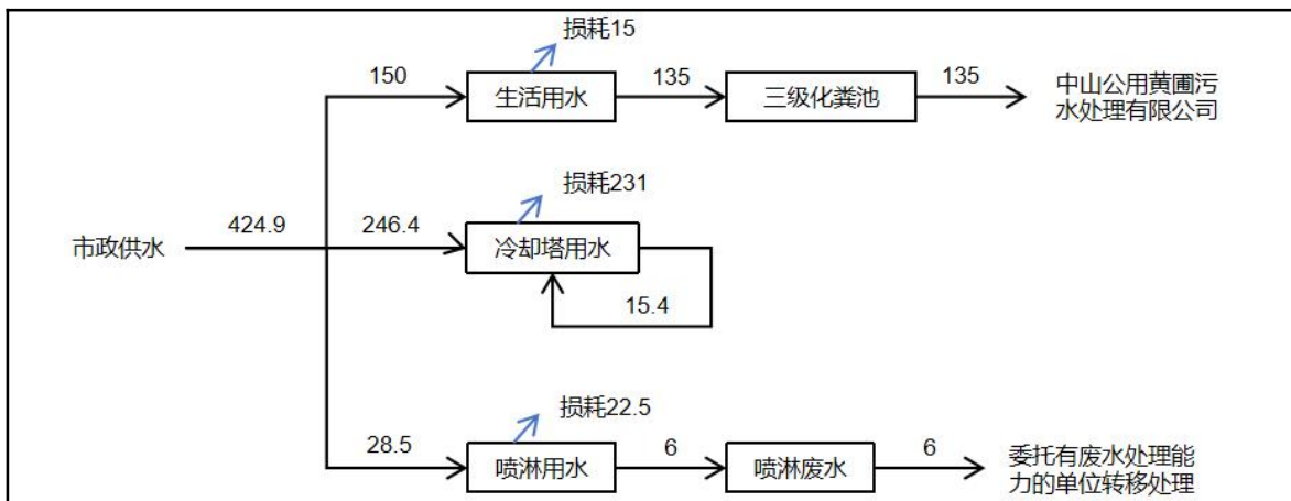
图 2 全厂水平衡图（单位：t/a）
