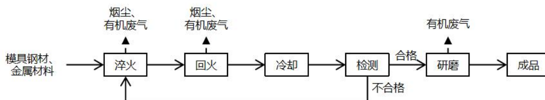
图 3 模具钢材、金属材料生产工艺流程图
