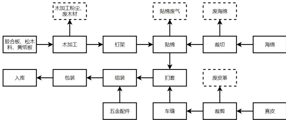
图八 沙发生产工艺流程图
