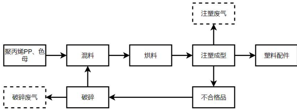
图九 塑料配件生产工艺流程图
