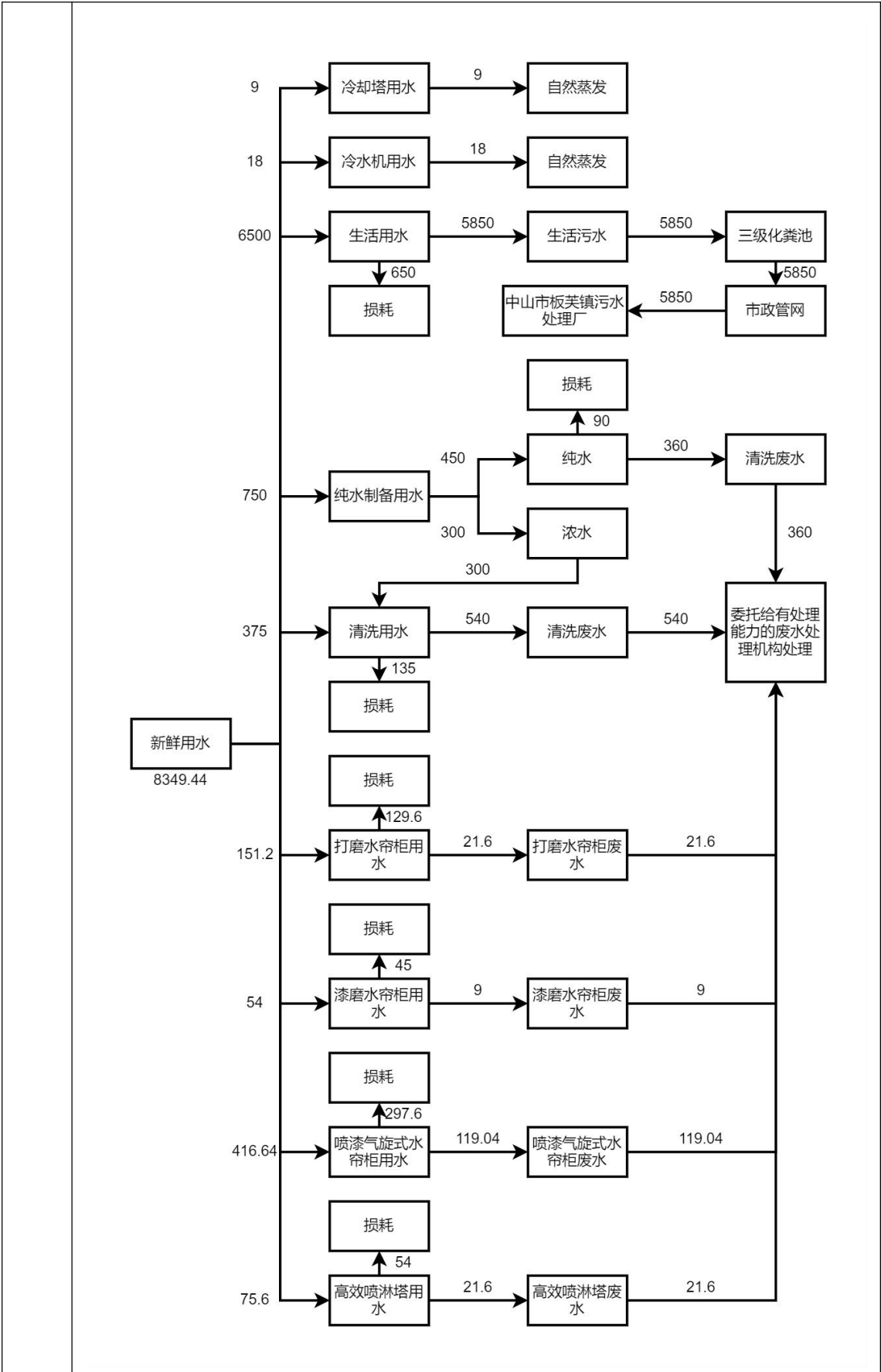
图一 原有项目水量平衡图 (t/a)
