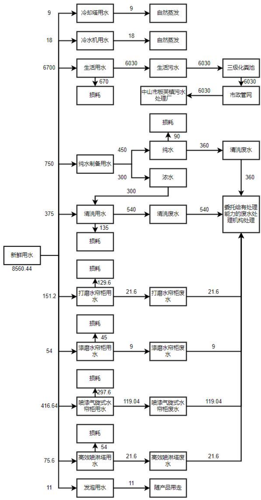
图三 扩建后项目水量平衡图 (t/a)
