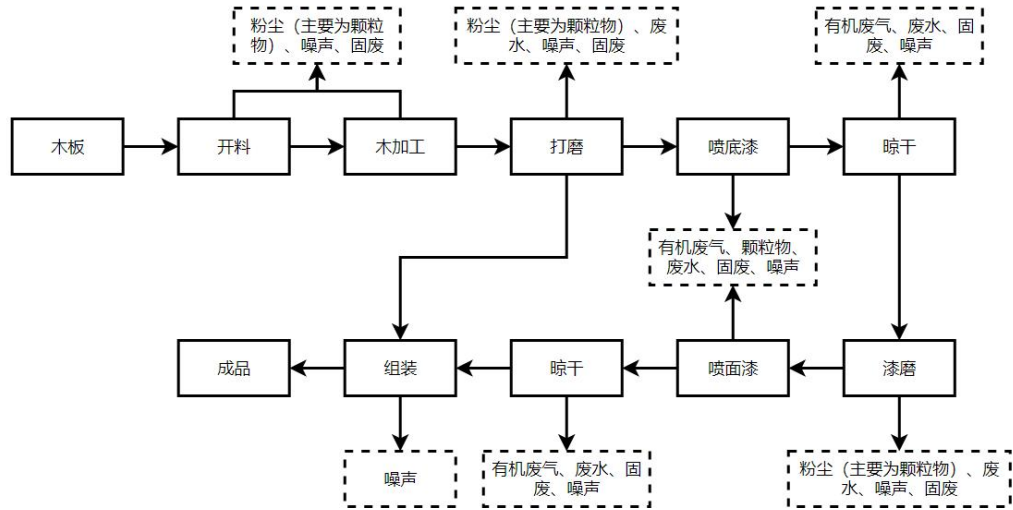
图十二 斗柜、衣柜生产工艺流程图
