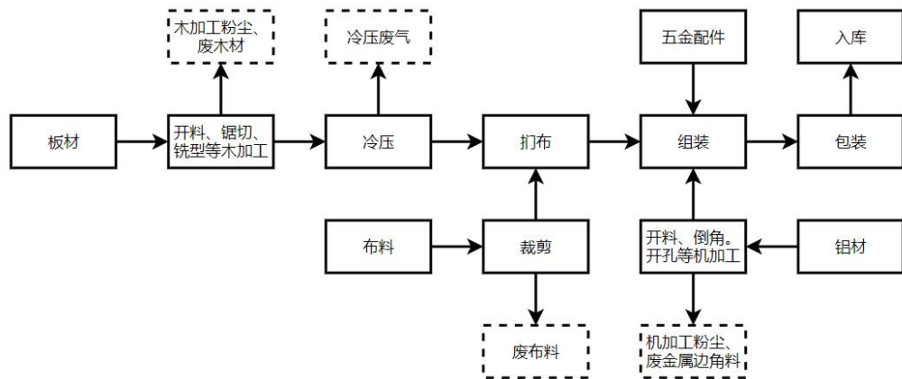
图六 屏风生产工艺流程图
