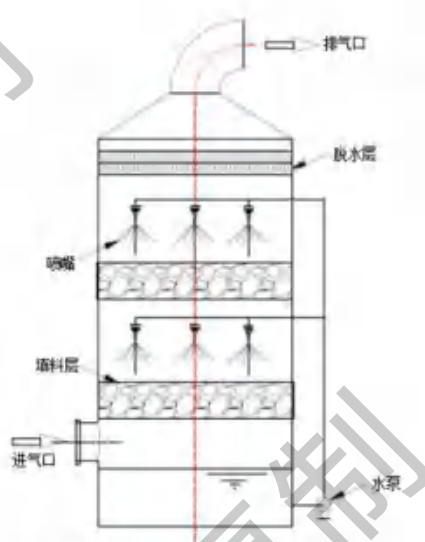
图 6.2-2 酸雾废气喷淋塔示意图
