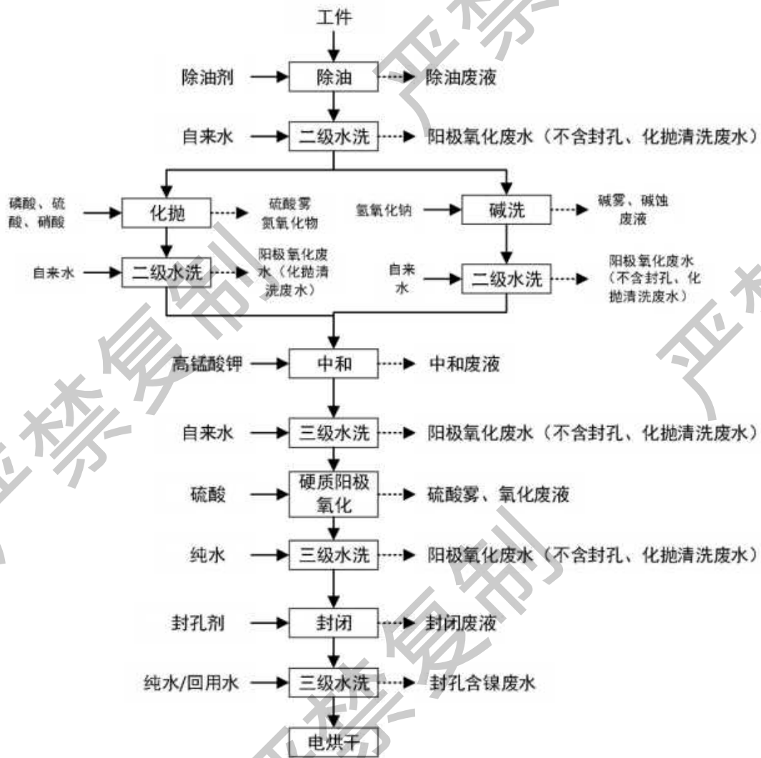
图 3.2-9 自动阳极氧化线 8#生产工艺流程图
