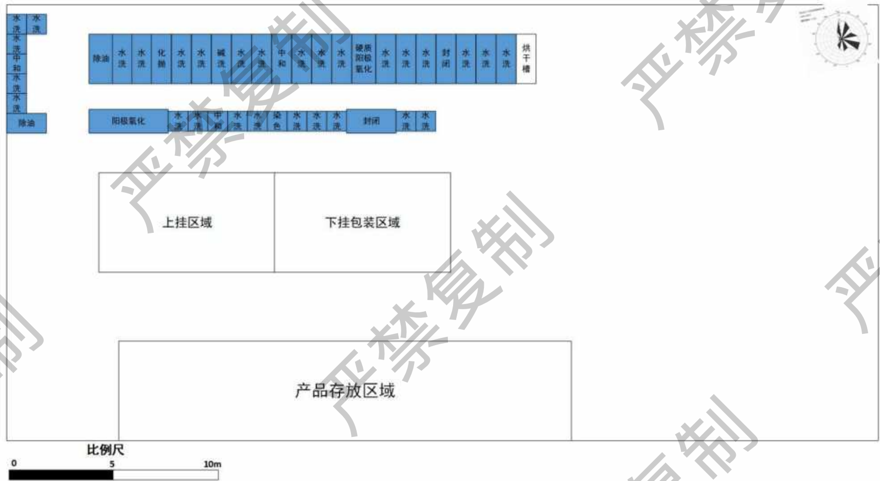
图 3.1-13 槽体平面布置图—自动阳极氧化线 8#、手动阳极氧化线 9#
