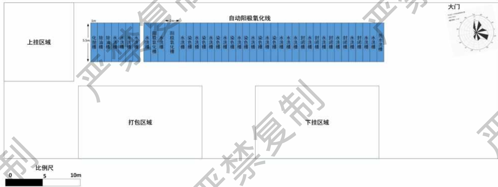
图 3.1-6 槽体平面布置图—自动阳极氧化线 1#
