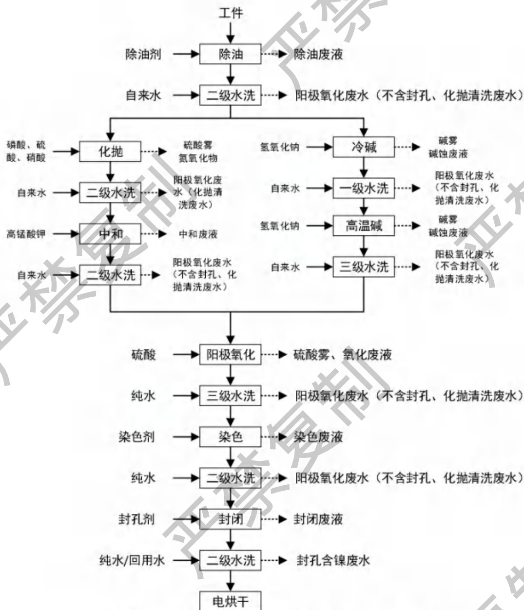
图 3.2-11 半自动阳极氧化线 10#生产工艺流程图
