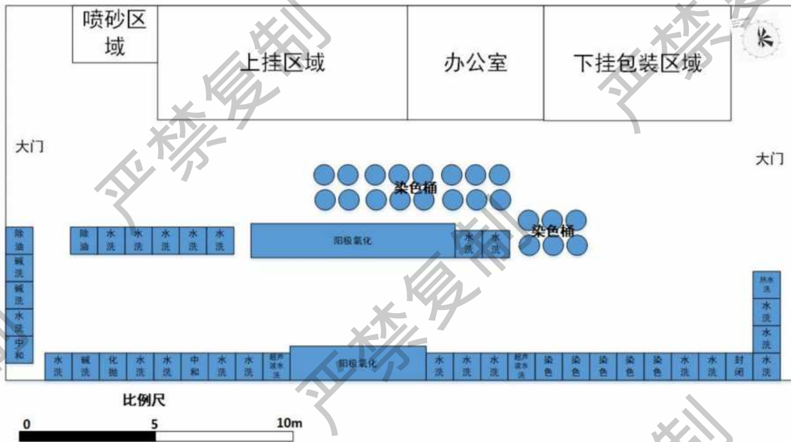
图 3.1-8 槽体平面布置图—手动阳极氧化线 3#
