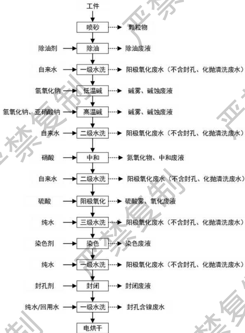
图 3.2-8 半自动阳极氧化线 7#生产工艺流程图
