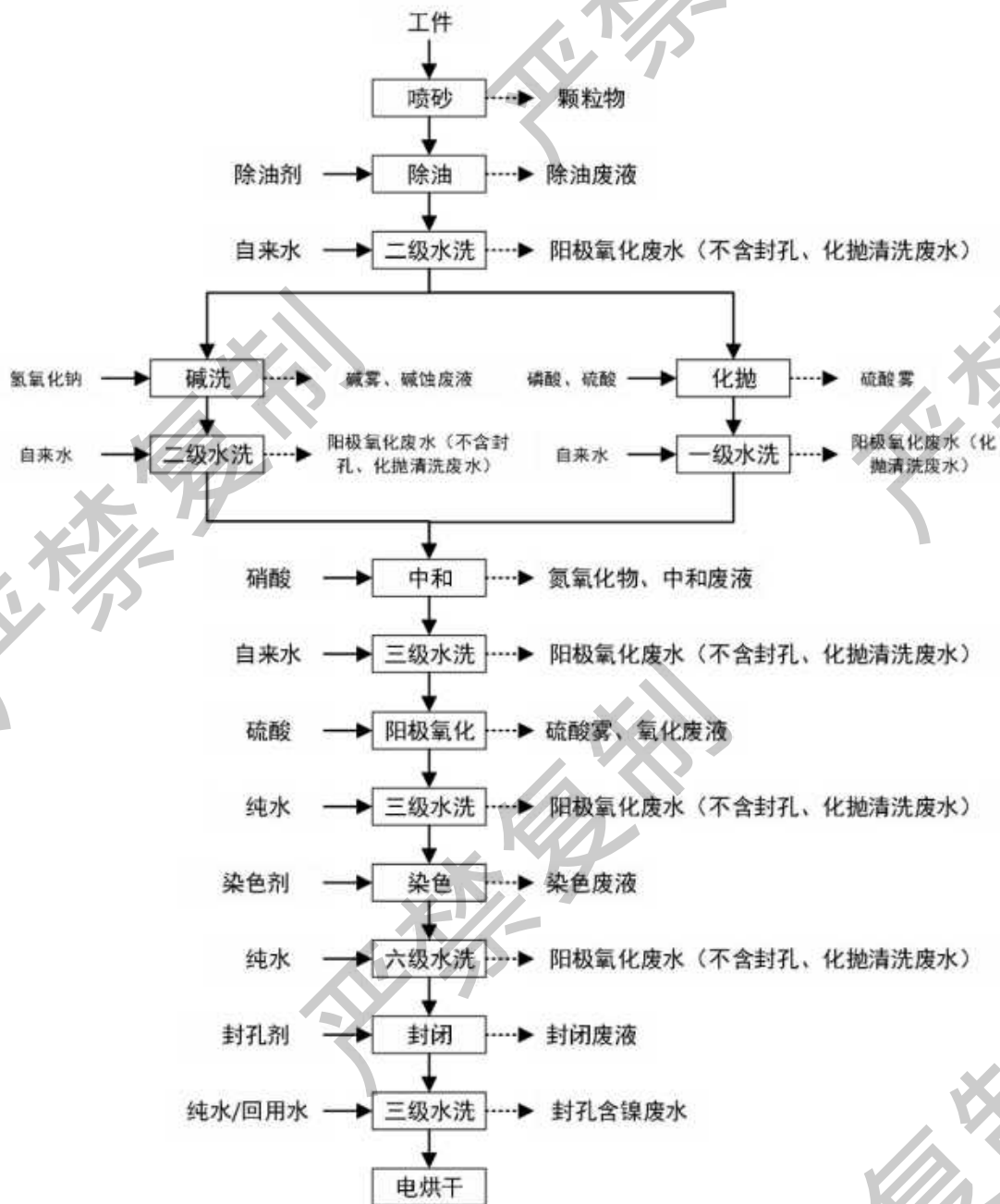
图 3.2-5 手动阳极氧化线 4#生产工艺流程图
