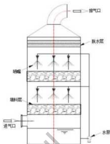
图 6.2-4 碱雾废气喷淋塔示意图
