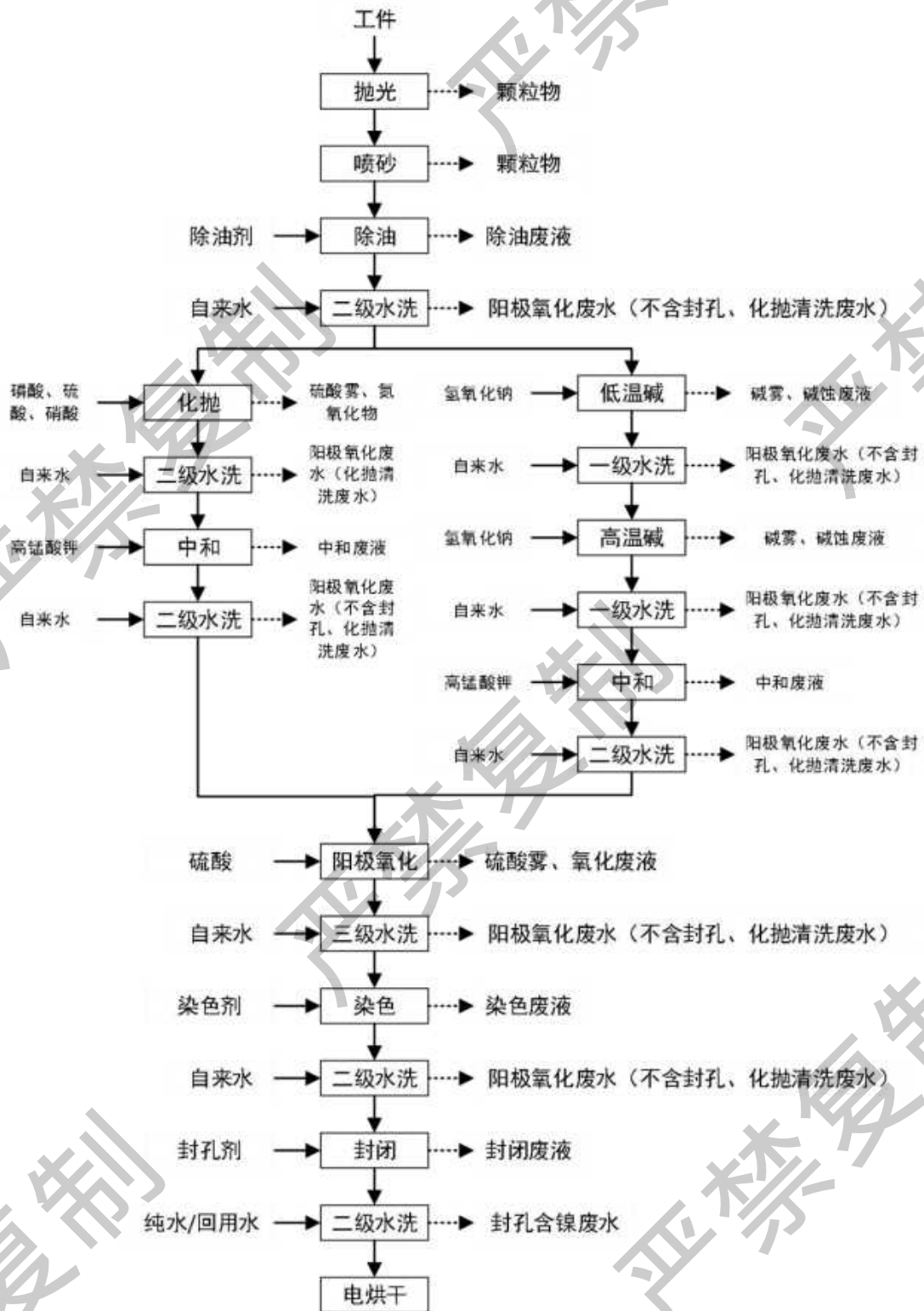
图 3.2-3 手动阳极氧化线 2#生产工艺流程图
