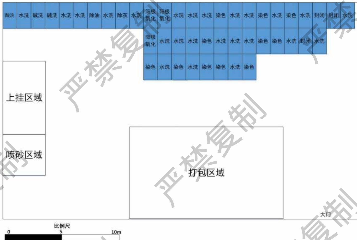
图 3.1-10 槽体平面布置图—半自动阳极氧化线 5#
