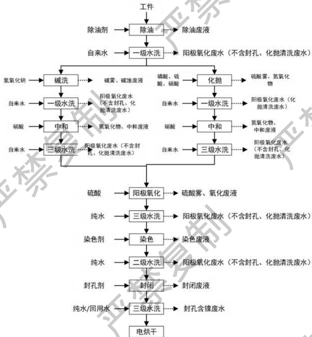
图 3.2-7 手动阳极氧化线 6#生产工艺流程图
