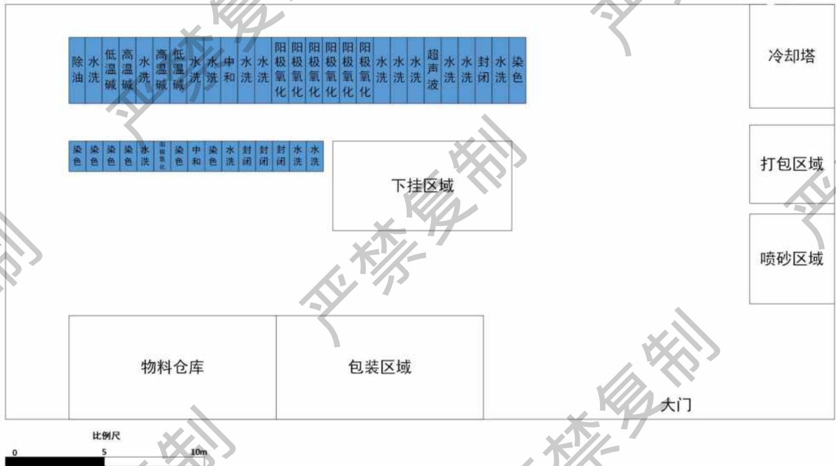
图 3.1-12 槽体平面布置图—半自动阳极氧化线 7#
