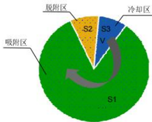
沸石转轮分子筛原理图
