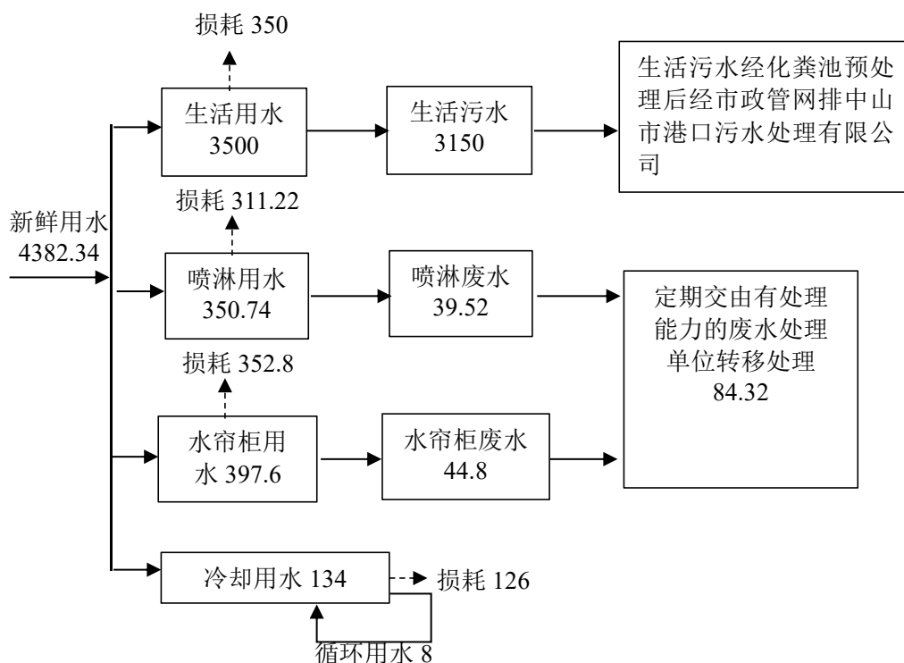
图1 水平衡图 (单位: t/a)
