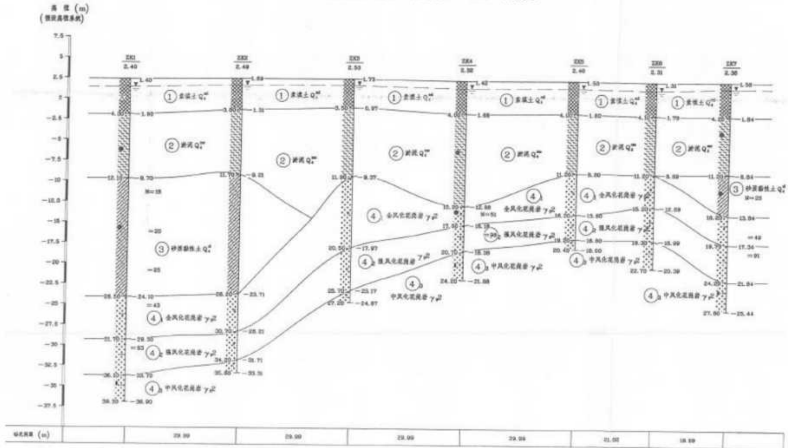
图7.3-5 项目场地水文地质剖面图
