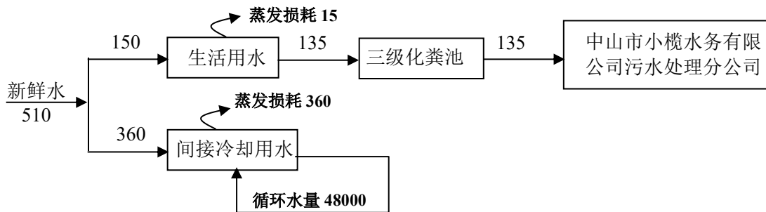
图 2-1 本项目水平衡图（单位：吨/年）
