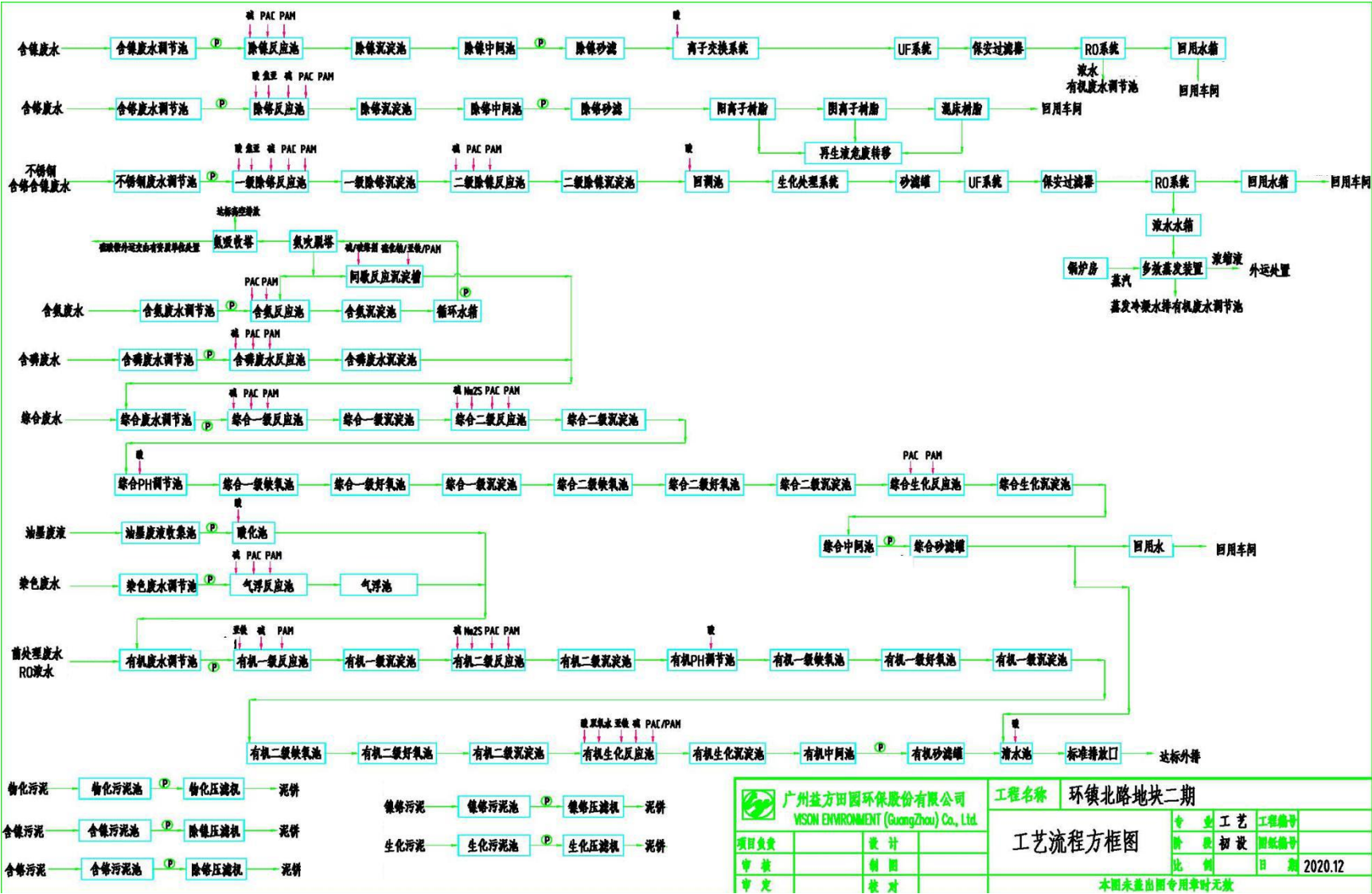
图 6.2-2 污水厂二期废水处理工艺流程图
