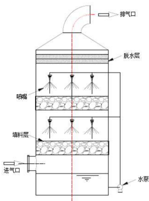
图 8.1-2 喷淋塔结构示意图
