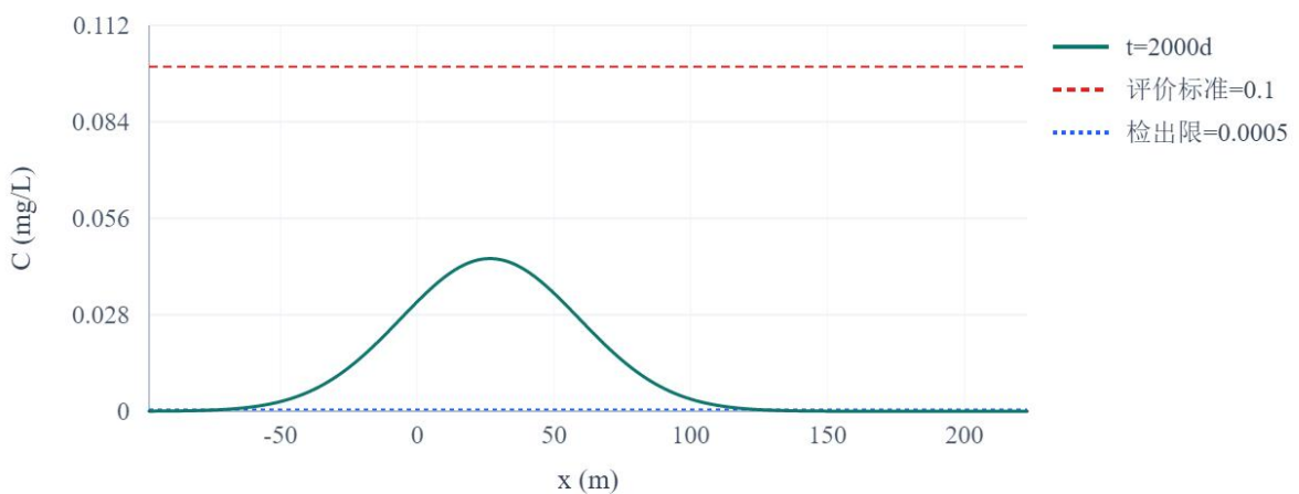
图 6.3-6 封孔槽-镍 t=2000d 地下水流向浓度变化趋势图
