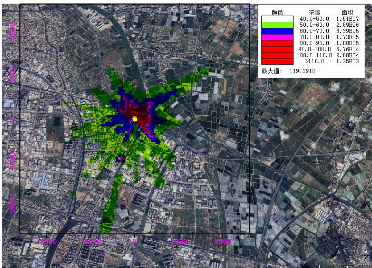
图 6.1-19 正常排放下，叠加后硫酸 1 小时平均质量浓度分布图（单位： \mu\text{g}/\text{m}^3 ）
