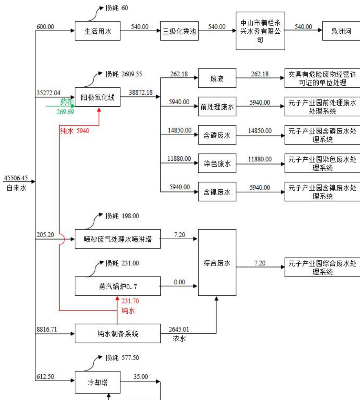
图 3.2-2 本项目年给排水平衡图 (单位 t/a)
