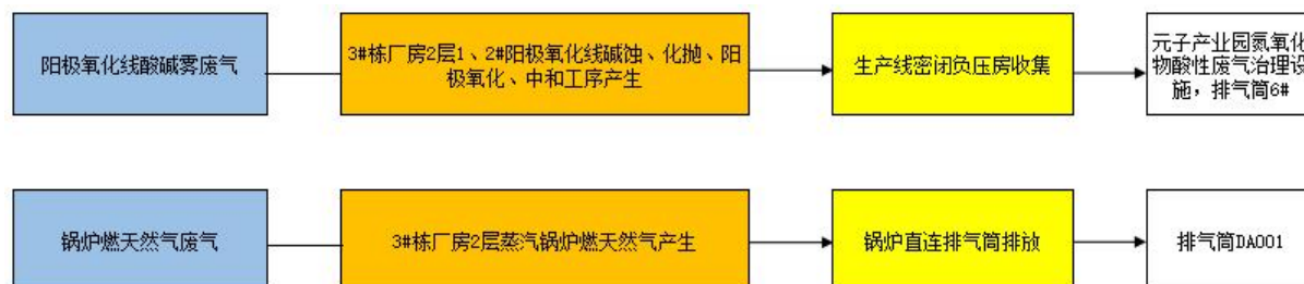
图 4.2-1 本项目有组织废气收集及治理系统示意图
