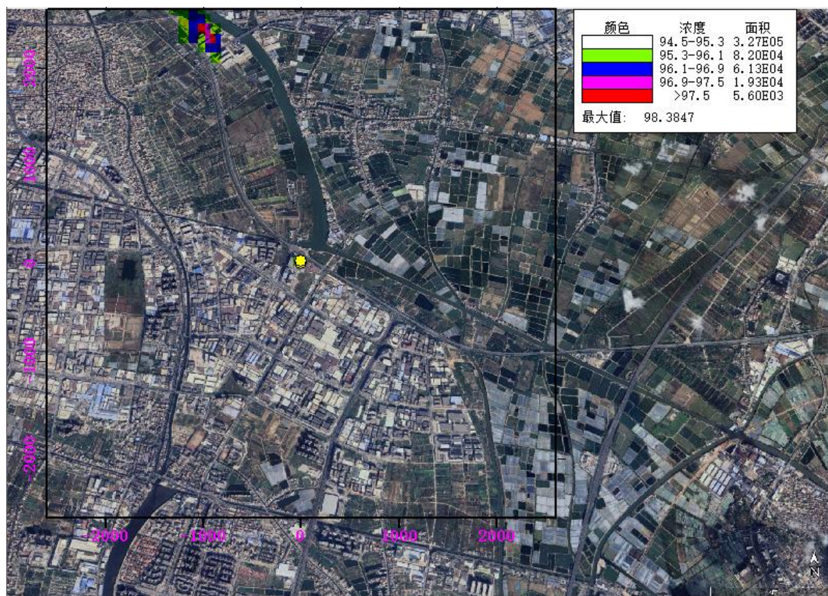
图 6.1-15 正常排放下，叠加后 PM_{10} 保证率日平均质量浓度分布图 (单位: \mu g/m^3 )
