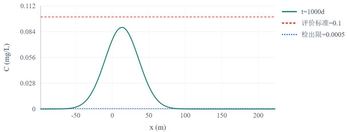
图 6.3-4 封孔槽-镍 t=1000d 地下水流向浓度变化趋势图
