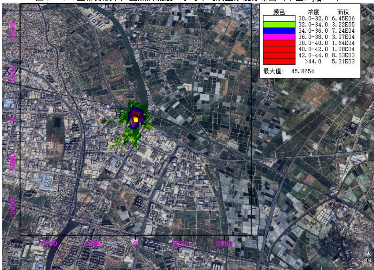
图 6.1-20 正常排放下，叠加后硫酸日平均质量浓度分布图（单位： \mu\text{g}/\text{m}^3 ）
