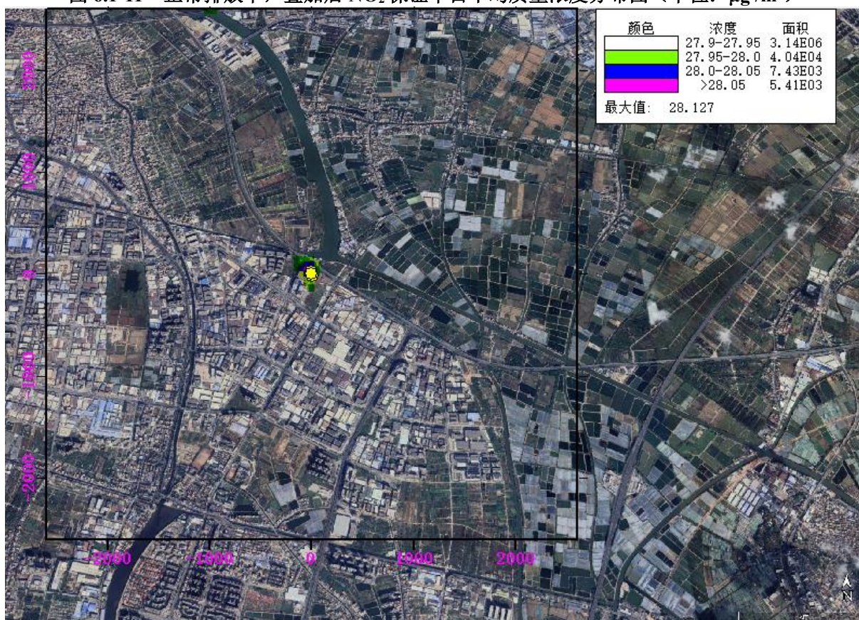
图 6.1-12 正常排放下，叠加后 NO 2 年平均质量浓度分布图（单位：μg/m 3 ）
