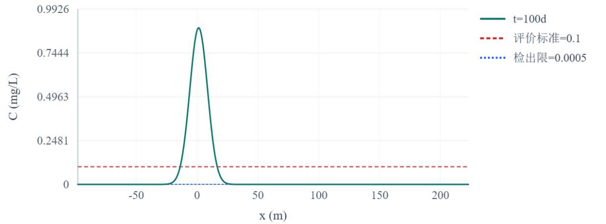
图 6.3-2 封孔槽-镍 t=100 d 地下水流向浓度变化趋势图
