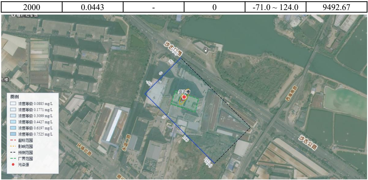
图 6.3-1 封孔槽-镍 t=100 d 浓度等值线图
