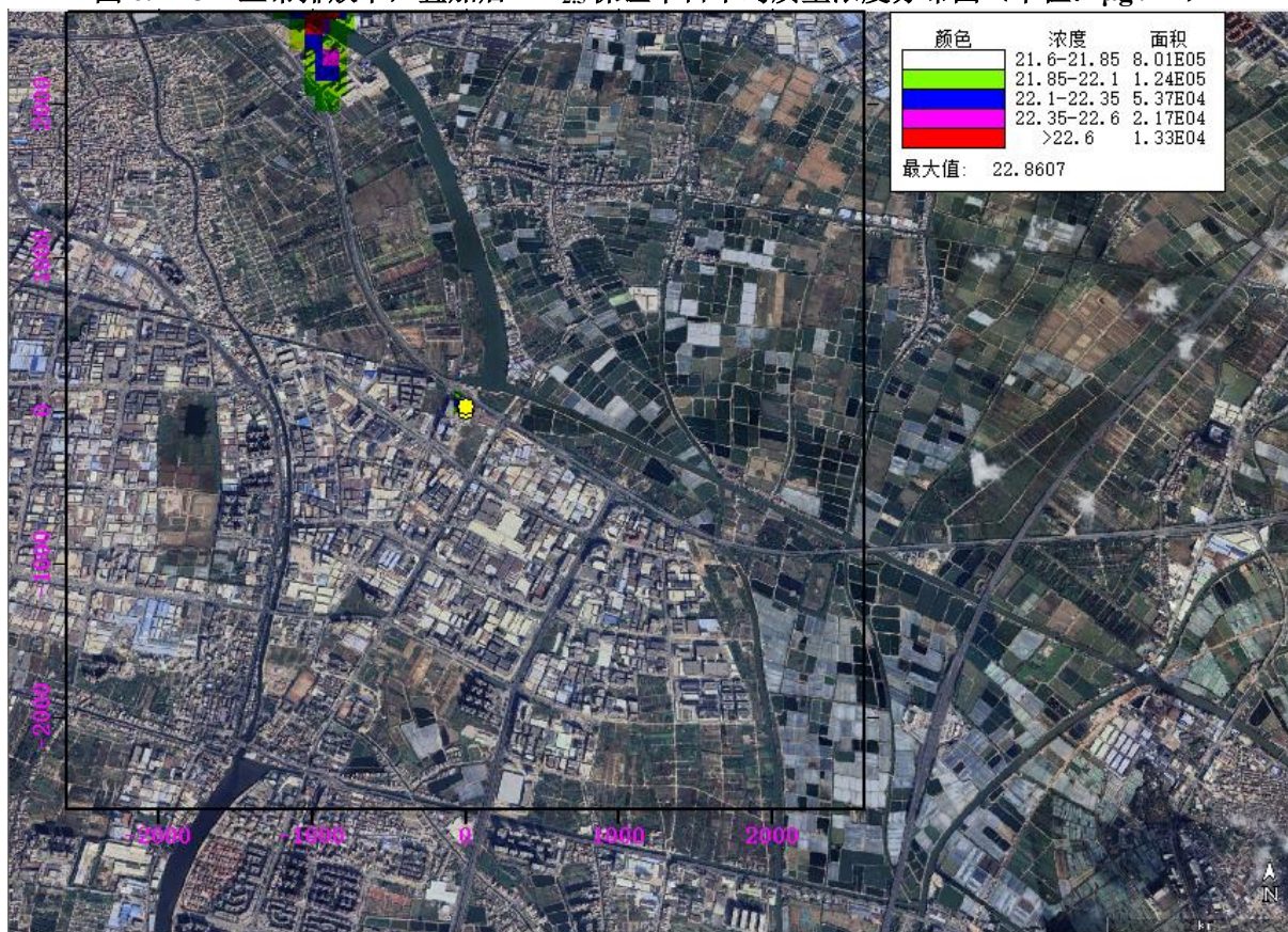
图 6.1-14 正常排放下，叠加后 PM_{2.5} 年平均质量浓度分布图（单位: \mu g/m^3 ）
