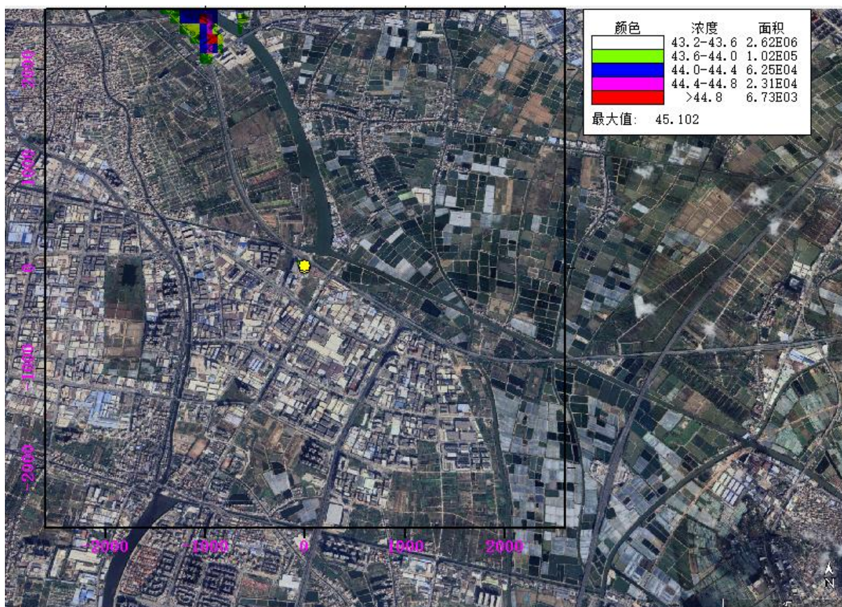
图 6.1-13 正常排放下，叠加后 PM_{2.5} 保证率日平均质量浓度分布图（单位: \mu g/m^3 ）
