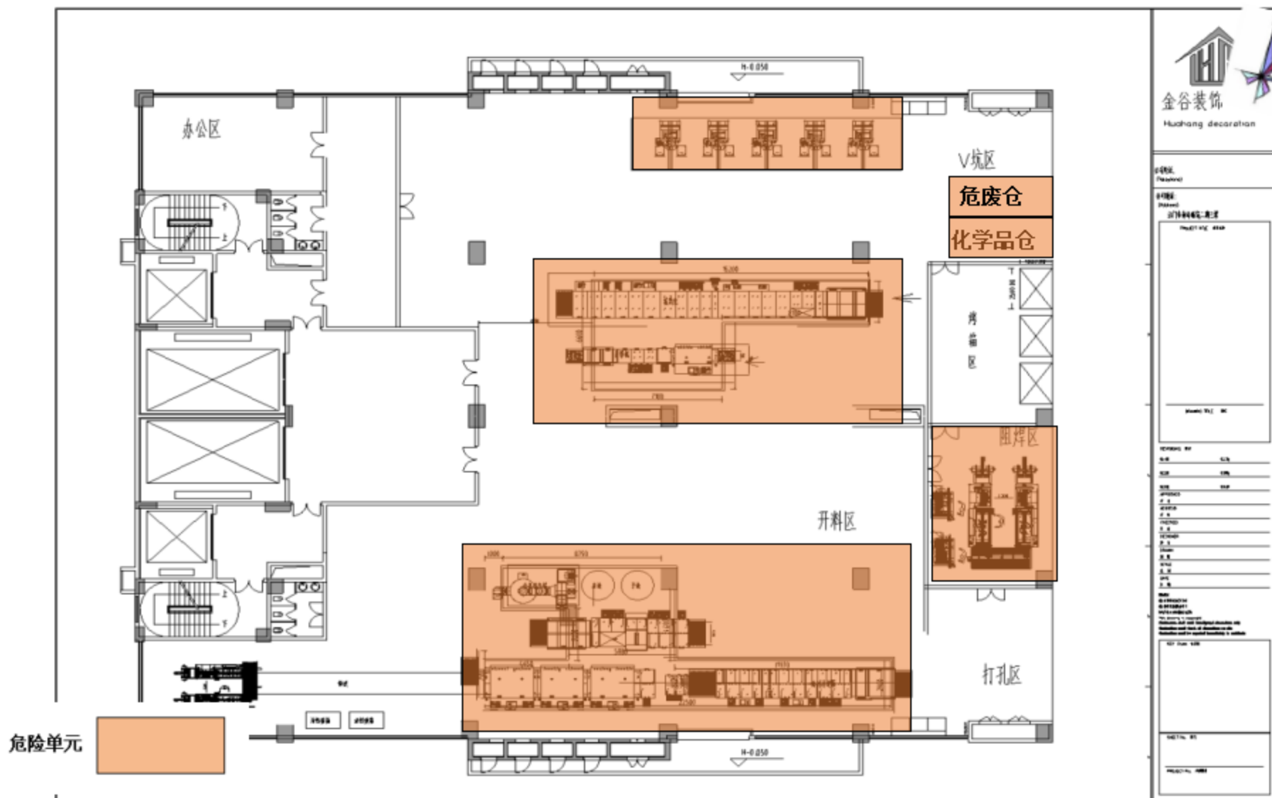
图 4.2-1 危险单元分布图 (5 楼生产车间)
