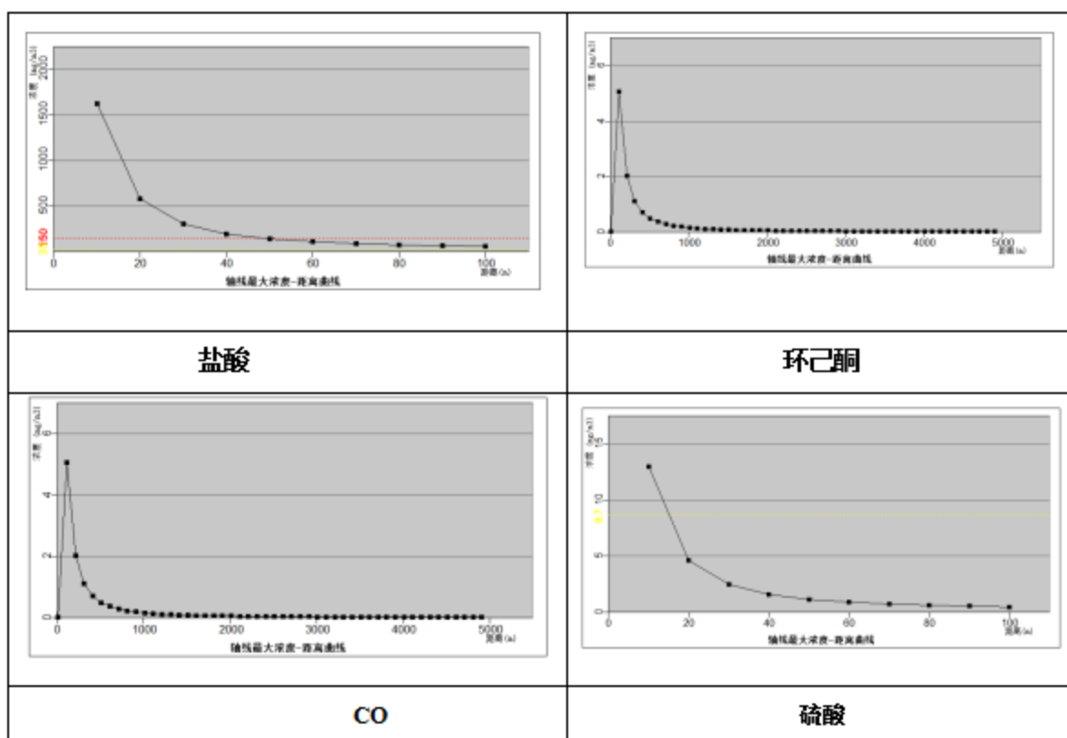
6.2-1 最不利气象条件下环己酮泄漏排放下风向轴线最大浓度-距离曲线图
