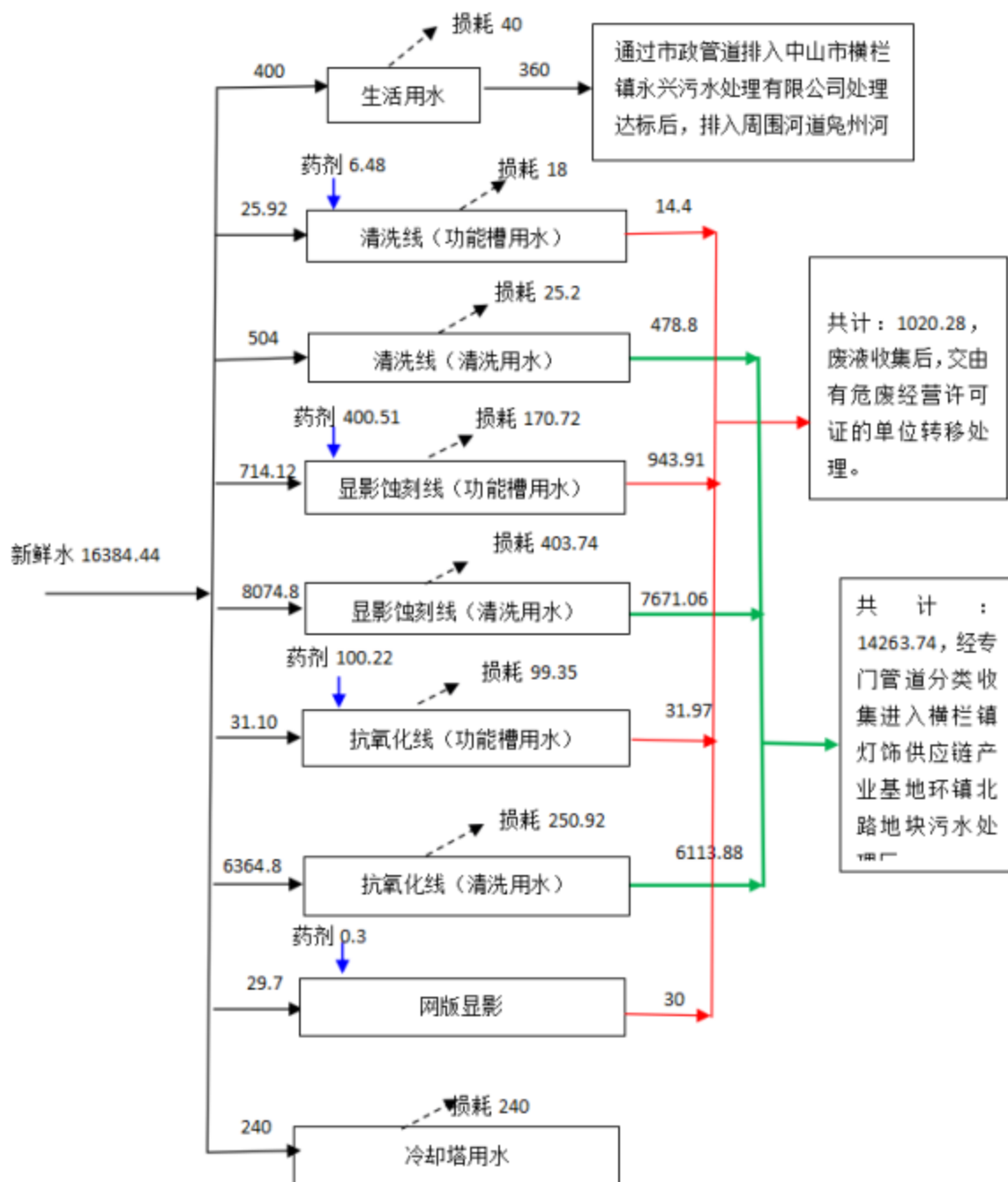
图 1 项目水平衡图 单位： m 3 /a
