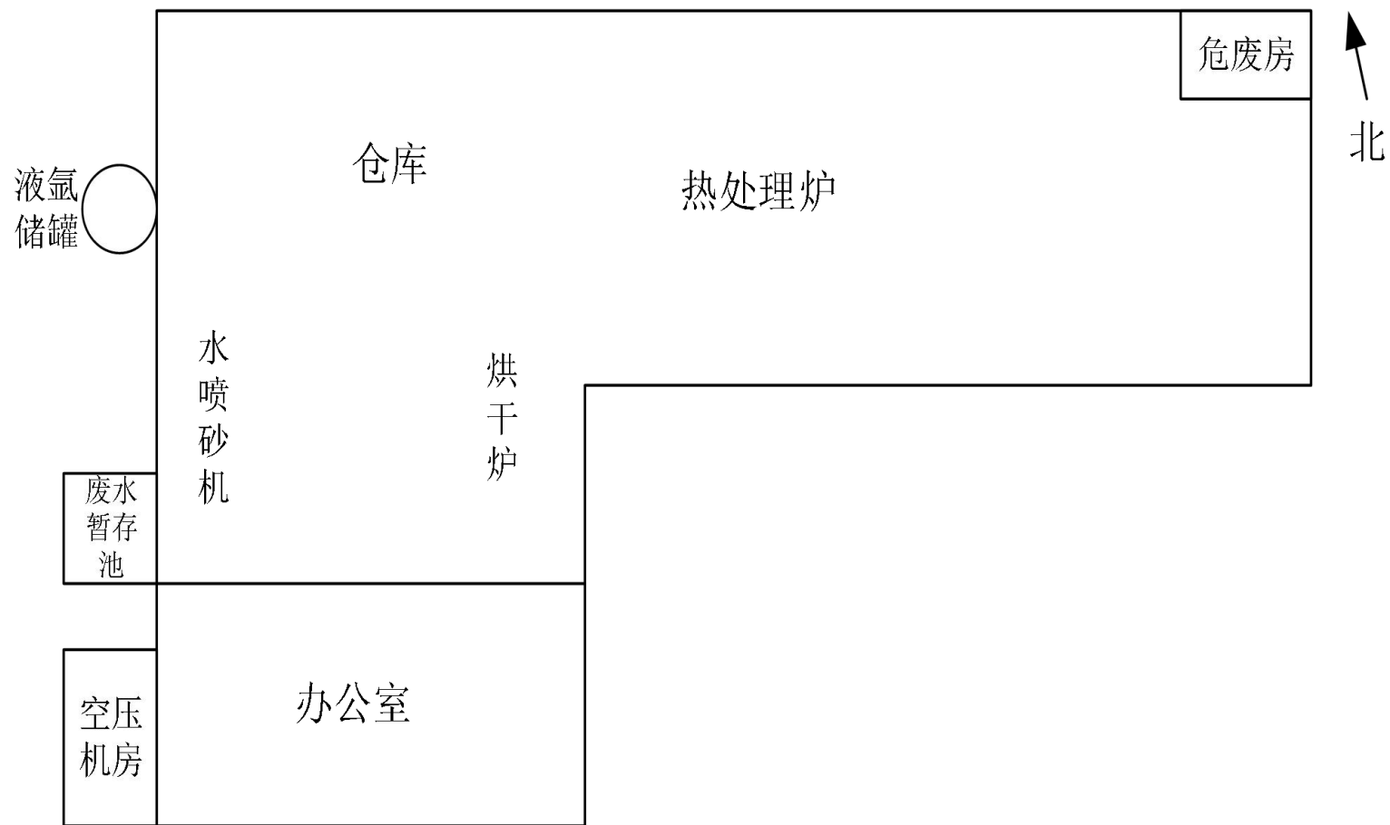
图一 建设项目平面布置图
