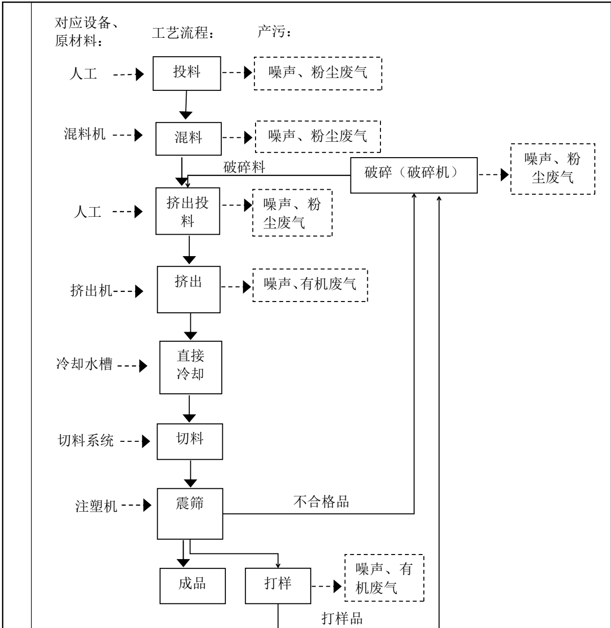
图2 项目生产工艺流程图
