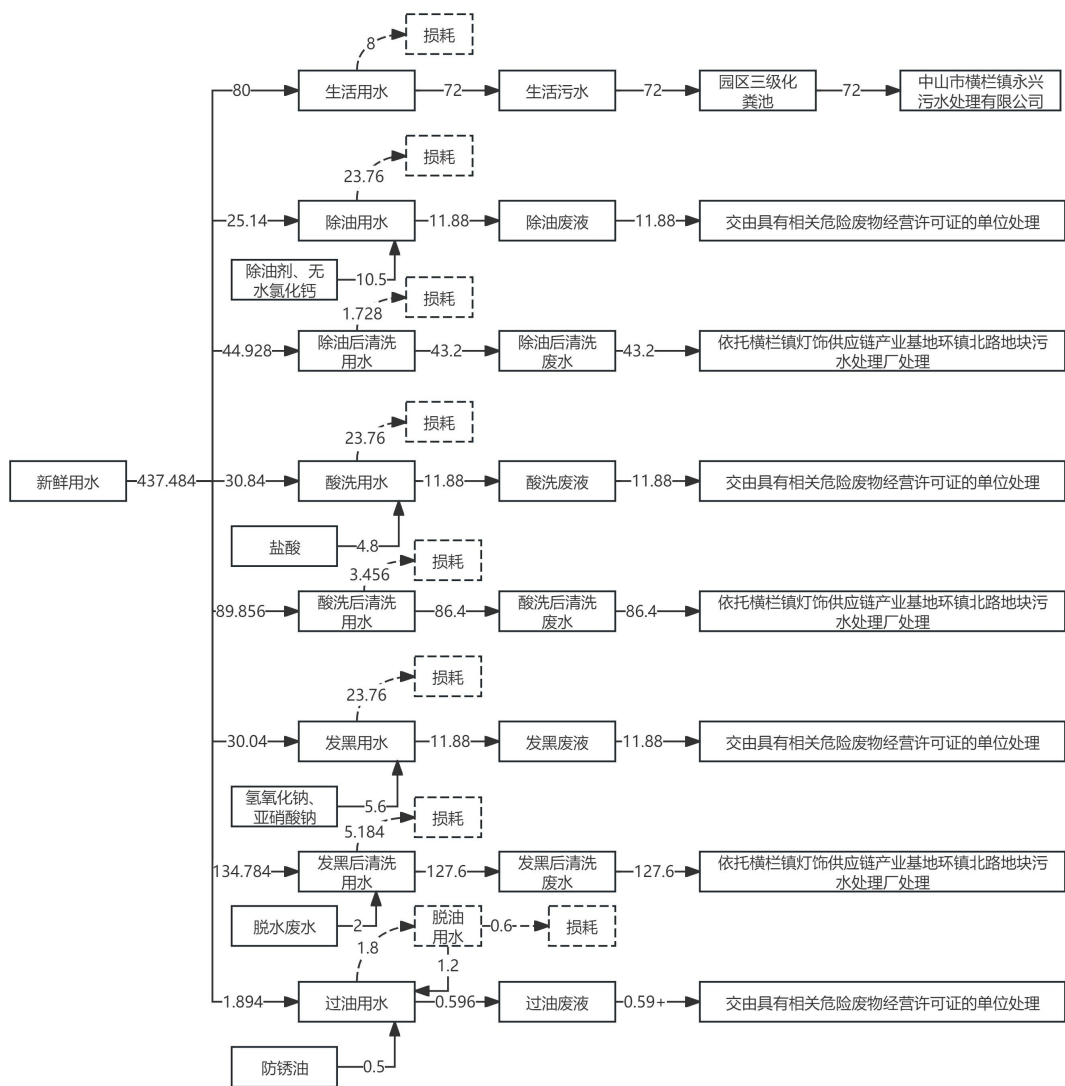
水平衡图 (m³/a)
