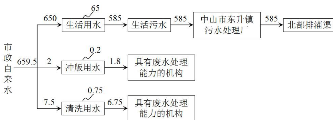
水平衡图 (t/a)
