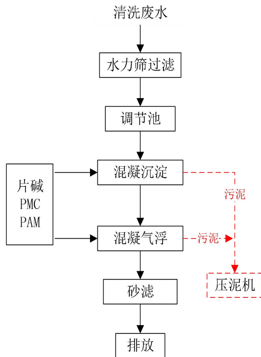
图 6 污水处理设施工艺流程
