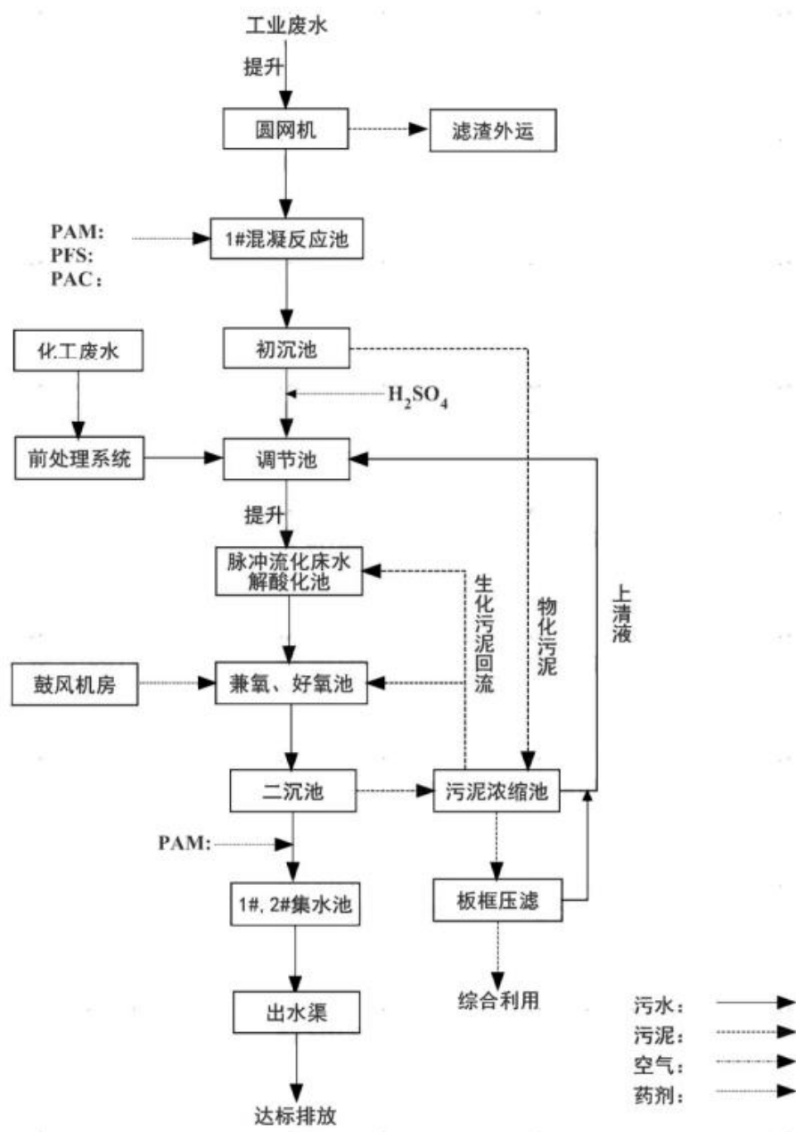
图 7 中山海滔环保科技有限公司废水治理工艺流程图
