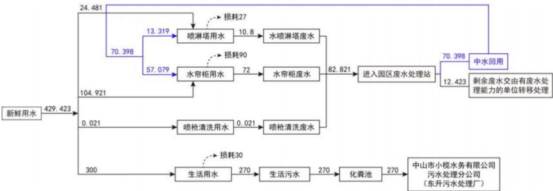
图 1 项目水平衡图（单位：t/a）
