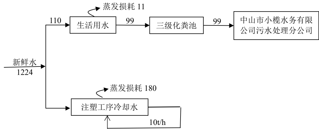
图 2-1 本项目水平衡图（单位：吨/年）
