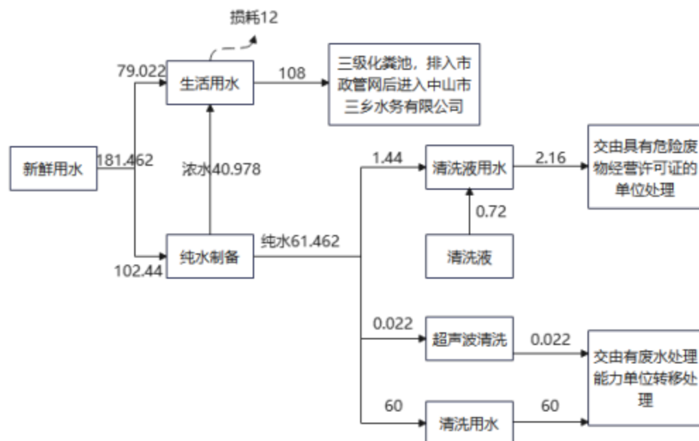
图一 项目水平衡图 单位：t/a
