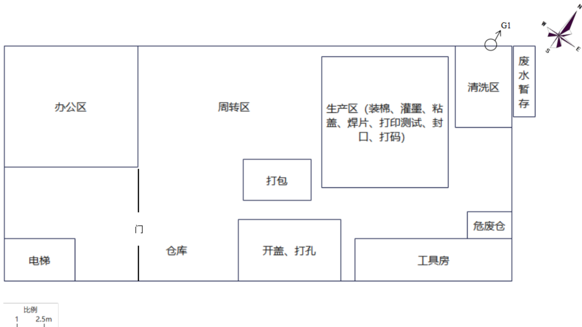
附图二 平面布置图
